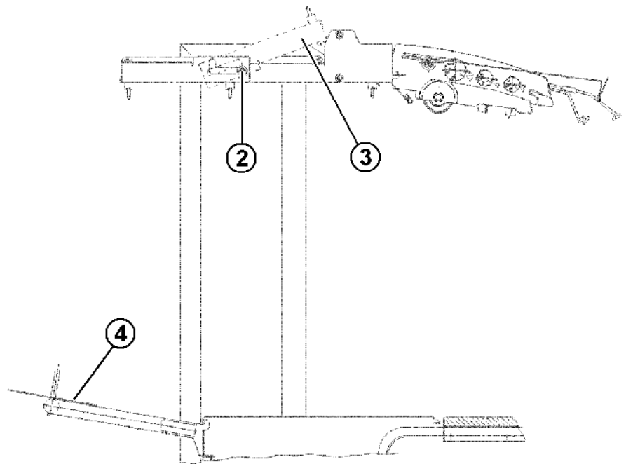
Fig. 4-16 Position der Träger für die Fadenkontrolleinrichtung
