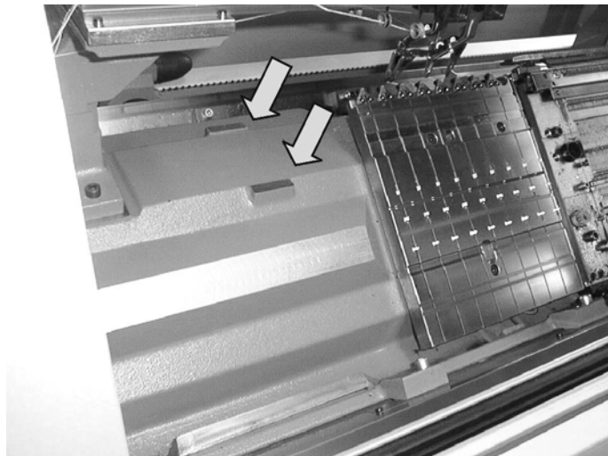
Fig. 4-14 Linke Auflagefläche für die Wasserwaage
