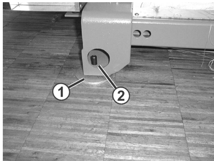
Fig. 4-1 Unterlegscheibe unter dem Strickmaschinenfuß
