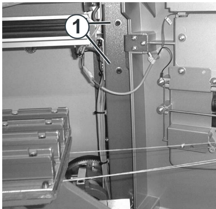
Fig. 4-15 Träger für die Fadenkontrolleinrichtung
