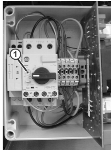
Fig. 4-8 Motorschutzscharter Q1
