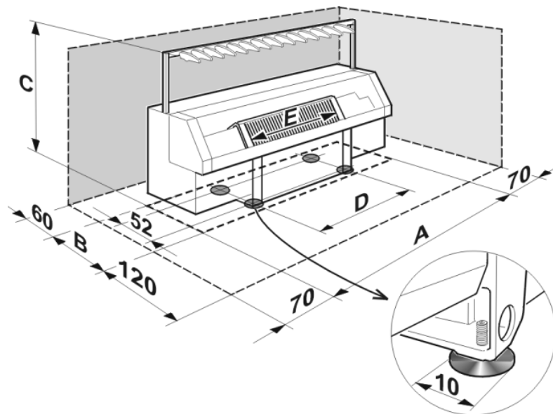
Fig. 2-1 Maße der Maschine (in cm)
