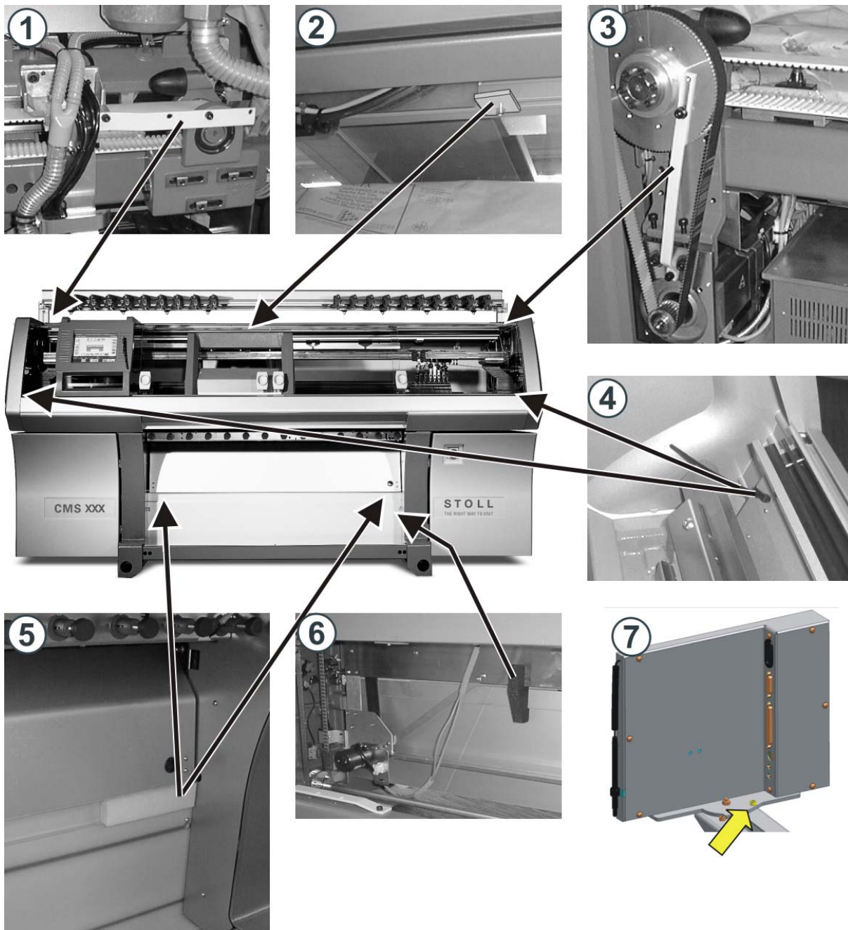
Fig. 4-3 Anbringungsorte der Transportsicherungen
