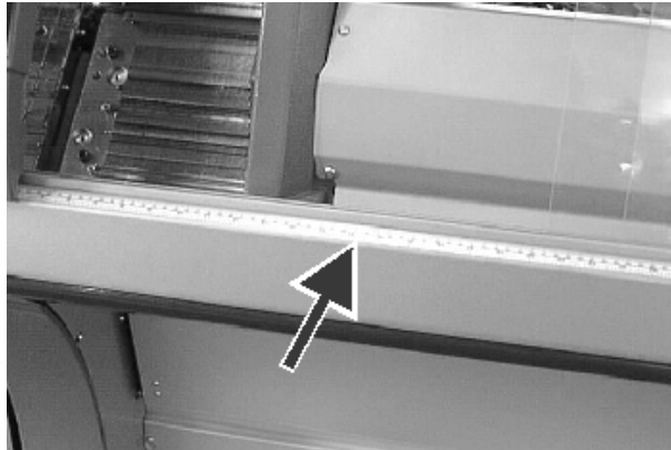
Fig. 4-18 Anbringen des Maßbandes
