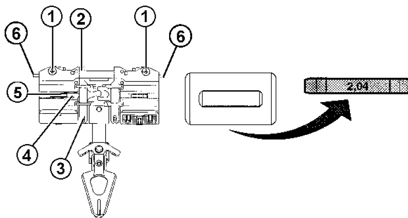
Fig. 4-71 卸下压板
