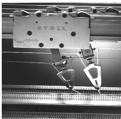
Fig. 2-10 嵌花导纱器
