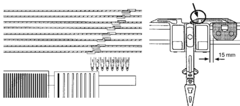
Fig. 4-65 调节导纱器限位器
