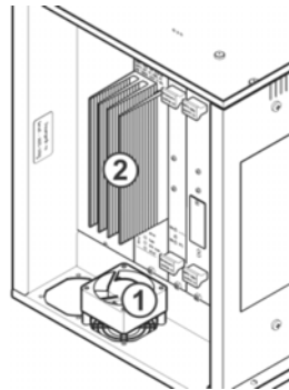
Fig. 5-13 控制单元
