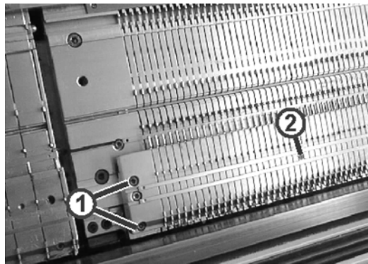
Fig. 6-29 松开选针片所在的针床
