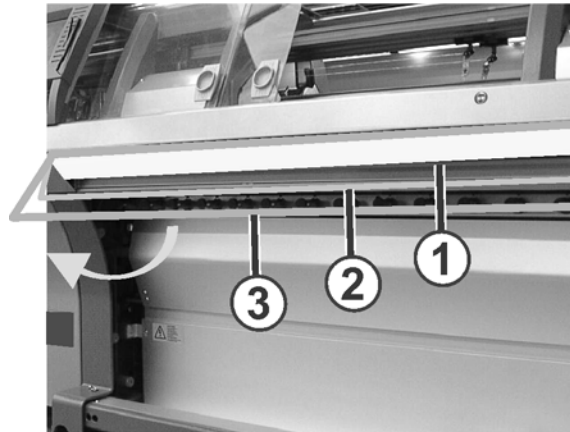
Fig. 3-18 操纵杆
