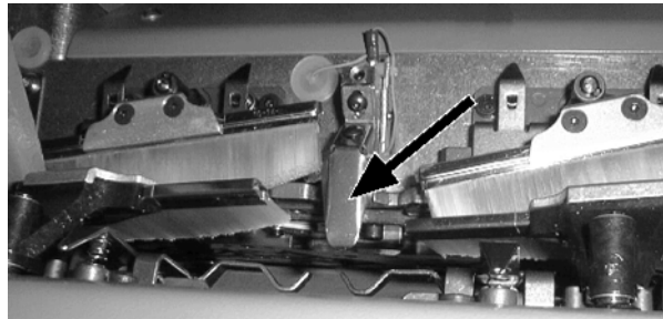
Fig. 6-40 织针探测器
