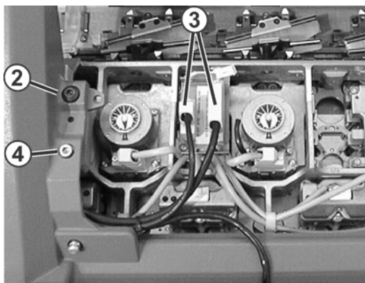
Fig. 6-38 打开的机头
