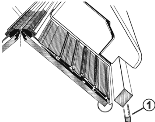
Fig. 5-26 润滑脉冲生成器导轨
