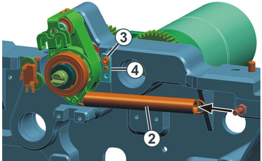
Fig. 6-65 牵拉辊的停位点
