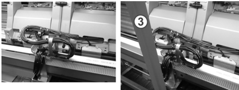
Fig. 4-60 将电缆放入线夹内
