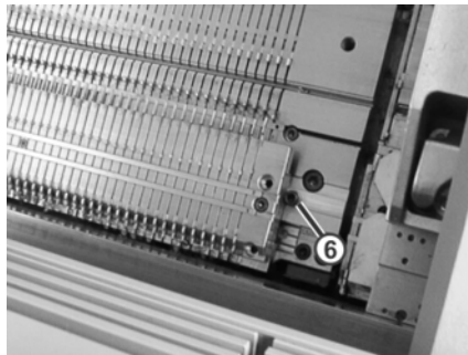
Fig. 6-31 安装选针片所在的针床
