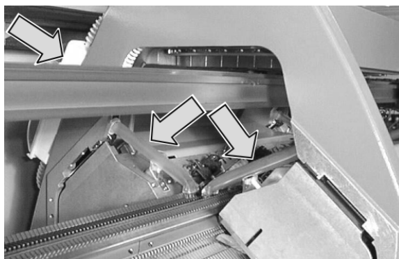
Fig. 2-13 吸尘装置和集尘盒(001系列或更高)
