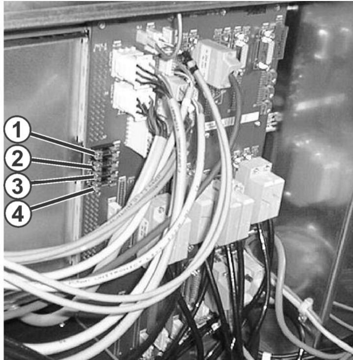
Fig. 6-73 左边控制单元后面的保险丝
