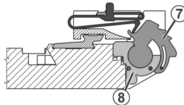
Fig. 6-15 将弹簧向前推
