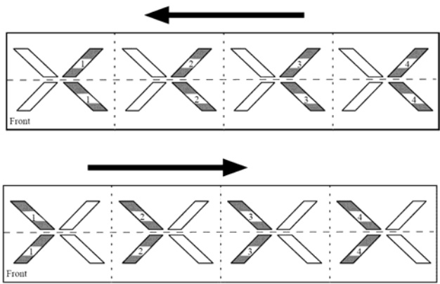
Fig. 4-46 四系统编织机成圈三角的编号
