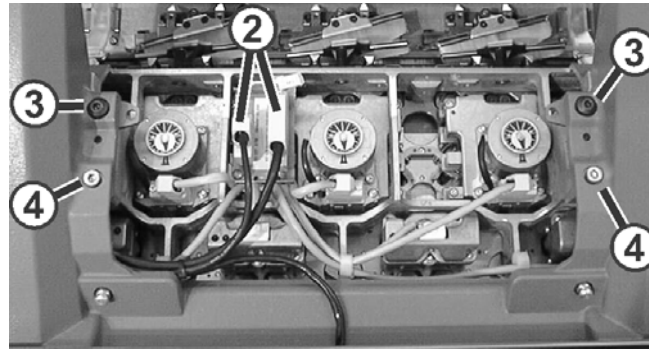
Fig. 6-44 将机头固定在三角座上
