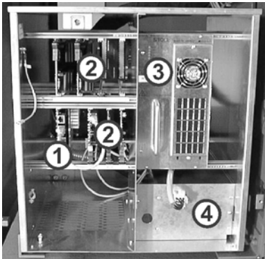
Fig. 6-69 左控制箱
