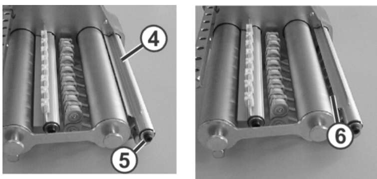
Fig. 4-10 设置自停板和摩擦辊之间的距离
