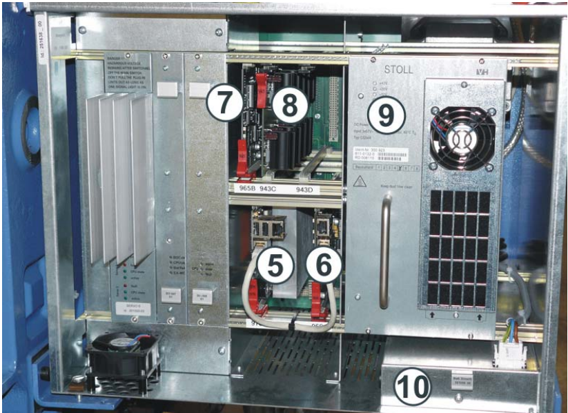
Fig. 6-68 右控制箱
