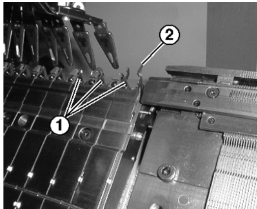
Fig. 2-9 切夹纱装置
