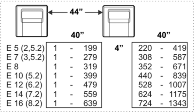
Fig. 4-52 44" 连接宽度的织针区域
