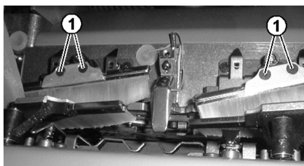
Fig. 4-62 毛刷螺丝
