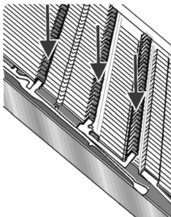
Fig. 5-27 挺针片针锤和中间片加润滑脂
