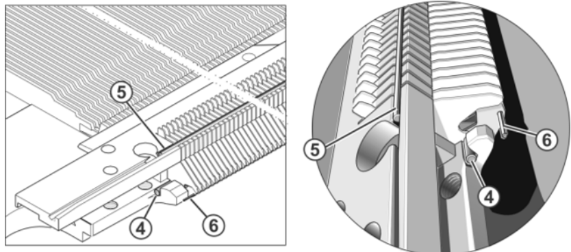
Fig. 6-11 更换沉降片
