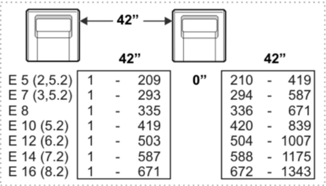
Fig. 10-6 42" 连接宽度的织针区域
