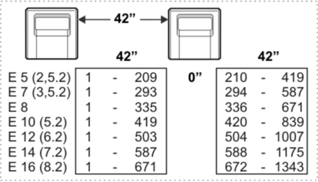
Fig. 10-2 42" 连接宽度的织针区域
