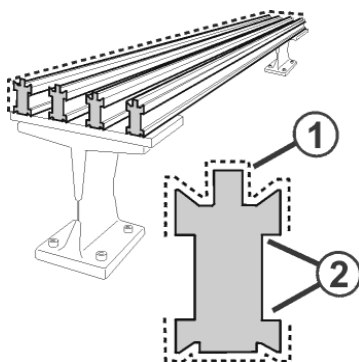
Fig. 5-29 导纱器杆加润滑脂
