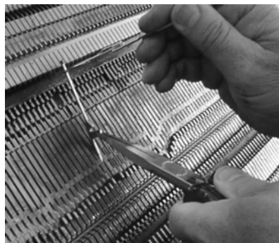
Fig. 6-6 移动挺针片部分
