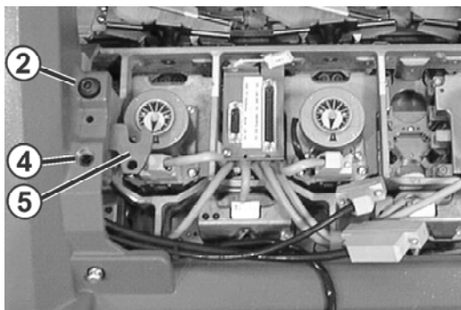
Fig. 6-37 摆动板
