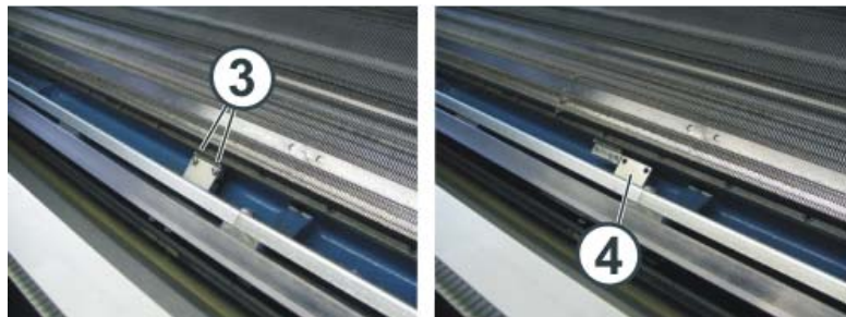
Fig. 6-19 连接脉冲发生器轨道
