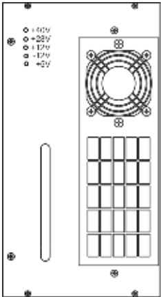
Fig. 6-71 电源装置
