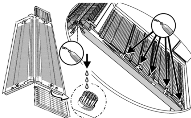
Fig. 5-21 针床加油
