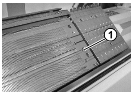
Fig. 2-15 清洁选针系统的毛刷
