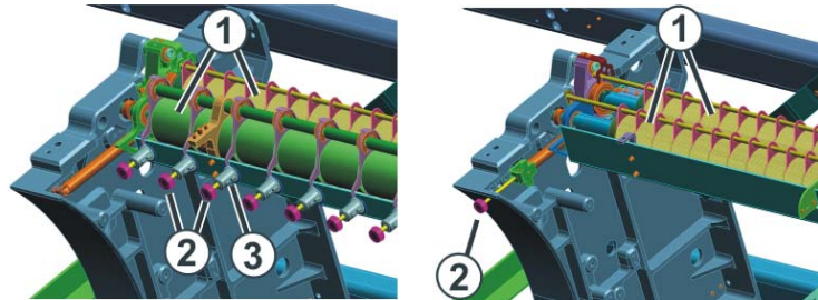
Fig. 2-27 主牵拉辊 (见右图: CMS 420 E)
