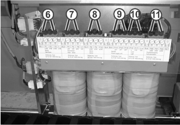
Fig. 6-76 机器后面变压器上的保险丝
