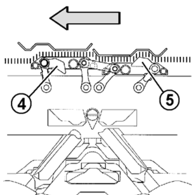
Fig. 2-21 沉降片滑片
