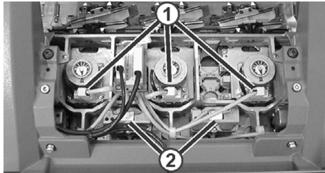
Fig. 6-45 选针系统插头
