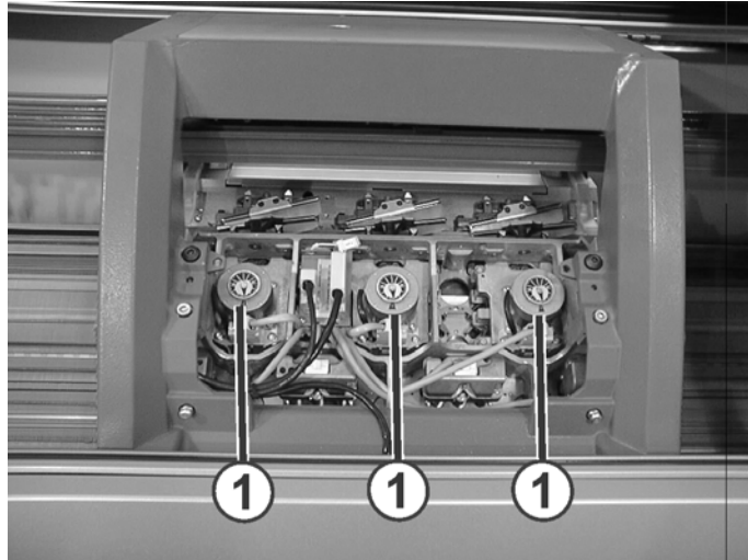
Fig. 2-22 调节线圈密度的步进马达
