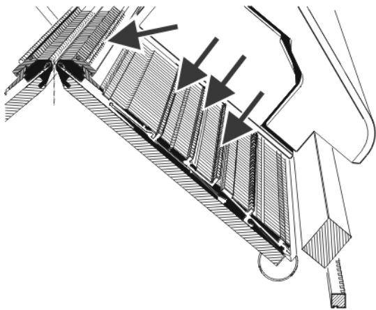
Fig. 5-18 中央润滑部分的润滑点
