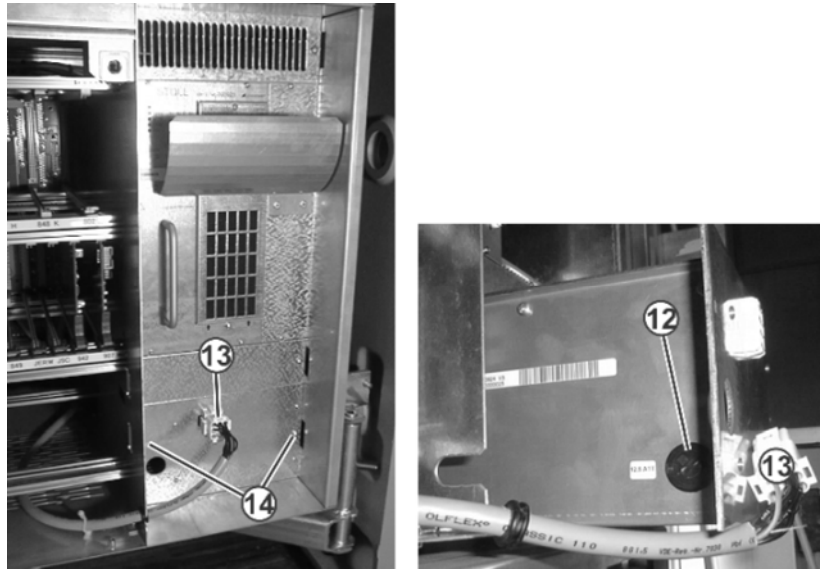
Fig. 6-74 电源装置下方的电池保险丝 (12)
