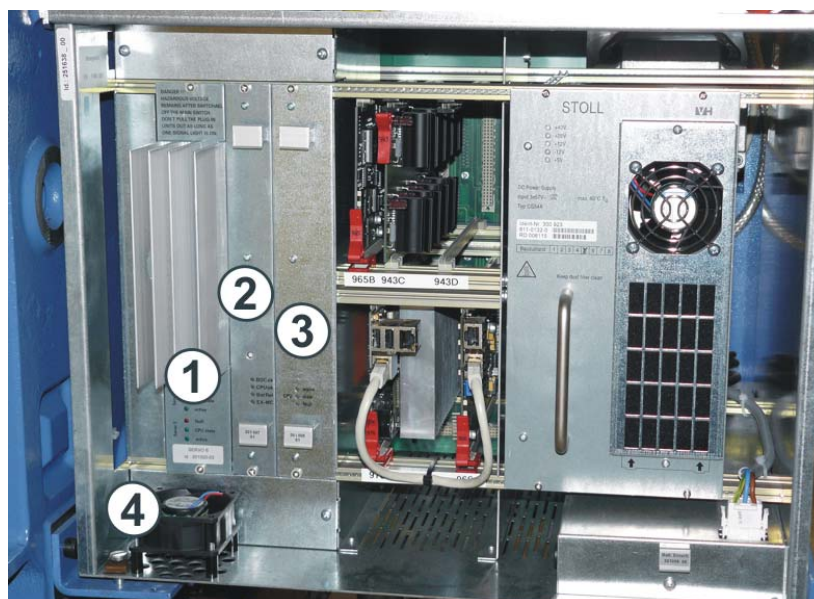
Fig. 6-67 右控制箱
