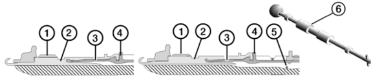
Fig. 6-5 更换织针和挺针片 (右图: CMS 520 C 和 CMS 830 C)
