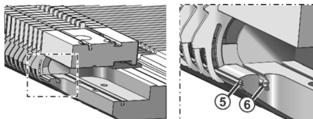
Fig. 6-16 拉出钢丝
