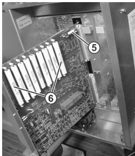
Fig. 6-75 右侧控制箱上的伺服传动及横移稳压保险丝 (5)
