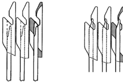
Fig. 2-30 牵拉梳钩和牵拉梳滑杆(左图: 打开, 右图: 关闭)
