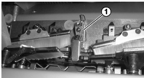
Fig. 2-24 织针探测器
