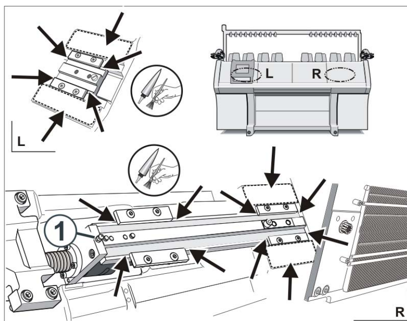
Fig. 5-31 横移装置加润滑脂
