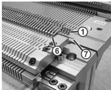
Fig. 6-32 抬起选针片
