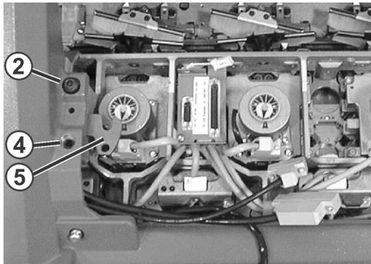
Fig. 6-41 摆动板
