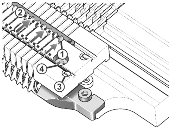
Fig. 6-12 将弹簧推入"打开位置"
