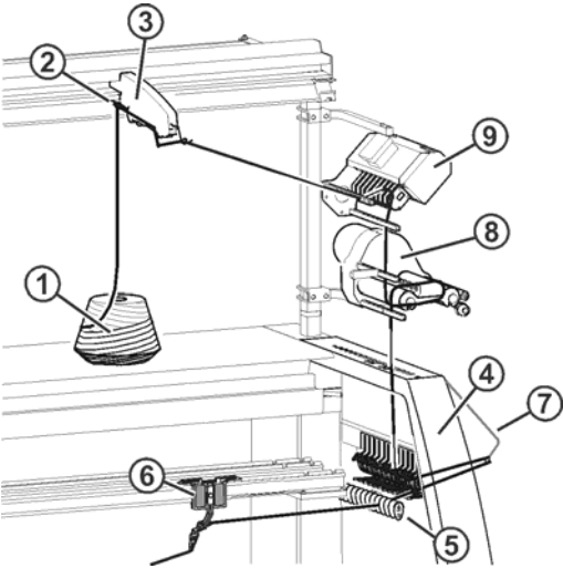
Fig. 2-4 穿纱方式4
