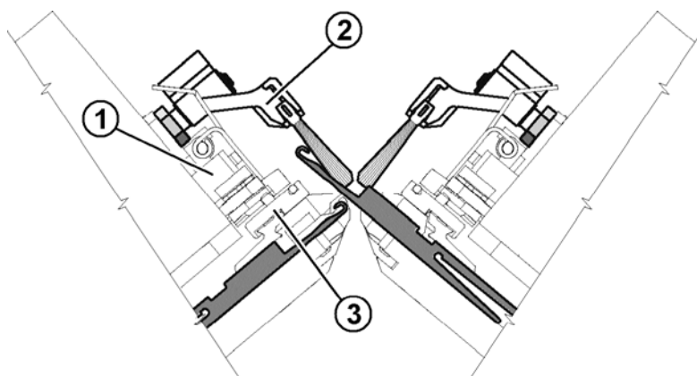
Fig. 2-20 沉降片控制装置
