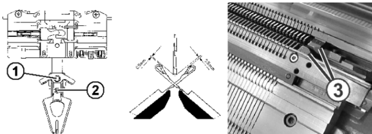
Fig. 4-69 调节嵌花导纱器
