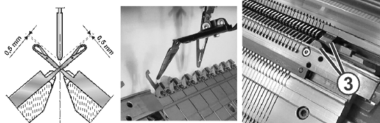
Fig. 4-63 调节导纱器
