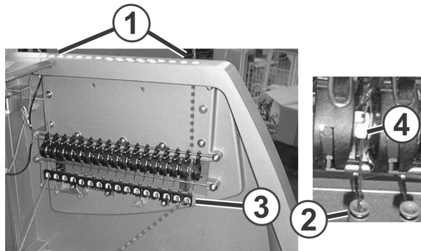
Fig. 3-14 从侧安全盖的穿纱路径
