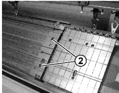
Fig. 6-18 松动针床
