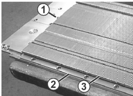
Fig. 6-28 修理组装型针床
