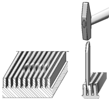
Fig. 6-25 竖直固定底座
