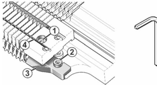
Fig. 6-14 卸下导纱器限位器 (3)
