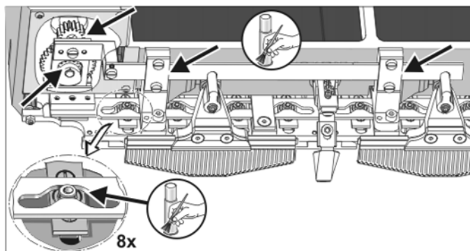
Fig. 5-30 给控制片加油
