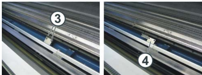
Fig. 6-22 连接脉冲发生器轨道
