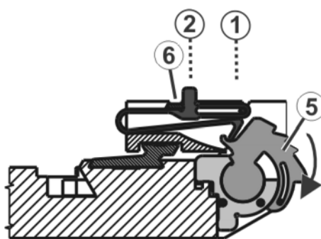
Fig. 6-13 更换弹簧
