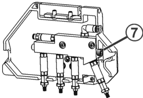
Fig. 6-63 排除中央润滑器的空气
