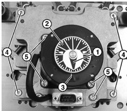
Fig. 6-48 卸下步进马达
