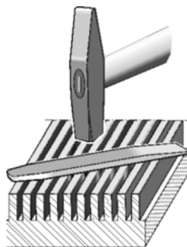
Fig. 6-26 校平表面
