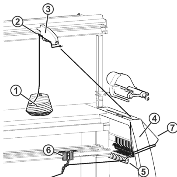
Fig. 2-2 穿纱方式2
