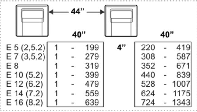
Fig. 10-3 44" 连接宽度的织针区域
