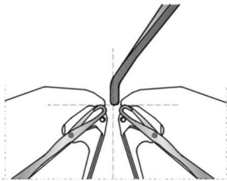
Fig. 4-61 调节织针探测器
