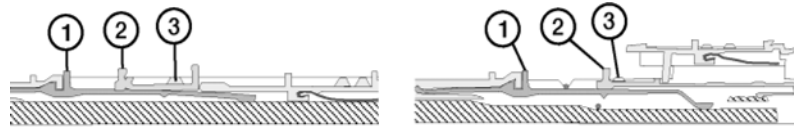
Fig. 6-8 更换中间片(右图: CMS 520 C 和 CMS 830 C)
