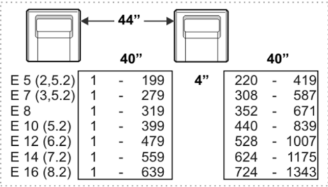
Fig. 10-7 44" 连接宽度的织针区域
