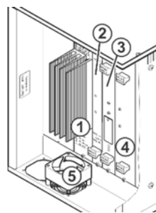
Fig. 6-70 右控制箱
