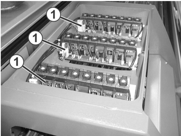
Fig. 6-72 电子卡用于控制导纱器
