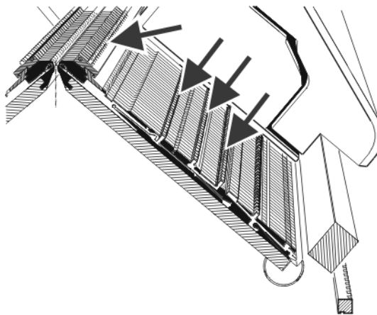
Fig. 2-17 中央润滑部分的润滑点
