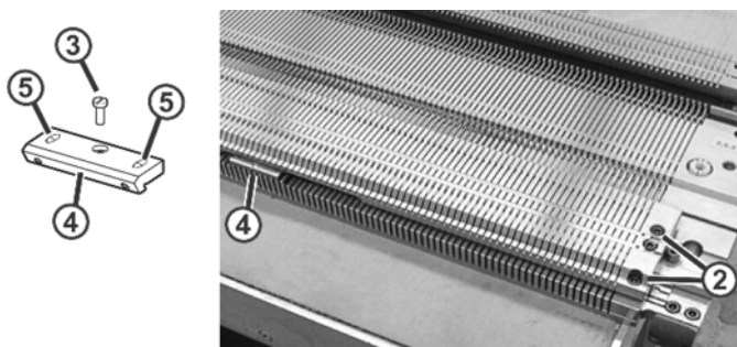
Fig. 6-33 松开选针片所在的针床
