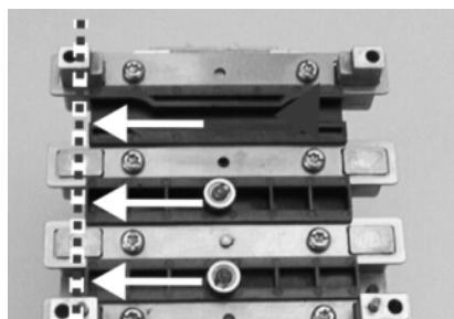
Fig. 6-52 安装位置监测
