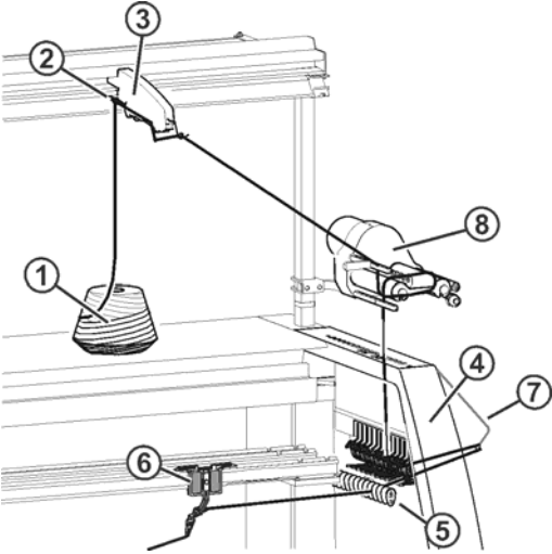
Fig. 2-3 穿纱方式3
