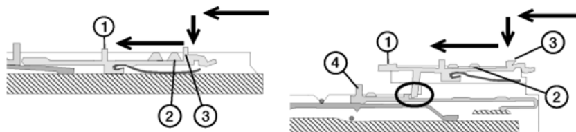
Fig. 6-9 更换选针片 (右图: CMS 520 C 和 CMS 830 C)
