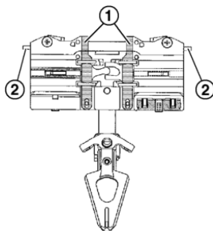
Fig. 6-56 嵌花导纱器
