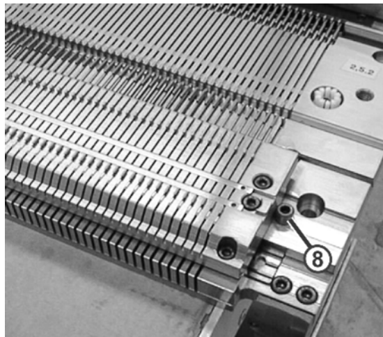
Fig. 6-34 安装选针片所在的针床
