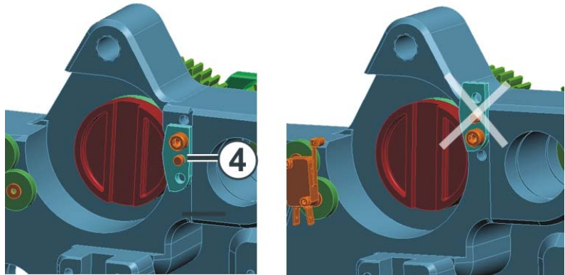
Fig. 6-66 旋转后的停位点
