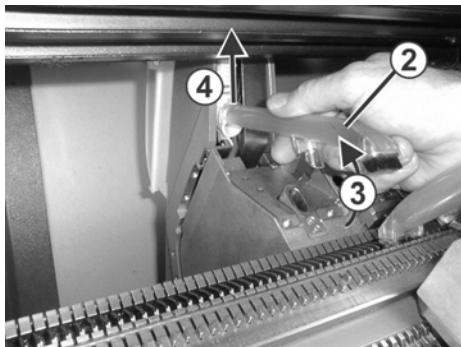
Fig. 5-3 吸管
