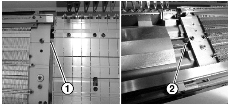
Fig. 6-23 安装前后针床
