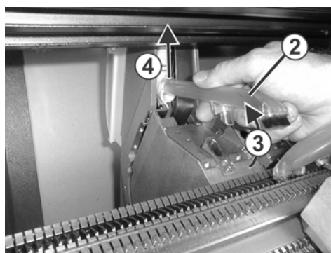
Fig. 5-3 Tubo di aspirazione
