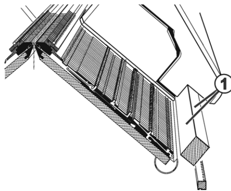
Fig. 5-25 Oliatura della barra di scorrimento del carro
