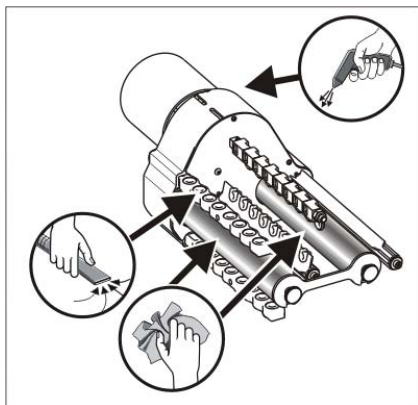
Fig. 5-11 Pulizia del fornitore a frizione
