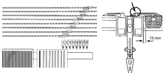
Fig. 4-65 Regolazione dei limitatori dei guidafili
