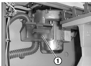
Fig. 5-4 Contenitore per la lanugine dell'aspirazione
