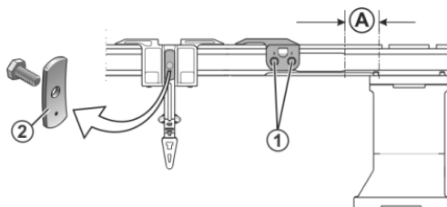
Fig. 6-53 Viti del limitatore dei guidafili
