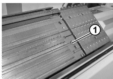
Fig. 2-15 Spazzolini per la pulizia dei sistemi di selezione
