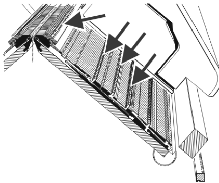
Fig. 2-17 Punti di lubrificazione della lubrificazione centrale
