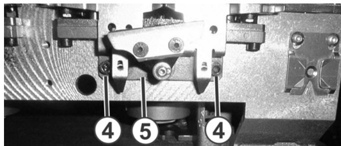
Fig. 6-47 Comando delle platine di abbattaggio
