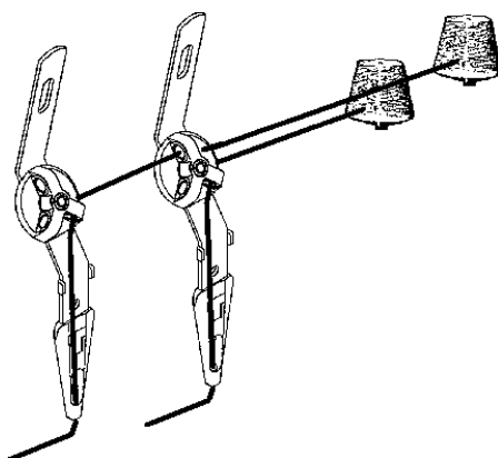
Fig. 3-15 Infilaggio in più guidafili di una guida
