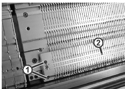
Fig. 6-29 Allentamento della frontura delle platine di selezione
