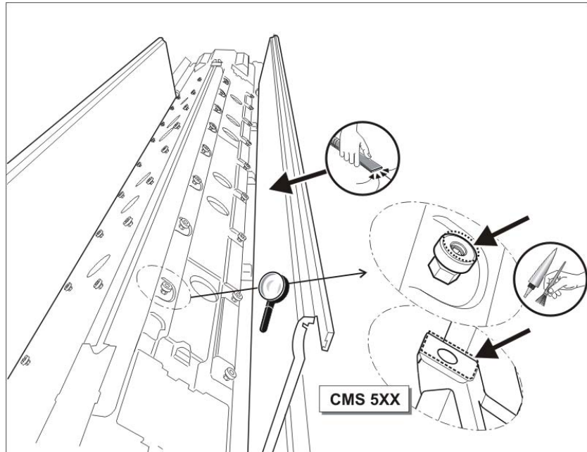
Fig. 5-32 Ingrassaggio degli appoggi della frontura
