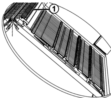
Fig. 5-23 Oliatura della frontura delle platine
