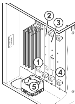
Fig. 6-70 Armadio di comando destro
