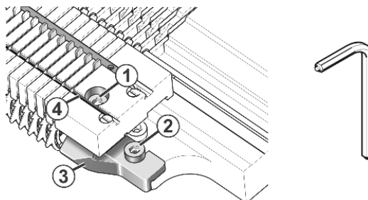
Fig. 6-14 Allontanamento del limitatore (3)
