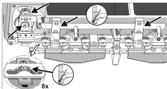
Fig. 5-30 Ingrassaggio della platina di comando
