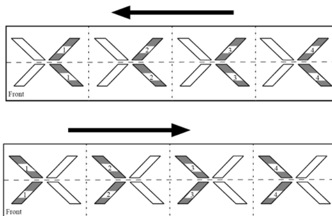
Fig. 4-46 Numerazione degli abbassa-agni per una macchina a 4 cadute
