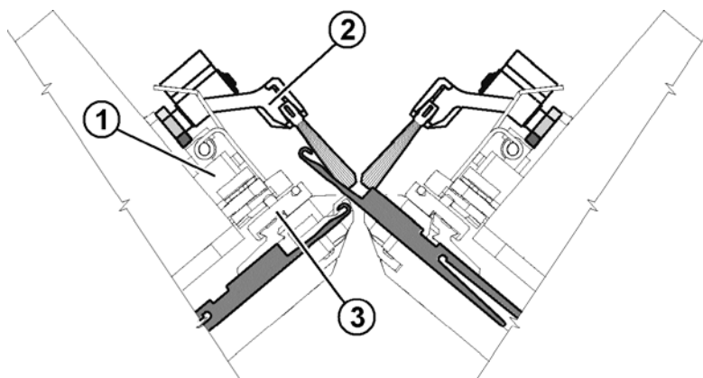
Fig. 2-20 Unità di comando delle platine
