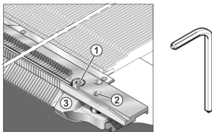
Fig. 6-10 Allontanamento del limitatore (3)
