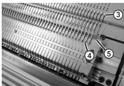
Fig. 6-30 Sollevamento delle platine di selezione
