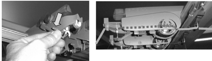
Fig. 3-12 Corso del filo nel dispositivo di controllo dei fili
