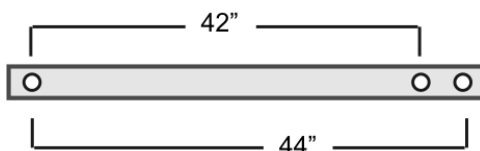
Fig. 4-49 Larghezze d'accoppiamento per la CMS 822
