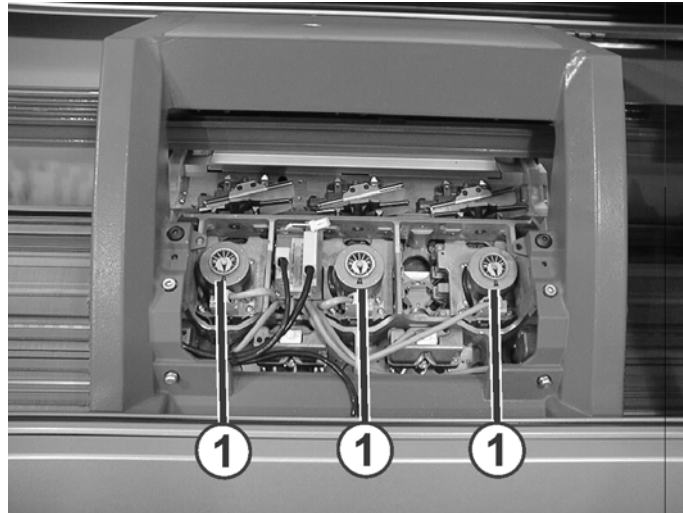
Fig. 2-22 Motorino passo a passo per la regolazione della fittezza della maglia Ogni sistema di lavorazione è dotato di un motorino passo a passo (1) che regola la fittezza della maglia. Il motorino passo a passo viene controllato dal programma di lavorazione.
