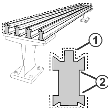
Fig. 5-29 Ingrassaggio delle barre dei guidafili
