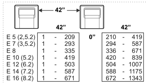
Fig. 10-2 Zona frontura per larghezza di accoppiamento 42"
