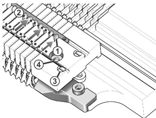
Fig. 6-12 Portare la molla in "Posizione aperta"
