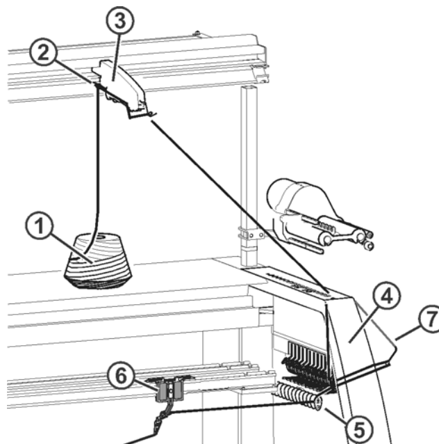
Fig. 2-2 Corsa 2
