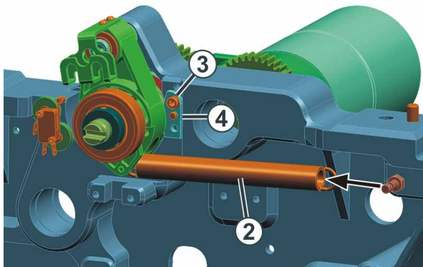
Fig. 6-65 Tacchetto del rullo di tiraggio
