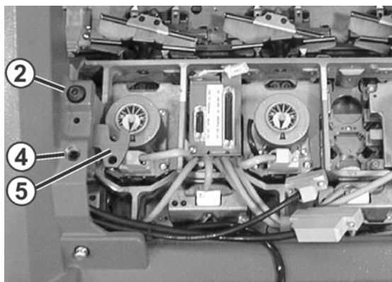
Fig. 6-41 Piastra girevole
