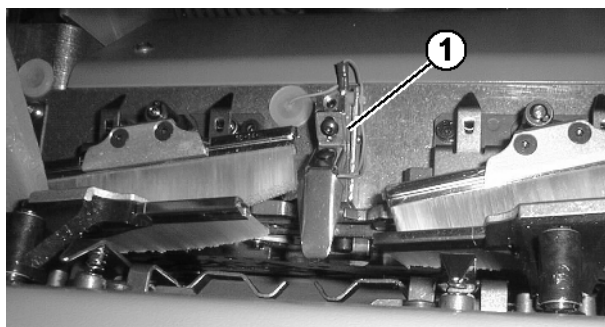
Fig. 2-24 Salva-aghi
