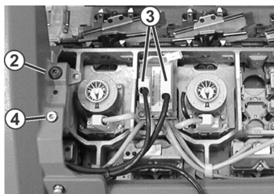
Fig. 6-38 Carro aperto
