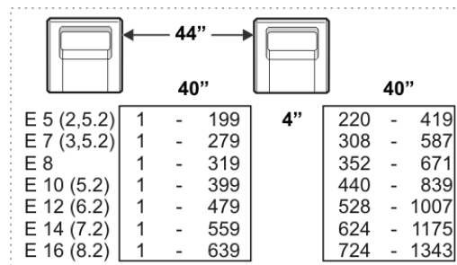
Fig. 10-7 Settore di aghi per larghezza di accoppiamento 44"
