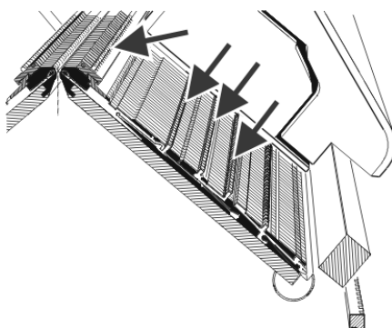
Fig. 5-18 Punti di lubrificazione della lubrificazione centrale
