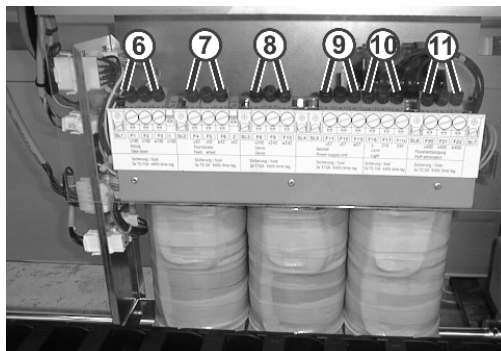
Fig. 6-76 Fusibili sul trasformatore sul lato posteriore della macchina
