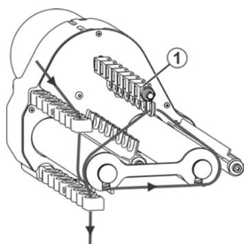
Fig. 4-8 Regolazione dell'alimentazione del filo sul fornitore a frizione
