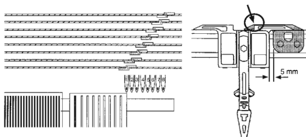
Fig. 4-64 Regolazione dei limitatori dei guidafili
