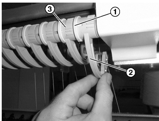
Fig. 4-9 Regolazione dell'alimentazione del filo sul fornitore a frizione
