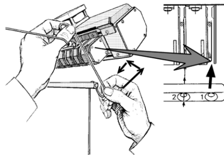
Fig. 3-13 Percorso del filo nell'apparecchio STIXX
