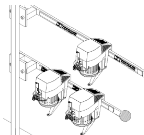
Fig. 2-7 Fornitore ad accumulo SFE
