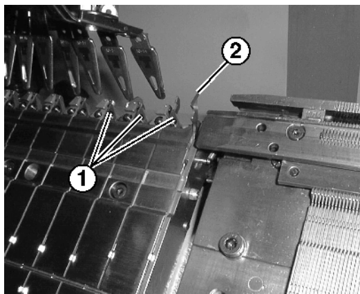
Fig. 2-9 Dispositivo di pinzatura e taglio
