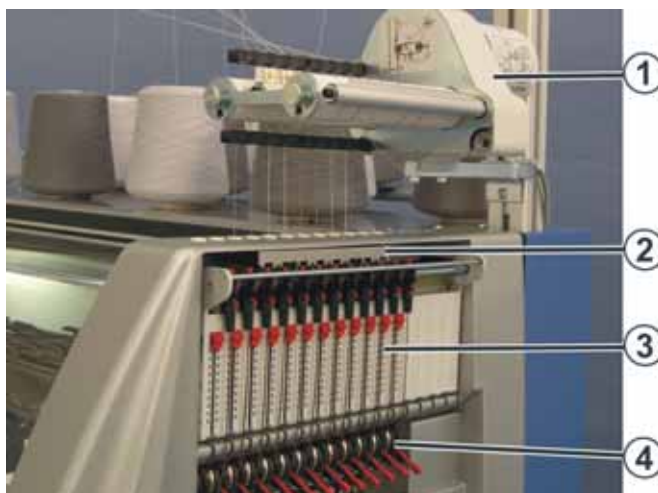
Fig. 2-6 Guida laterale del filo
