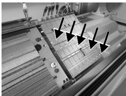
Fig. 5-22 Oliatura del dispositivo di pinzatura e taglio
