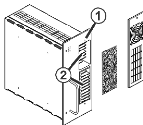
Fig. 5-14 Ventilatore dell'alimentatore
