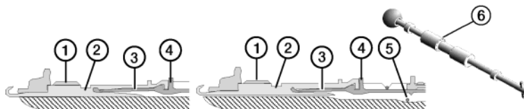
Fig. 6-5 Sostituzione dell'ago e del pezzo d'accoppiamento (figura destra: CMS 520 C e CMS 830 C)
