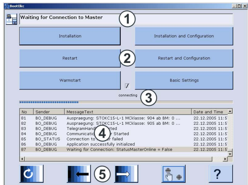
Fig. 7-3 Finestra "BootOkc"
