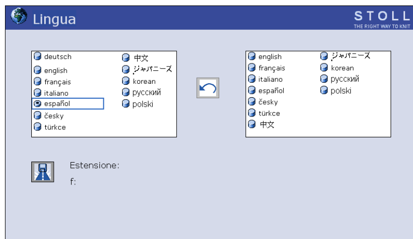
Fig. 4-37 Finestra "Lingua"
