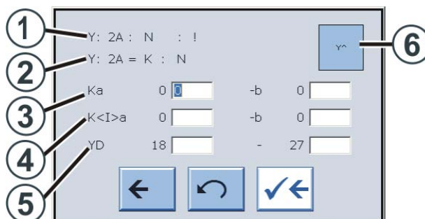
Fig. 4-30 Finestra "Guidafili"
