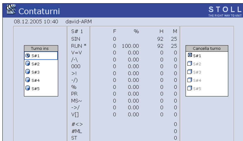
Fig. 3-20 Finestra "Contaturni"
