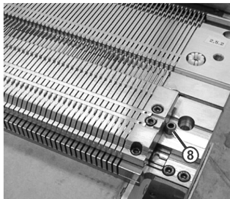
Fig. 6-34 Montaggio della frontura della platina di selezione
