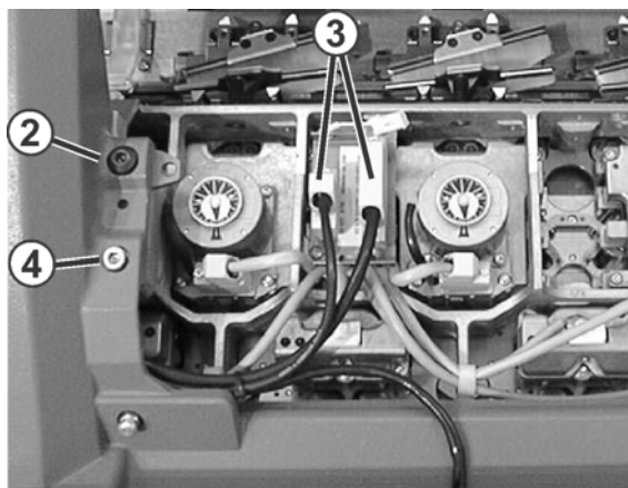
Fig. 6-42 Carro aperto
