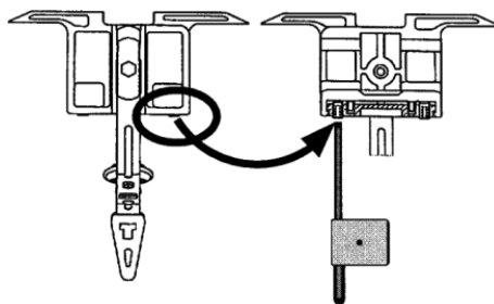
Fig. 4-66 Regolazione della guida del guidafilo
