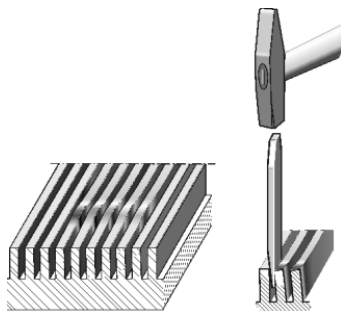
Fig. 6-25 Raddrizzamento delle platinette in posizione verticale
