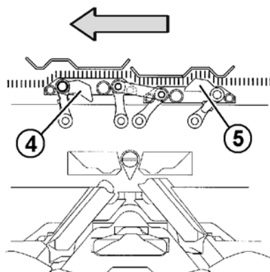
Fig. 2-21 Spingi-platine
