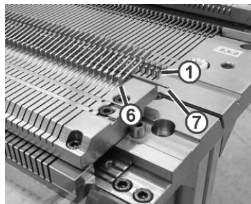
Fig. 6-32 Sollevamento delle platine di selezione
