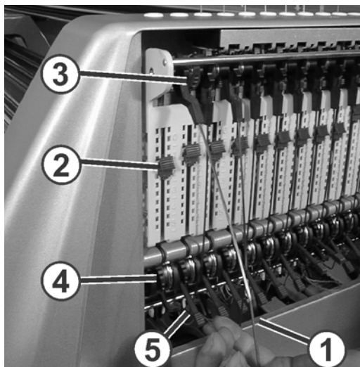
Fig. 4-7 Regolazione della tensione del filo
