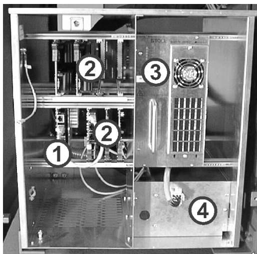
Fig. 6-69 Armadio di comando sinistro
