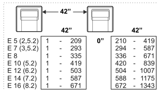
Fig. 10-6 Settore di aghi per larghezza di accoppiamento 42"
