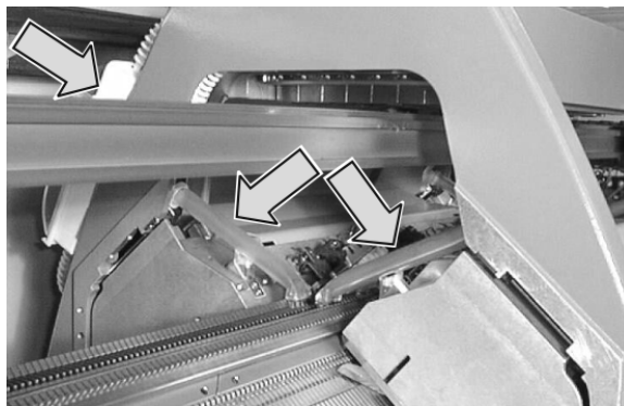
Fig. 2-13 Eliminazione della peluria e contenitore per la peluria (a partire dal modello 001)
