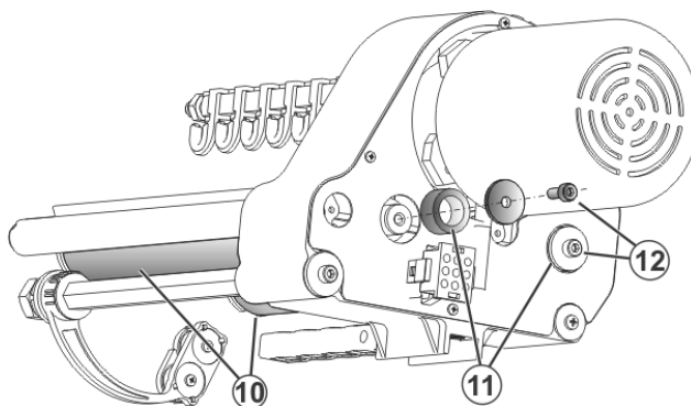
Fig. 6-61 Viti per i rulli a frizione
