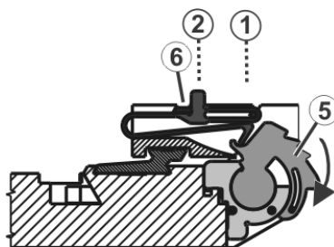
Fig. 6-13 Sostituzione della molla
