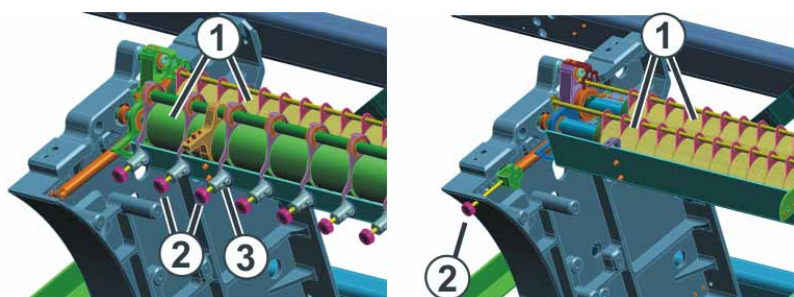
Fig. 2-27 Tiraggio principale (figura a destra: CMS 420 E)
