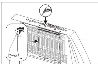
Fig. 5-9 Pulizia della pinza del filo attiva
