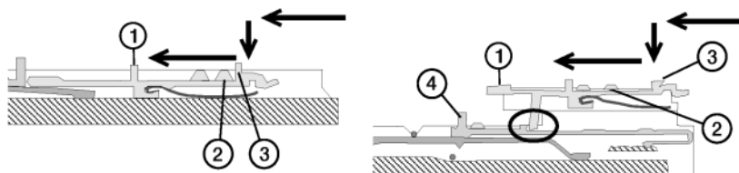
Fig. 6-9 Sostituzione della platina di selezione (figura a destra: CMS 520 C e CMS 830 C)
