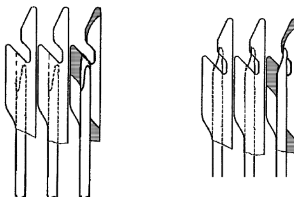
Fig. 2-30 Gancio del pettine di tiraggio con spingitoidi (aperto a sinistra, chiuso a destra)
