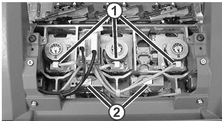
Fig. 6-45 Spine dei sistemi di selezione
