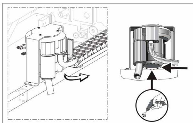
Fig. 5-2 Pulizia del coperchio del motore
