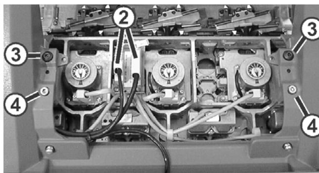
Fig. 6-44 Fissaggio del carro alla slitta
