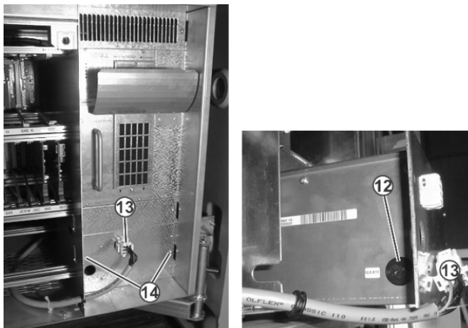
Fig. 6-74 Fusibile della batteria (12) sotto l'alimentatore
