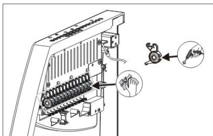
Fig. 5-10 Pulizia del freno permanente
