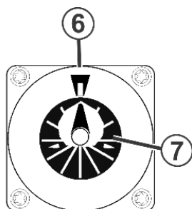
Fig. 6-49 Posizione di base del motorino passo a passo
