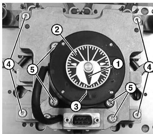
Fig. 6-48 Asportazione del motorino passo a passo
