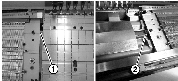
Fig. 6-23 Montaggio della frontura anteriore e posteriore
