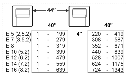
Fig. 4-52 Zona di aghi per larghezza di accoppiamento 44"
