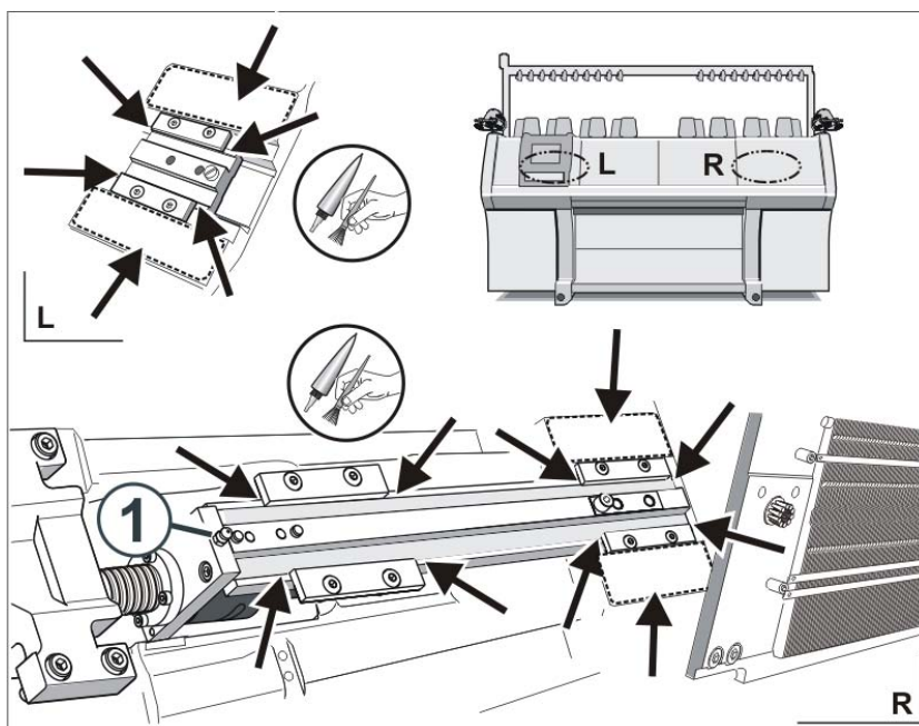
Fig. 5-31 Ingrassaggio del dispositivo di spostamento
