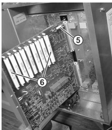
Fig. 6-75 Fusibile zavorra (5) per servoazionamento e spostamento sull'apparecchio di comando a destra
