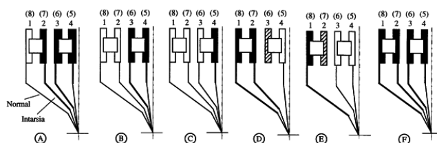
Fig. 6-54 Possibilità di combinazione per guidafile normali e per intarsio
