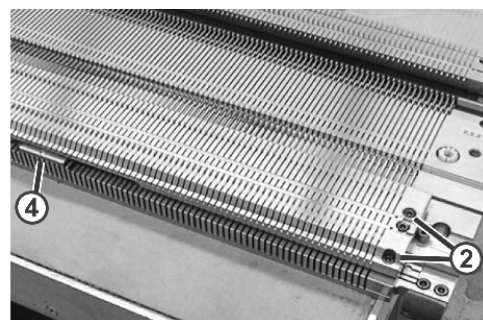
Fig. 6-33 Allentamento della frontura delle platine di selezione
