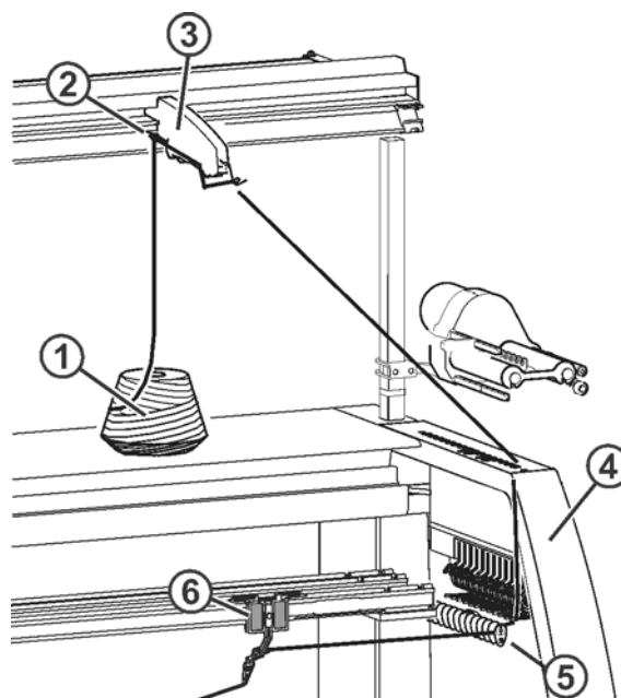
Fig. 2-1 Corsa 1
