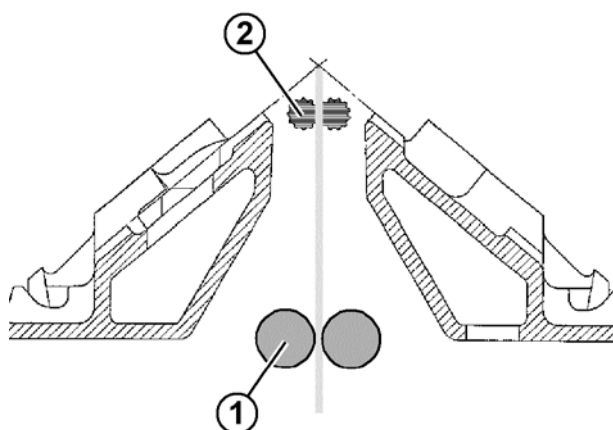
Fig. 2-28 Tiraggio ausiliario
