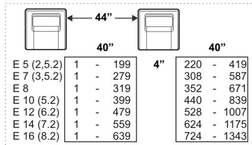
Fig. 10-3 Zona frontura per larghezza di accoppiamento 44"
