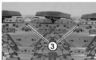
Fig. 6-46 Viti del corpo in ghisa sulla piastra carro
