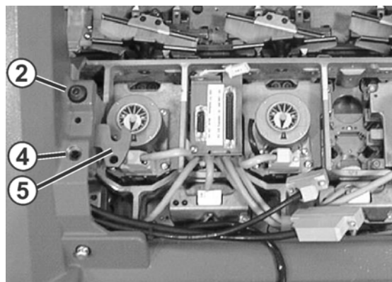
Fig. 6-37 Piastra girevole sinistra
