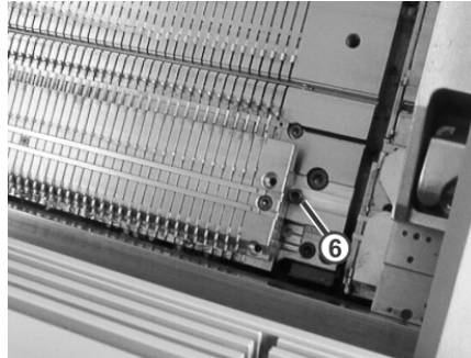
Fig. 6-31 Montaggio della frontura della platina di selezione
