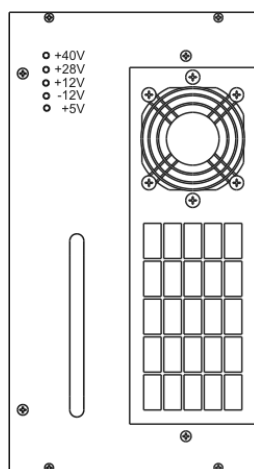
Fig. 6-71 Alimentatore
