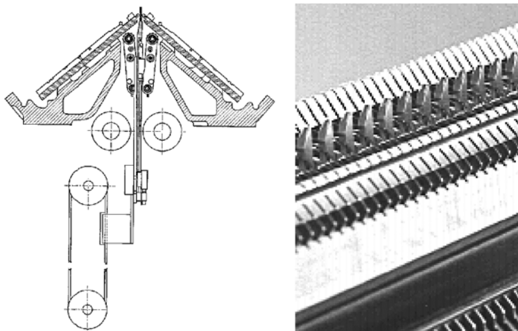
Fig. 2-29 Pettine di tiraggio
