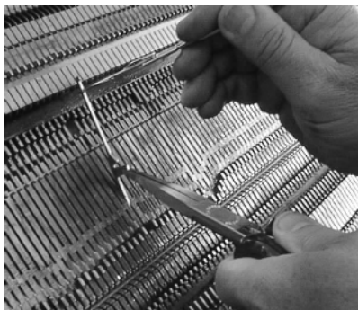
Fig. 6-6 Levare un pezzo d'accoppiamento fuori
