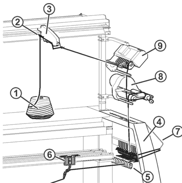
Fig. 2-4 Corsa 4
