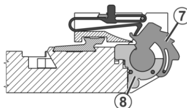
Fig. 6-15 Spostamento in avanti delle molle
