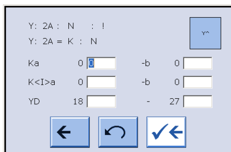
Fig. 4-27 Finestra "Guidafili"
