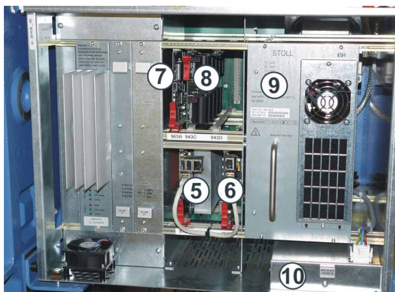
Fig. 6-68 Armadio di comando destro
