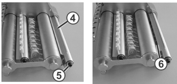
Fig. 4-10 Regolazione della distanza fra la barra di arresto ed il rullo a frizione
