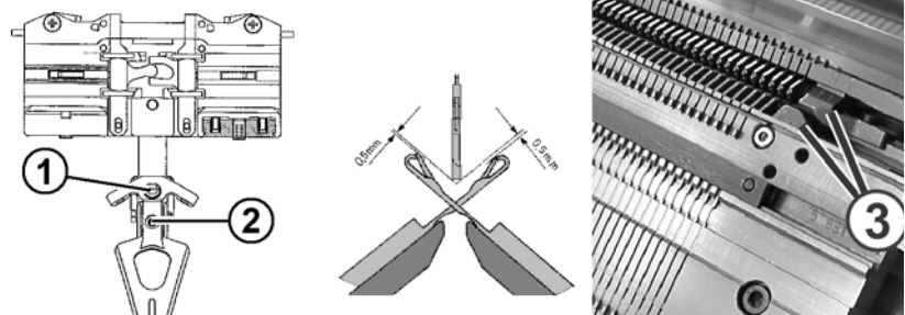
Fig. 4-69 Regolazione dei guidafili per intarsio
