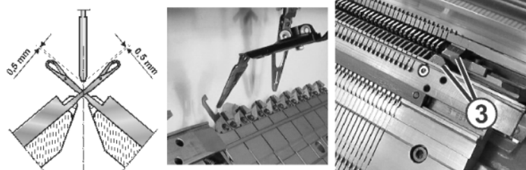
Fig. 4-63 Regolazione dei guidafile
