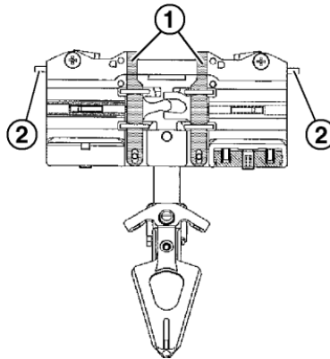
Fig. 6-56 Guidafili per intarsio
