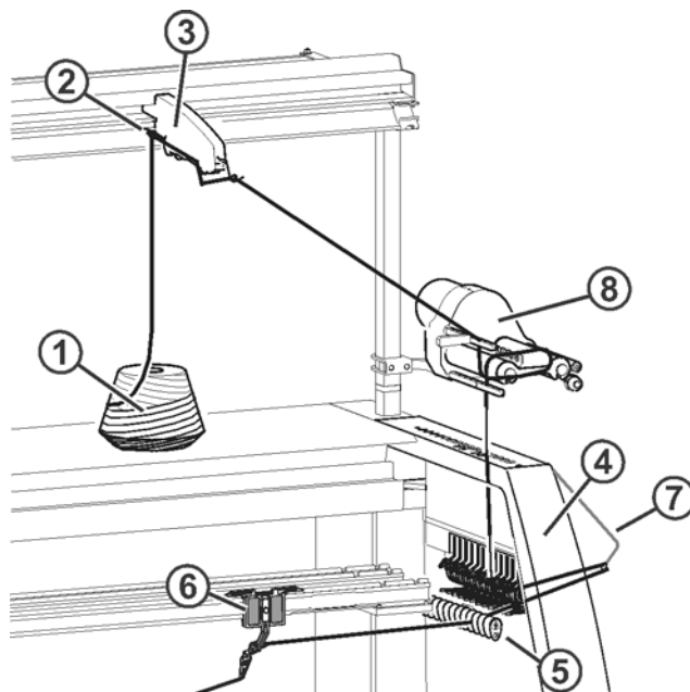
Fig. 2-3 Corsa 3
