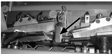
Fig. 6-40 Salva-ago
