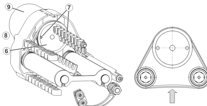
Fig. 6-60 Cinghia di comando
