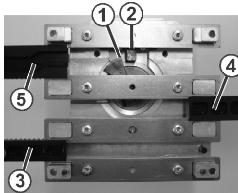
Fig. 6-51 Posizione di montaggio
