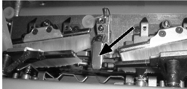
Fig. 6-28 Nadelwächter
