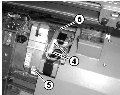
Fig. 6-50 Kabel und Schrauben der Fadenklemm- und Schneideinrichtung
