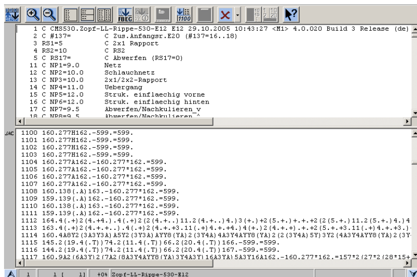
Fig. 4-98 Fenster bei der Funktion "Fenster teilen horizontal"
