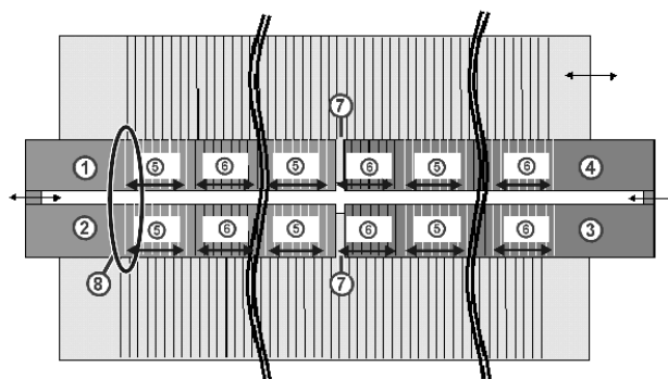
Fig. 4-48 Grundstellung der Nadelbetten zu den Zusatzbetten
