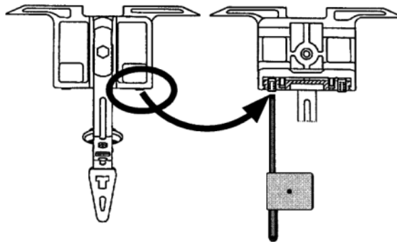
Fig. 4-69 Einstellen der Führung des Fadenführers
