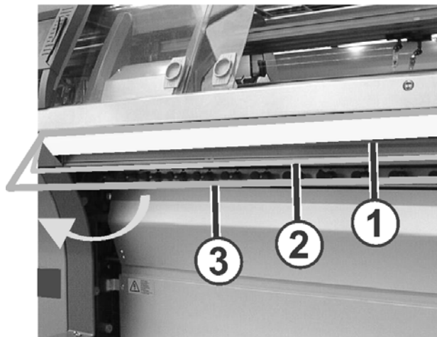
Fig. 2-38 Einrückstange
