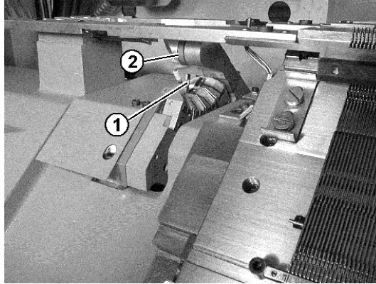
Fig. 2-9 Fadenklemm- und Schneideinrichtung
