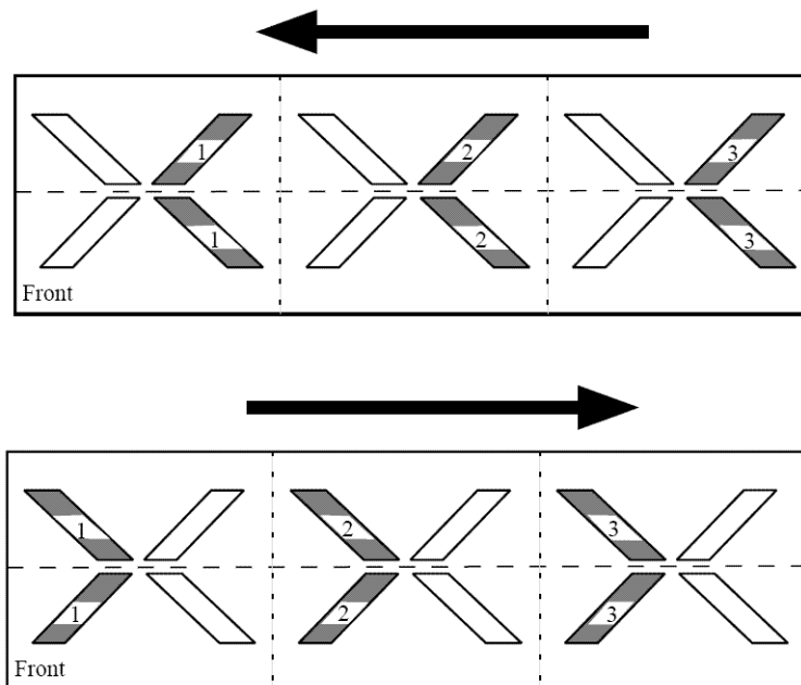
Fig. 4-62 Nummerierung der Abzugsteile für eine 3-systemige Maschine
