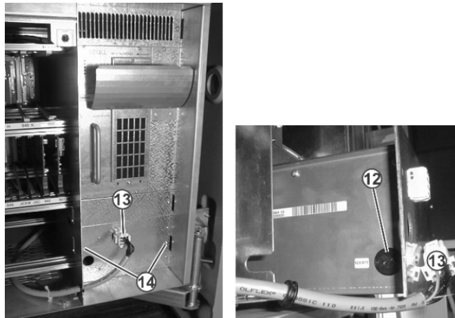
Fig. 6-67 Batteriesicherung (12) unterhalb des Netzgerätes
