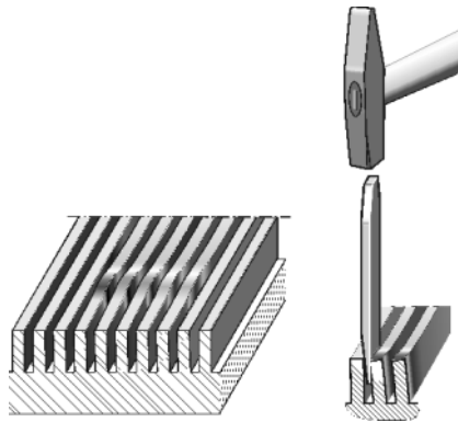
Fig. 6-23 Stege senkrecht stellen
