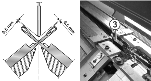
Fig. 4-67 Einstellen der Fadenführer
