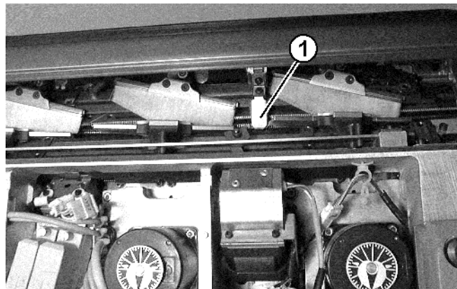
Fig. 2-23 Nadelwächter
