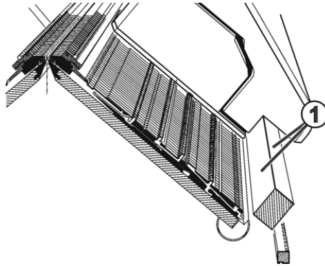
Fig. 5-41 Ölen des Schlittenführungsstabs
