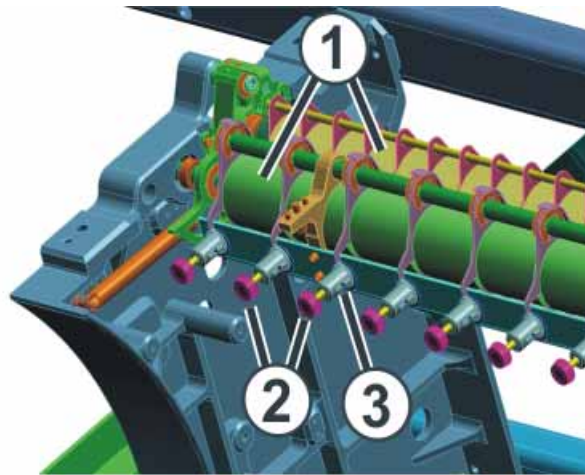
Fig. 2-33 Hauptabzug
