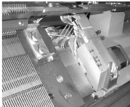
Fig. 5-27 Zahnriemen in Pfeilrichtung spannen
