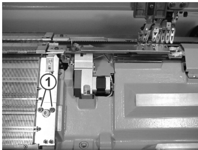
Fig. 6-17 Lösen des Nadelbetts
