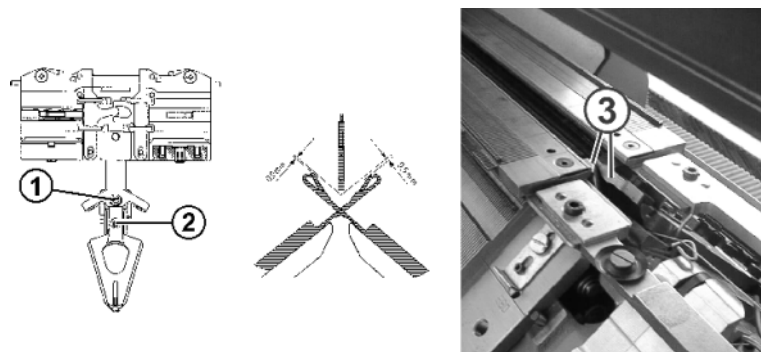
Fig. 4-72 Einstellen der Intarsienfadenführer
