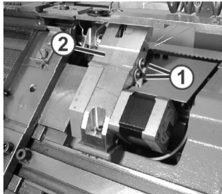
Fig. 5-24 Schrauben des Fingerträgers
