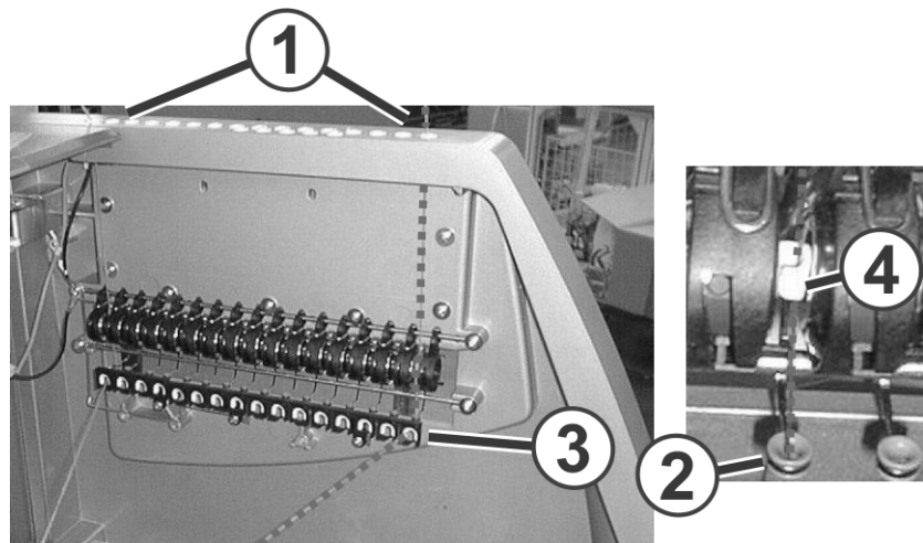
Fig. 3-13 Weg des Fadens durch die seitliche Sicherheitshaube
