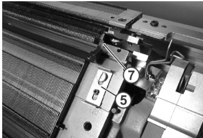
Fig. 6-13 Draht als Platinenhalterung
