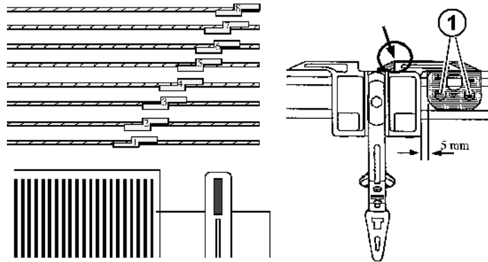
Fig. 4-68 Einstellen der Fadenführerbegrenzer
