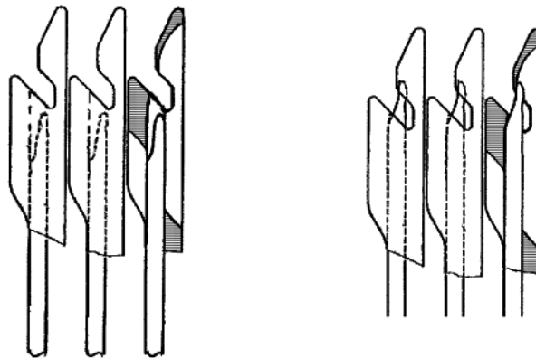
Fig. 2-36 Kammhaken des Kammabzugs mit Schiebern (links offen, rechts geschlossen)
