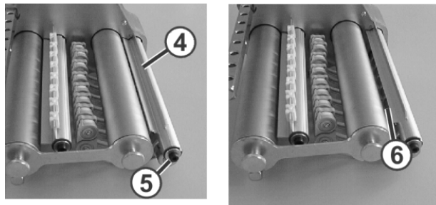
Fig. 4-12 Abstand einstellen zwischen Absteilschiene und Friktionswalze
