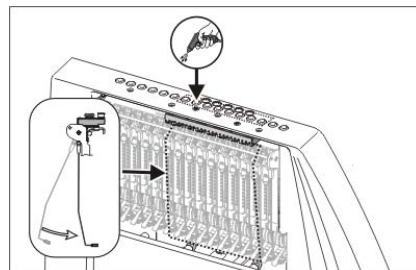
Fig. 5-10 Reinigen der aktiven Fadenklemme
