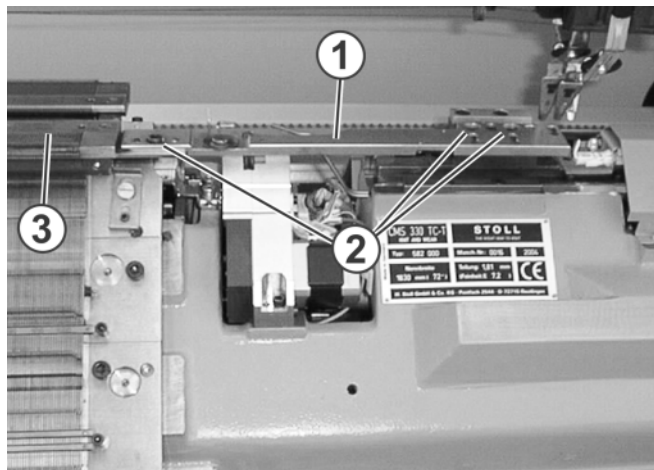
Fig. 6-11 Abnehmen der Anbindungen
