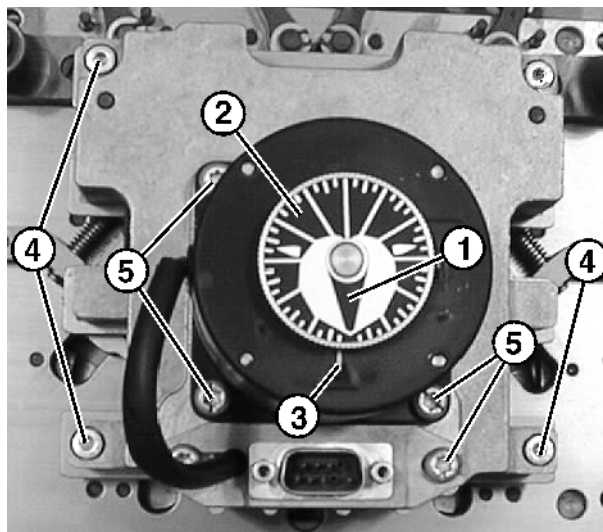
Fig. 6-43 Abnehmen des Schrittmotors
