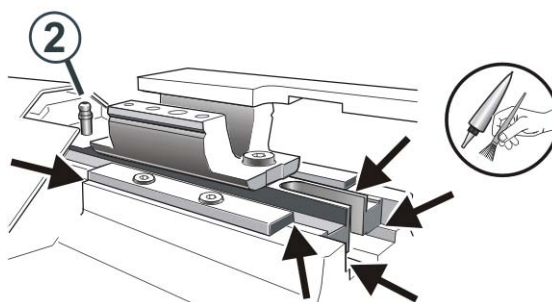
Fig. 5-47 Versatzeinrichtung der Zusatzbetten fetten
