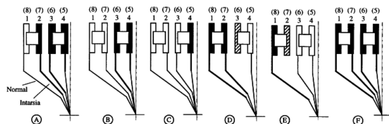
Fig. 6-54 Kombinationsmöglichkeiten für Normal- und Intarsienfadenführer
