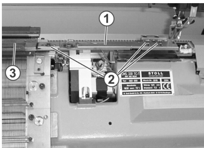
Fig. 6-19 Abnehmen der Zusatzbetten
