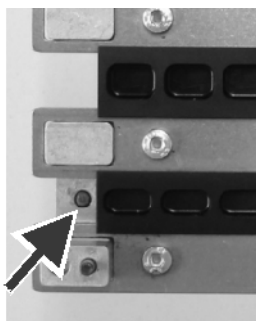
Fig. 6-45 Stift der Zahnstangenführung
