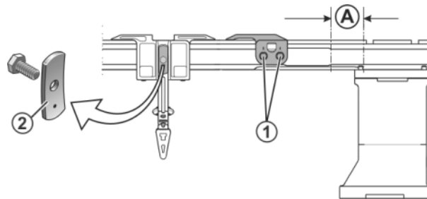
Fig. 6-53 Schrauben des Fadenführerbegrenzers
