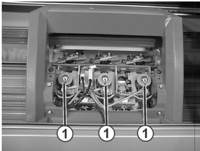
Fig. 2-20 Schrittmotor zur Einstellung der Maschenfestigkeit
