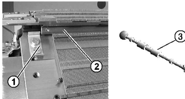
Fig. 6-5 Nadelschiene und Ausziehhaken
