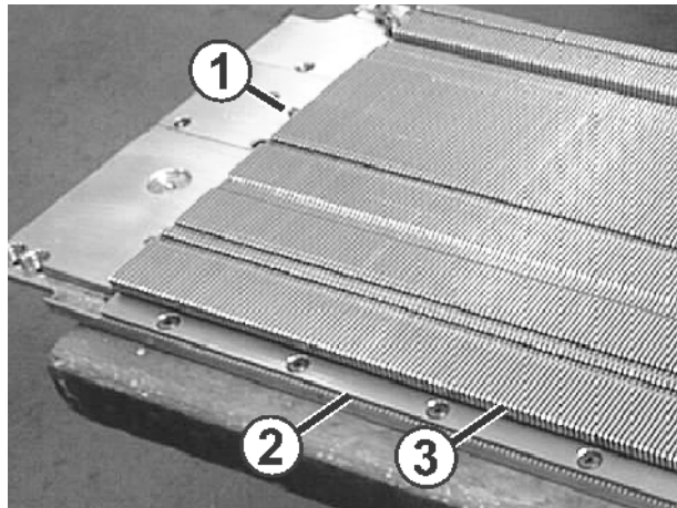
Fig. 6-26 Reparatur eines zusammengesetzten Nadelbetts
