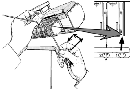
Fig. 3-12 Weg des Fadens durch das STIXX-Gerät
