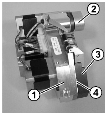
Fig. 5-28 Gehäuse der Fadenklemm- und Schneideinrichtung
