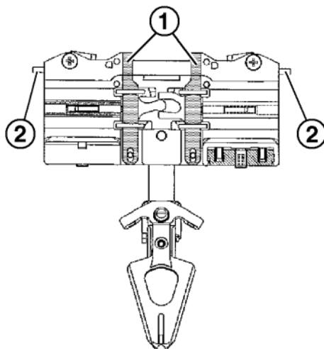
Fig. 6-56 Intarsienfadenführer
