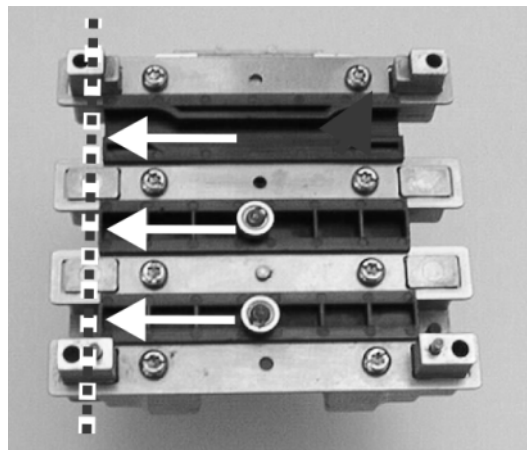
Fig. 6-47 Kontrolle der Einbauposition
