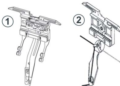
Fig. 2-12 Plattierfadenführer
