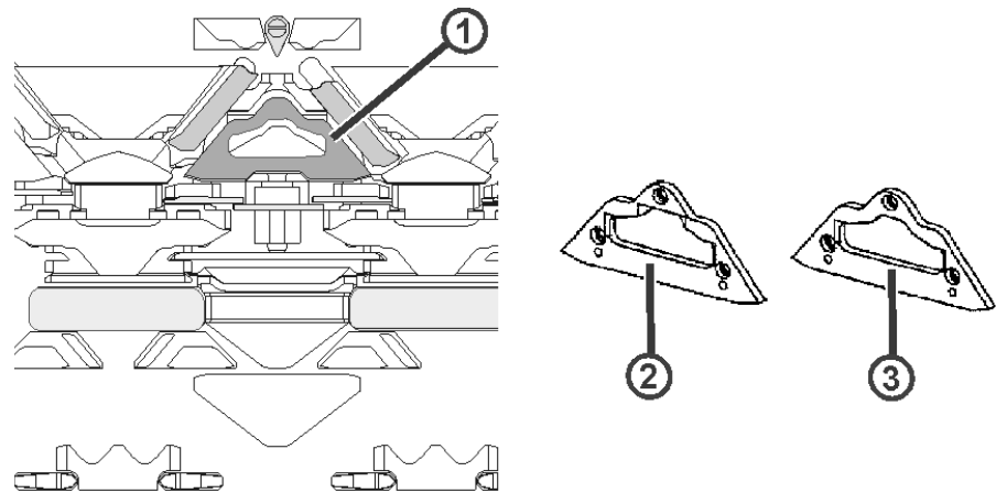
Fig. 2-18 Strickaustriebsteile
