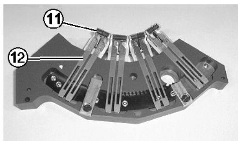
Fig. 5-33 Selektionsgehäuse
