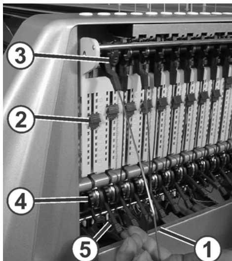
Fig. 4-9 Einstellen der Fadenspannung
