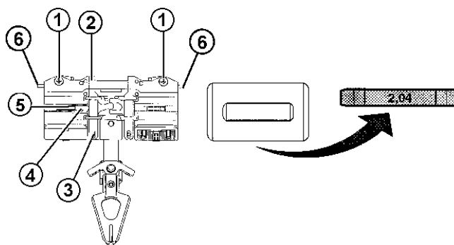
Fig. 4-74 Ausbau des Druckplättchens
