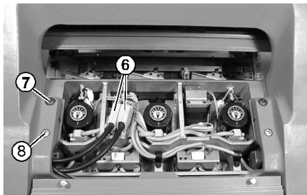
Fig. 6-30 Geöffneter Schlittenwagen
