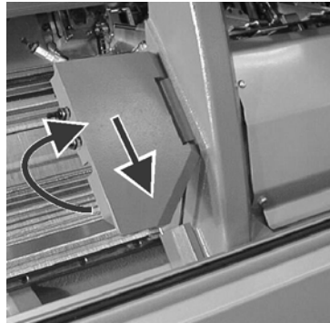
Fig. 6-2 Montagestellung der Zentralschmierung
