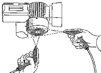
Fig. 5-6 Reinigen der Motorabdeckung
