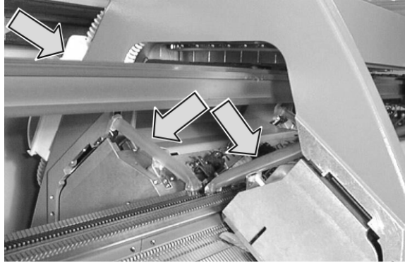
Fig. 2-14 Flusenentsorgung und Flusenbehälter (ab Baumuster 001)
