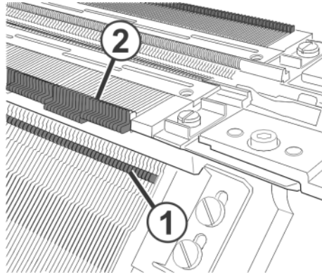
Fig. 5-39 Ölen der Füße der Niederhalteplatte (1) und der Umhängeteile (2)
