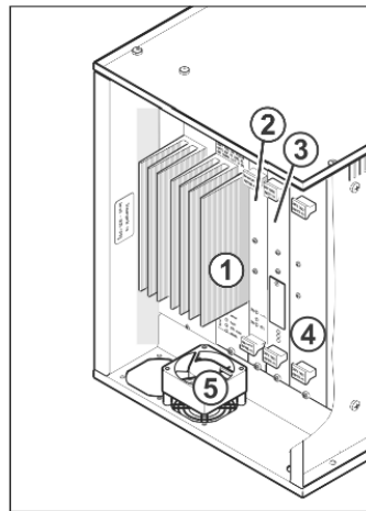
Fig. 6-63 Steuerschrank rechts
