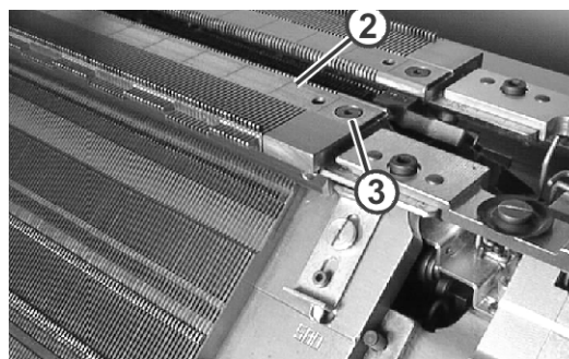
Fig. 6-10 Zusatzbett
