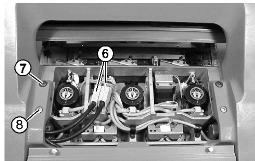
Fig. 6-36 geöffneter Schlittenwagen
