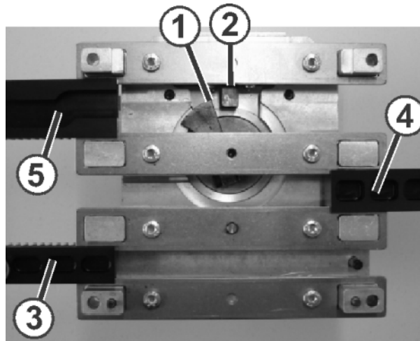
Fig. 6-46 Einbauposition
