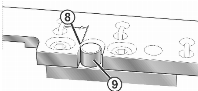
Fig. 6-14 Positionierung der Anbindung
