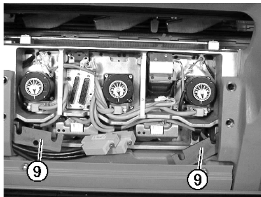
Fig. 6-31 Linke und rechte Schwenkplatte
