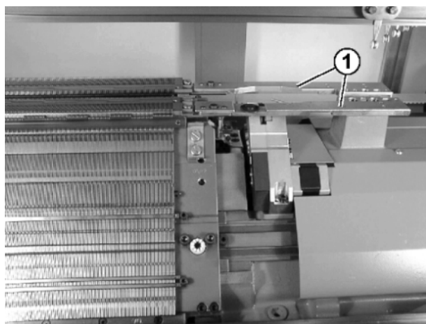
Fig. 6-48 Anbindung des Zusatzbetts
