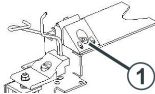
Fig. 4-64 Einstellen der Fadenklemme
