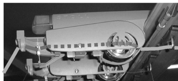
Fig. 3-11 Weg des Fadens durch die Fadenkontrolleinrichtung
