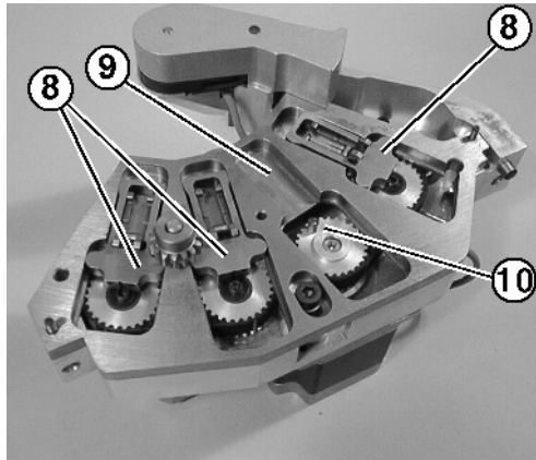
Fig. 5-32 Kurbelgehäuse
