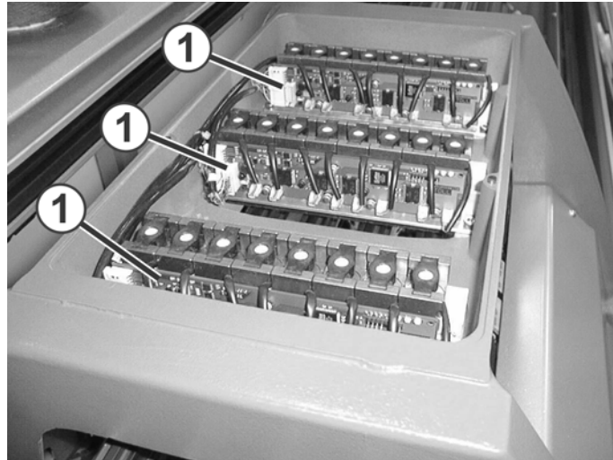
Fig. 6-65 Elektronikkarten zur Steuerung der Fadenführermagnete
