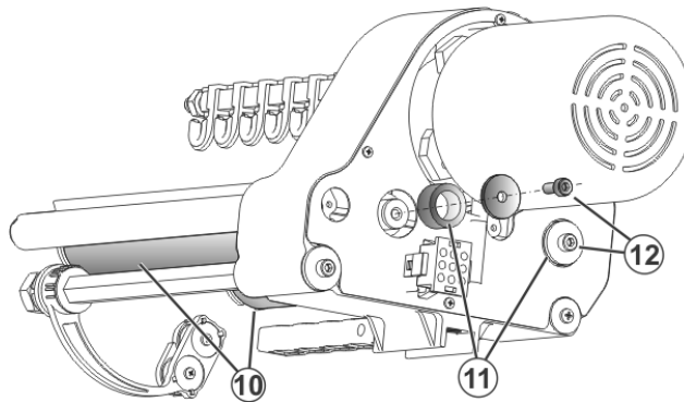
Fig. 6-61 Schrauben für Friktionswalzen
