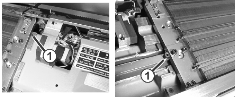
Fig. 6-20 Einbau des vorderen und hinteren Nadelbetts
