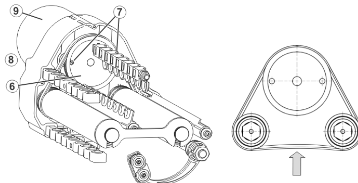
Fig. 6-60 Antriebsriemen
