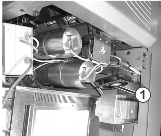
Fig. 5-15 Lüfter Hauptantrieb
