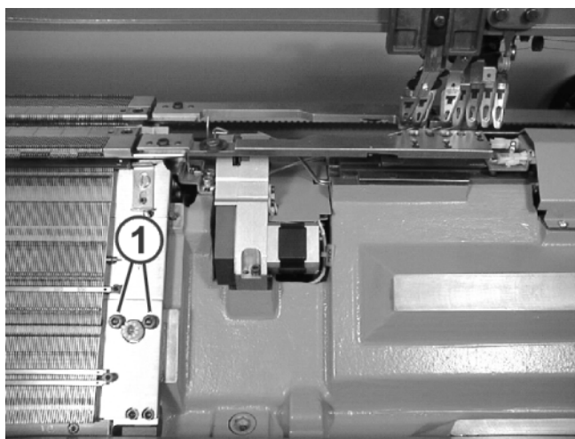
Fig. 6-15 Lösen des Nadelbetts
