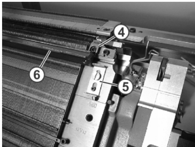
Fig. 6-12 Austausch einer Platine
