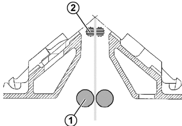
Fig. 2-34 Hilfsabzug
