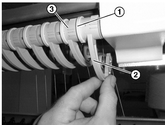
Fig. 4-11 Einstellung der Fadenlieferung am Friktionsfournisseur
