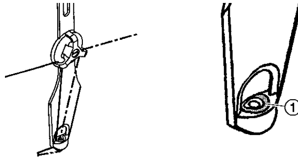
Fig. 4-75 Langloch des Plattierfadenführers
