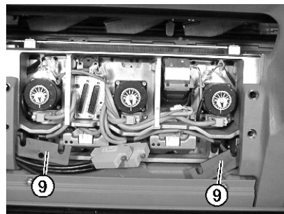
Fig. 6-37 Linke und rechte Schwenkplatte
