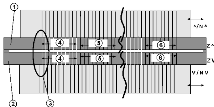
Fig. 4-55 Grundstellung der Nadelbetten zu den Zusatzbetten
