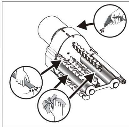
Fig. 5-12 Reinigen des Friktionsfournisseurs
