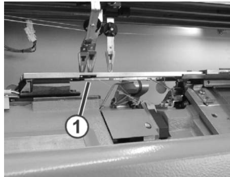
Fig. 2-22 Stoßabstellung für Zusatzbetten
