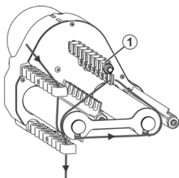
Fig. 4-10 Einstellung der Fadenlieferung am Friktionsfournisseur
