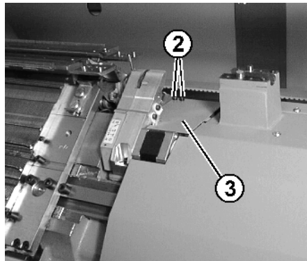
Fig. 6-49 Abdeckung der Fadenklemm- und Schneideinrichtung
