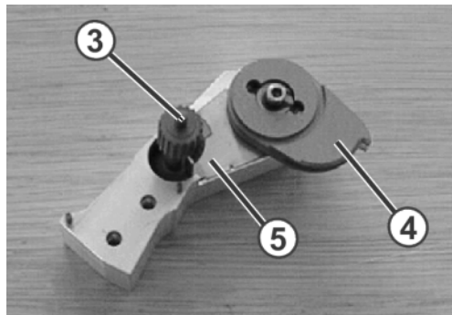
Fig. 5-25 Elemente des Fingerträgers
