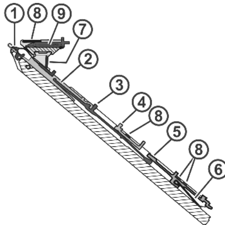
Fig. 2-24 Nadelbett
