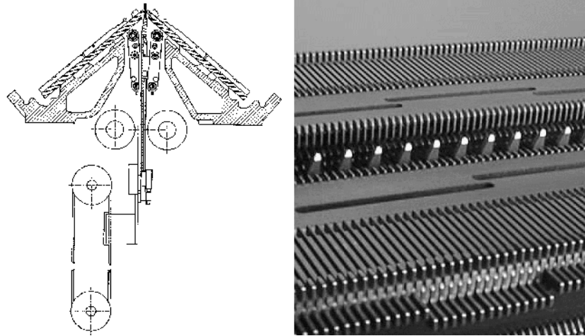
Fig. 2-35 Kammabzug
