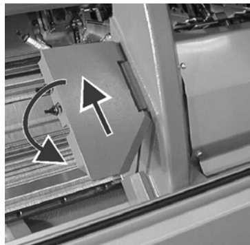
Fig. 6-3 Zentralschmierung in Arbeitsstellung schwenken
