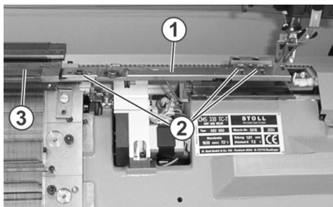
Fig. 5-20 Abnehmen der Zusatzbetten
