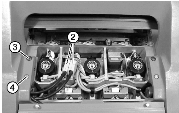
Fig. 6-40 Befestigung des Schlittenwagens am Schlittenteil
