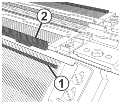
Fig. 5-49 Fetten der Mitnahmefüße und der Umhängeteile
