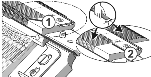
Fig. 5-9 Zusatzbett
