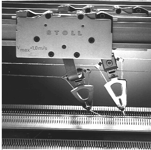
Fig. 2-11 Intarsienfadenführer
