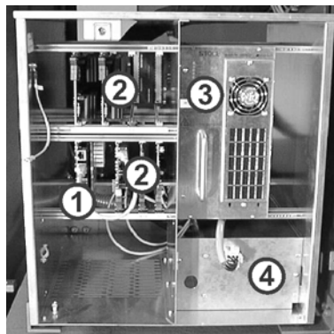
Fig. 6-62 Steuerschrank links
