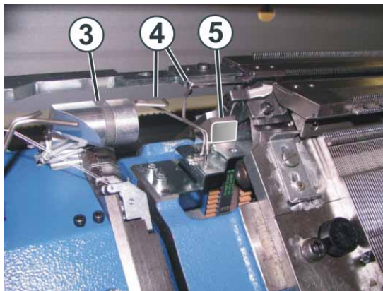
Fig. 2-10 Fadenleitsystem
