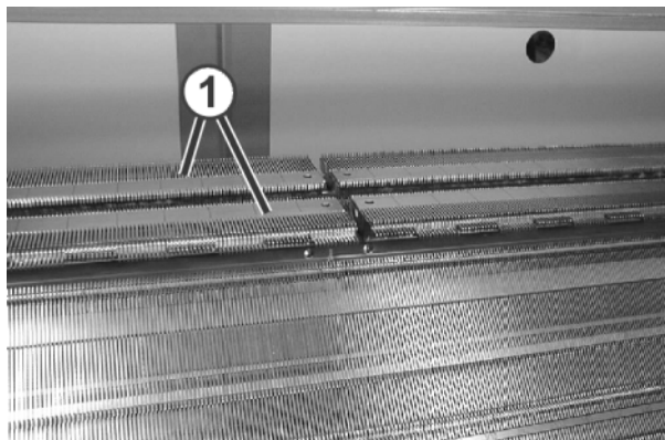
Fig. 2-27 Geteilte Zusatzbetten
