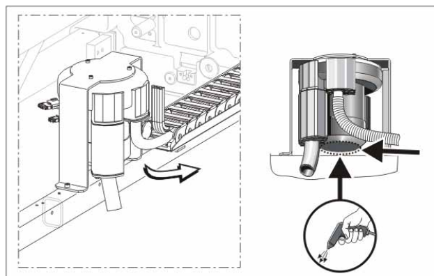
Fig. 5-2 Reinigen der Motorabdeckung
