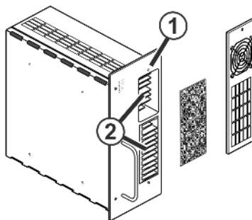
Fig. 5-17 Lüfter Netzteil
