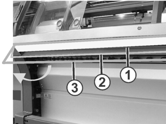
Fig. 3-19 Einrückstange
