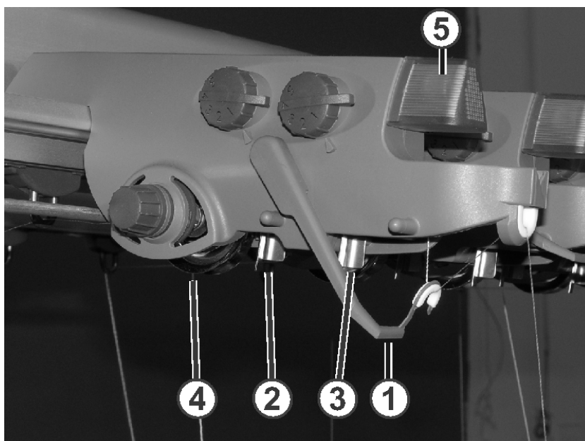
Fig. 2-5 Fadenkontrollleinrichtung
