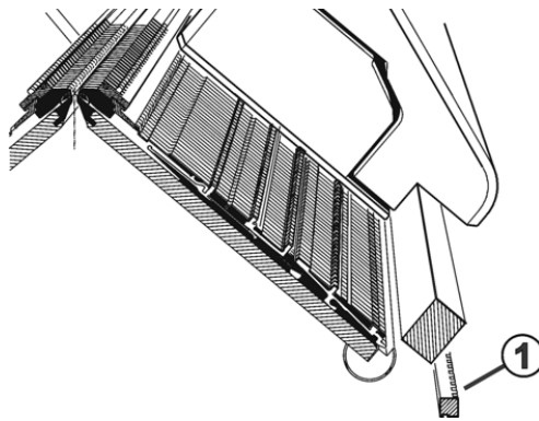
Fig. 5-42 Fetten der Impulsgeberschienen
