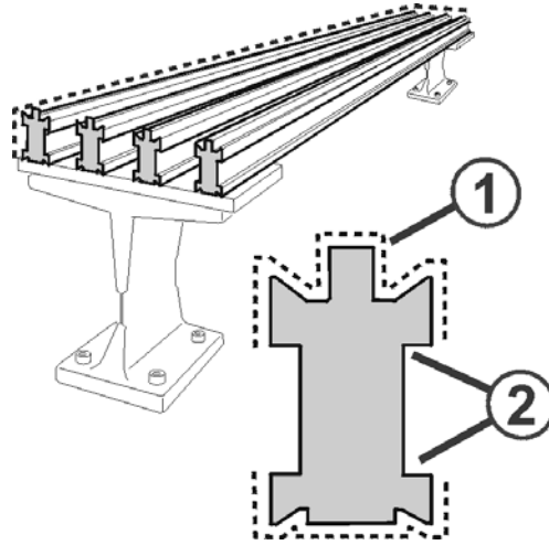
Fig. 5-45 Fetten der Fadenführerstäbe
