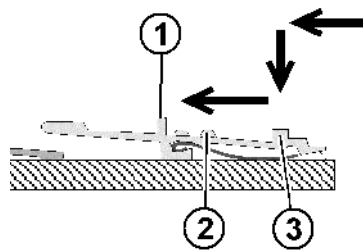
Fig. 6-8 Wechseln der Auswahlplatine
