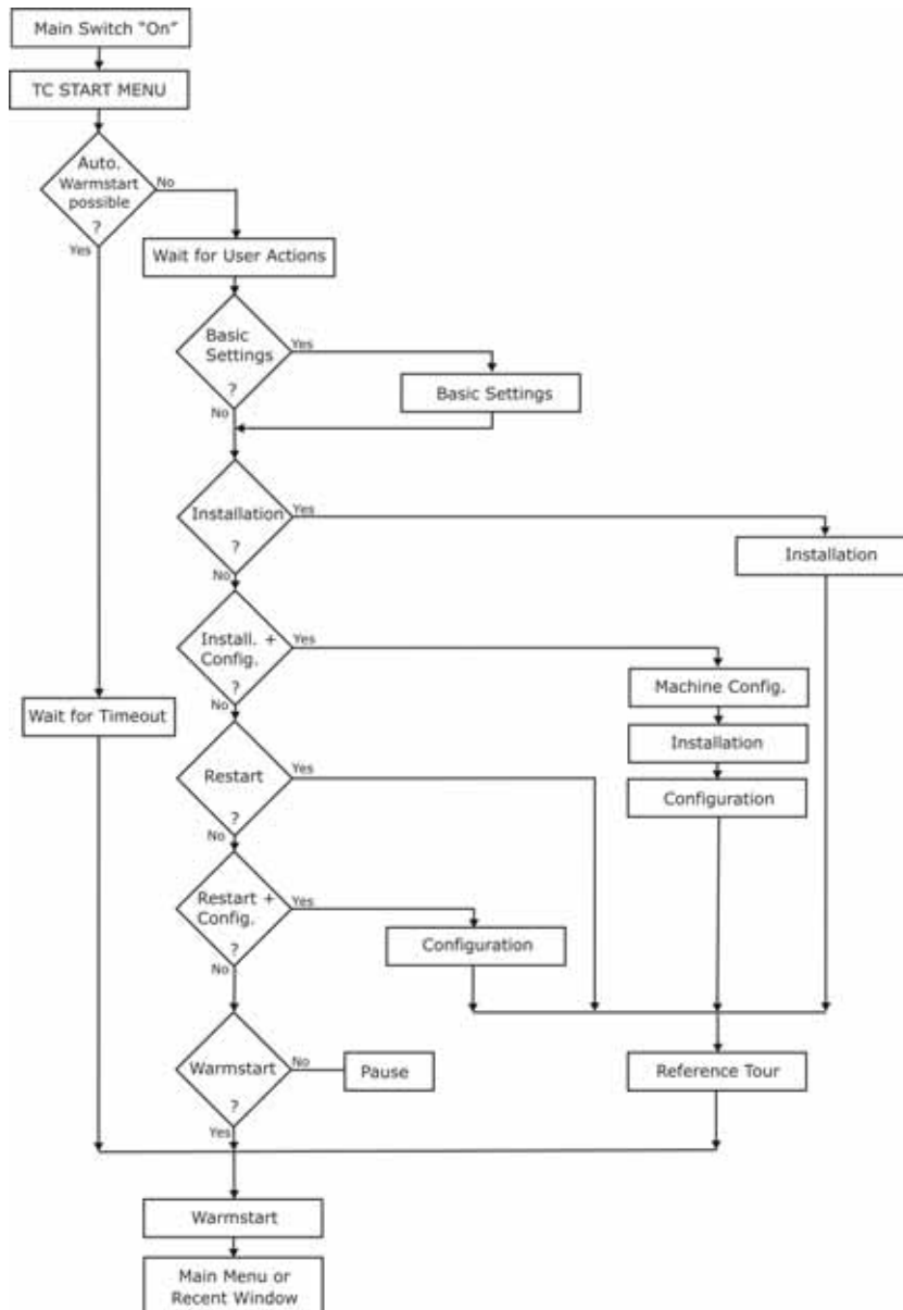
Fig. 7-1 Schematische Darstellung des Bootvorgangs
