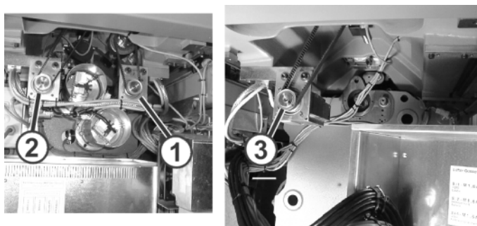
Fig. 2-26 Versatzmotoren
