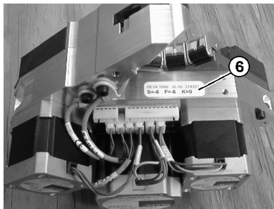
Fig. 6-51 Aufkleber Korrekturwerte
