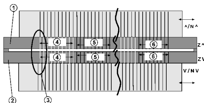
Fig. 4-55 Posición inicial de las fonturas hacia las fonturas adicionales
