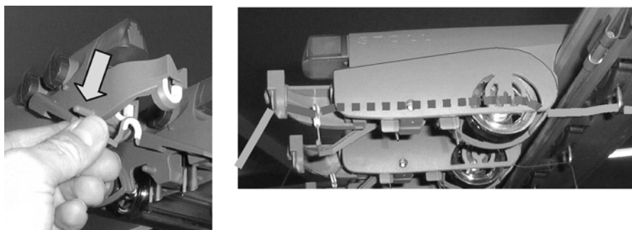
Fig. 3-11 Recorrido del hilo a través del dispositivo de control del hilo
