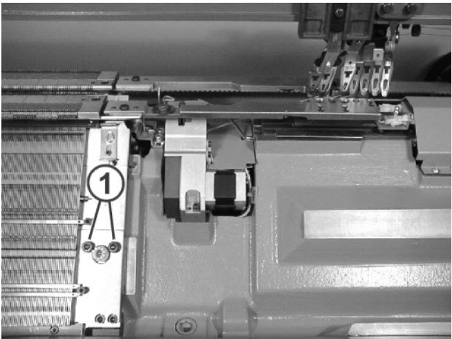
Fig. 6-17 Soltar la fontura
