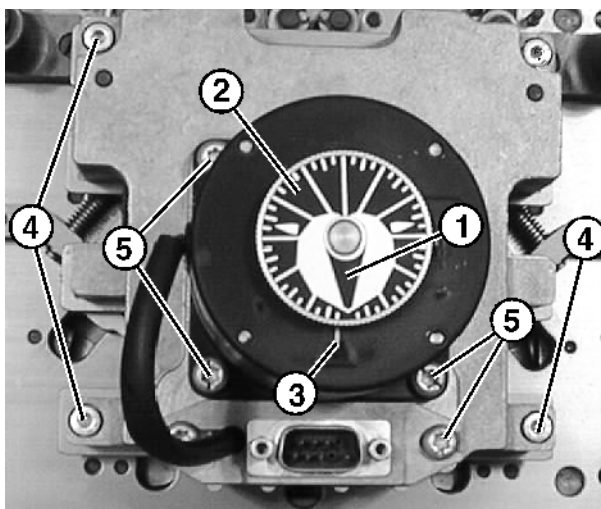
Fig. 6-43 Quitar el motor de paso a paso
