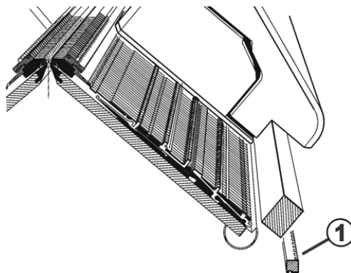
Fig. 5-42 Engrase de las barras ranuradas del generador de impulsos
