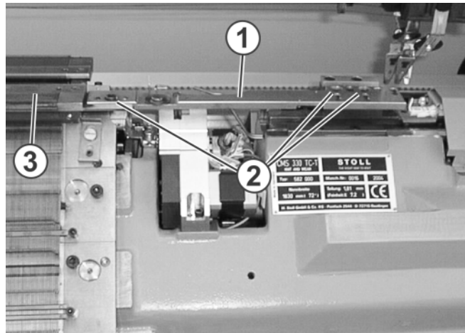
Fig. 6-11 Extracción de las ligaduras
