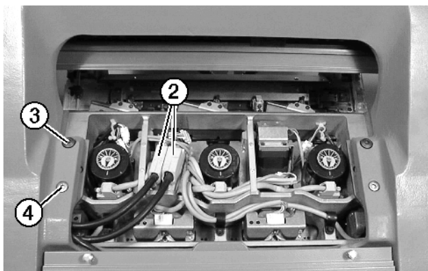
Fig. 6-40 Fijación del carro en la parte del carro
