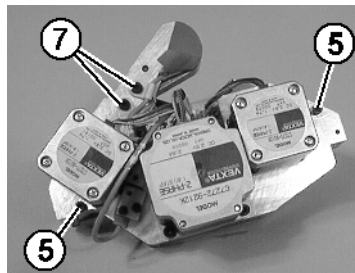
Fig. 5-29 Dispositivo de pinzado y corte del hilo
