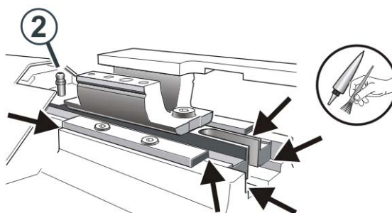
Fig. 5-47 Engrasar el dispositivo de variador de las fonturas adicionales
