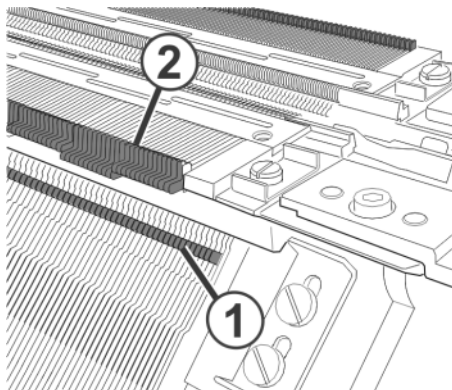
Fig. 5-49 Engrase de los talones de arrastre y de las piezas de transferencia
