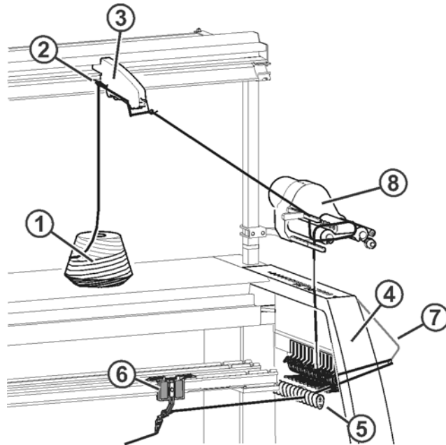
Fig. 2-3 Curso del hilo 3
