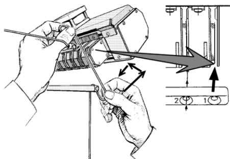
Fig. 3-12 Recorrido del hilo a través del aparato STIXX
