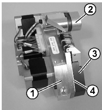
Fig. 5-28 Carcasa del dispositivo de pinzado y corte del hilo
