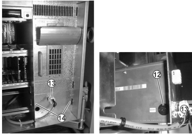
Fig. 6-67 El fusible de batería (12) debajo de la fuente de alimentación
