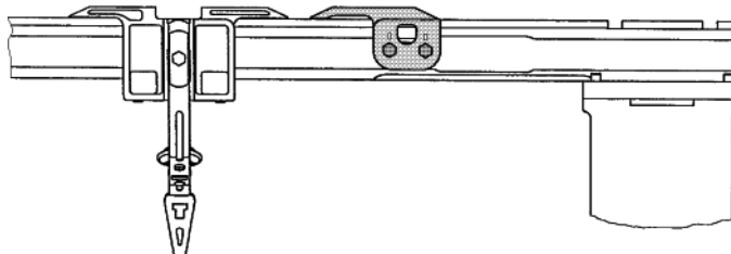
Fig. 6-55 Tope de guíahilos y reenvío del hilo
