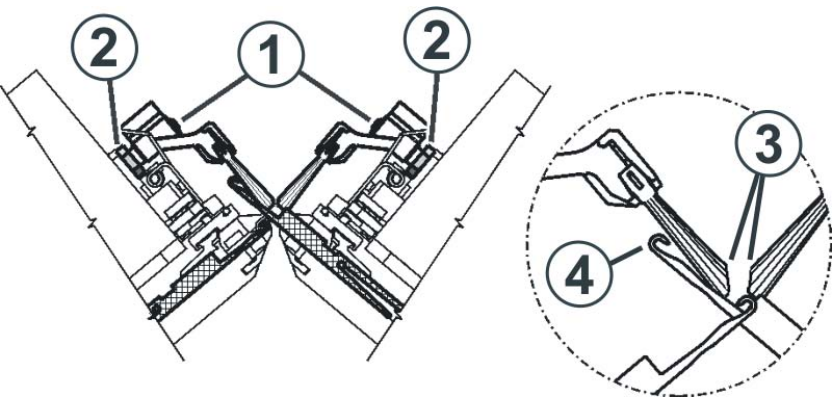
Fig. 4-63 Inclinación de los cepillos de las agujas
