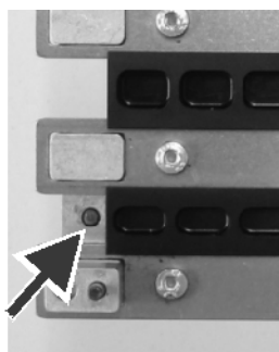
Fig. 6-45 Espiga de la guía de la barra dentada
