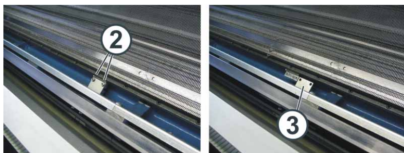
Fig. 6-18 Conexión del carril del generador de impulsos
