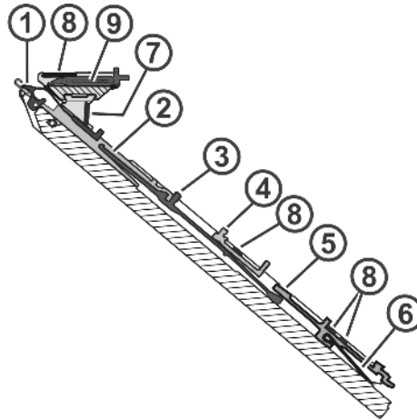
Fig. 2-24 Fontura
