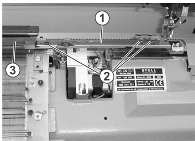
Fig. 6-19 Quitar las fonturas adicionales
