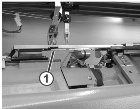
Fig. 2-22 Paro por choque para fonturas adicionales
