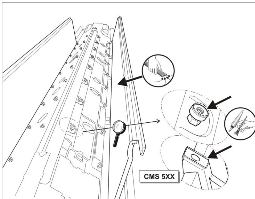
Fig. 5-50 Engrase de las piezas de ajuste
