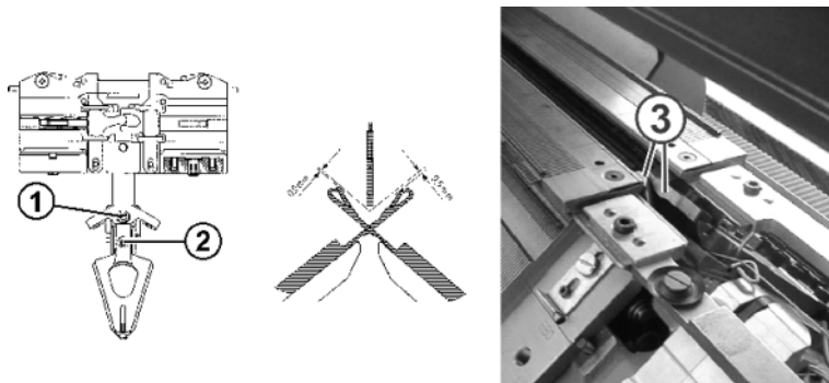
Fig. 4-72 Ajuste de los guíahilos de intarsia
