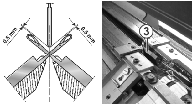
Fig. 4-67 Ajuste de los guiahilos
