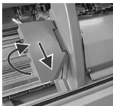
Fig. 6-2 Posición de montaje de la lubricación central
