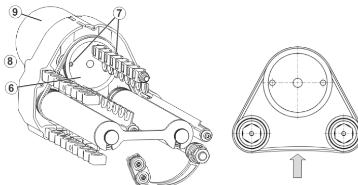
Fig. 6-60 Correa de accionamiento
