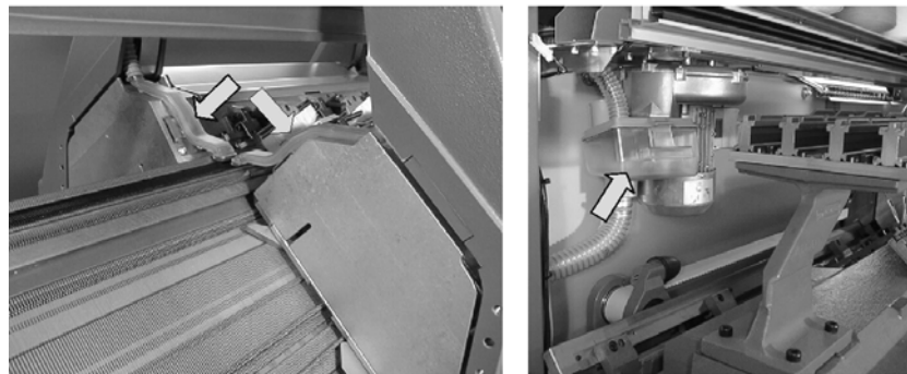
Fig. 2-15 Eliminación y depósito de pelusas (modelo de construcción 000)
