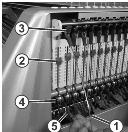
Fig. 4-9 Ajuste de la tensión del hilo
