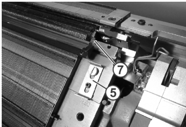
Fig. 6-13 Alambre como soporte de las platinas
