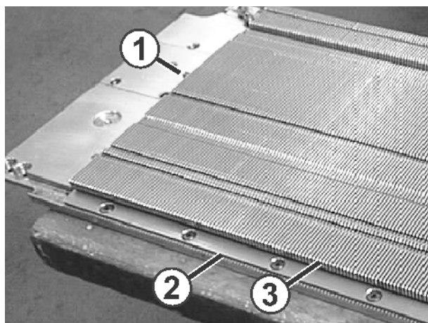
Fig. 6-26 Reparación de una fontura compuesta
