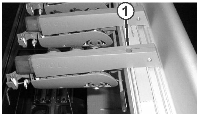
Fig. 6-58 Desmontaje de un dispositivo de control del hilo
