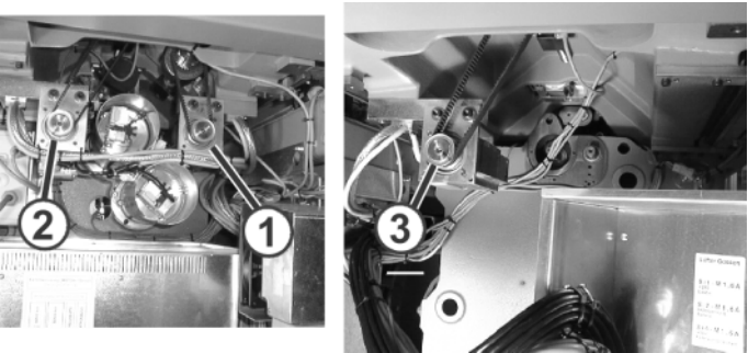
Fig. 2-26 Motores del variador
