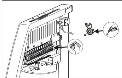
Fig. 5-11 Limpieza del freno permanente
