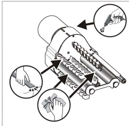
Fig. 5-12 Limpieza del alimentador de fricción
