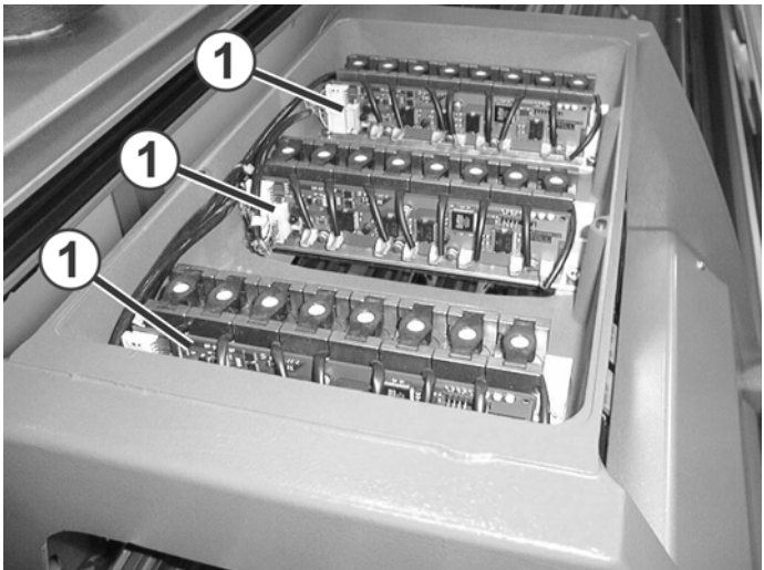
Fig. 6-65 Tarjetas electrónicas para controlar los imanes de los guíahilos
