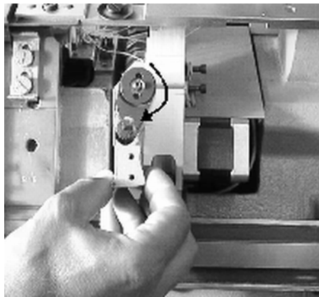
Fig. 5-26 Posición inicial del segmento de transporte
