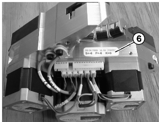
Fig. 6-51 Adhesivo de los valores de corrección
