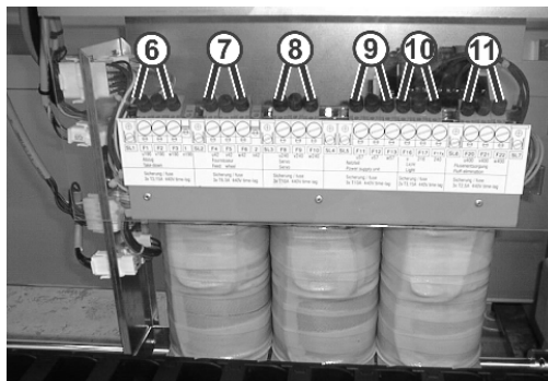
Fig. 6-69 Fusibles del transformador en la parte posterior de la máquina
