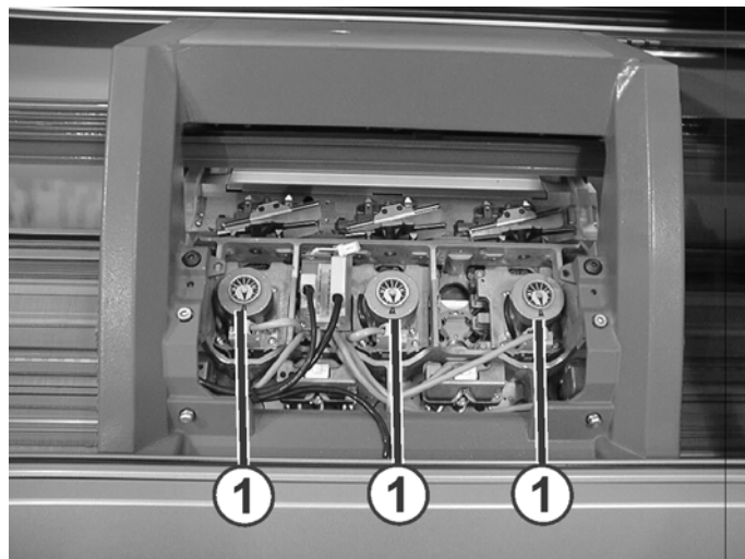
Fig. 2-20 Motor de paso a paso para el ajuste del cerraje del punto
