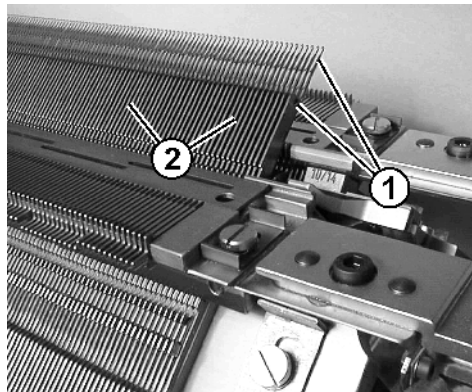
Fig. 5-8 Limpieza de la fontura
