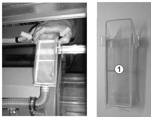
Fig. 5-1 Depósito de pelusas y filtro
