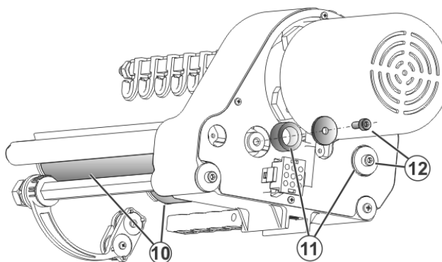
Fig. 6-61 Tornillos para el rodillo de fricción
