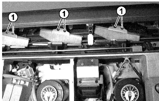
Fig. 4-66 Tornillos de los cepillos de las agujas
