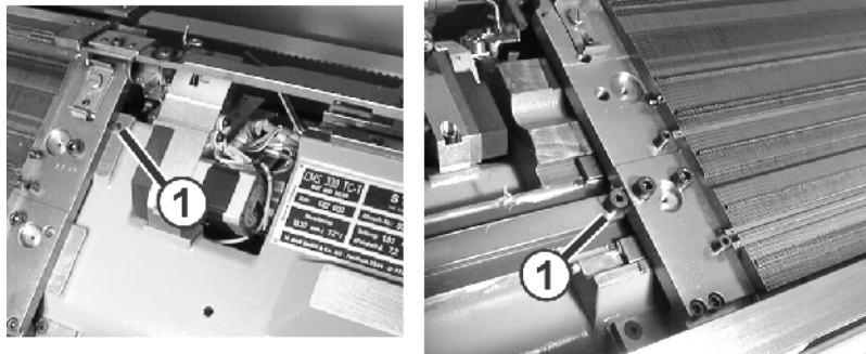
Fig. 6-20 Montaje de la fontura anterior y posterior
