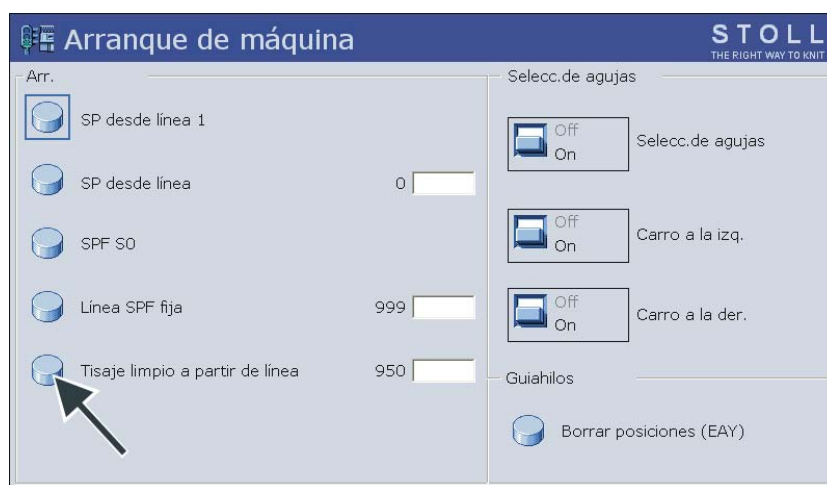
Fig. 3-34 Ventana "Arranque de la máquina"
