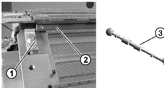
Fig. 6-5 Carril de la aguja y gancho extractor
