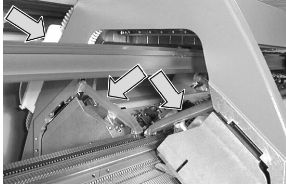
Fig. 2-14 Eliminación y depósito de pelusas (a partir del modelo de construcción 001)
