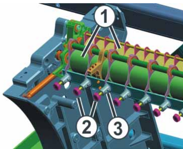
Fig. 2-33 Estirador principal
