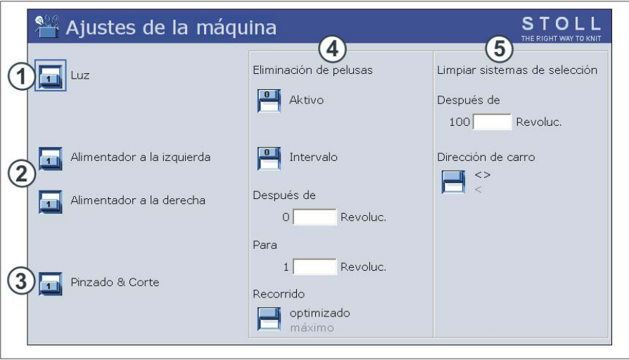
Fig. 4-40 Ventana "Ajustes de la máquina"
