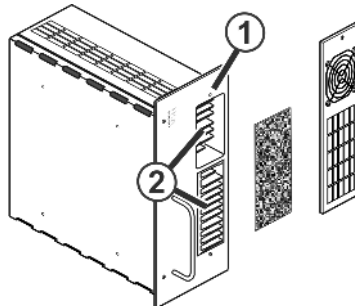
Fig. 5-17 Ventilador de la fuente de alimentación
