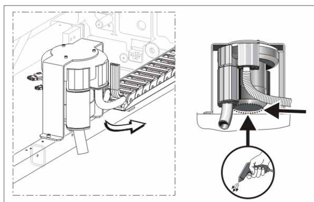
Fig. 5-2 Limpieza de la cubierta del motor
