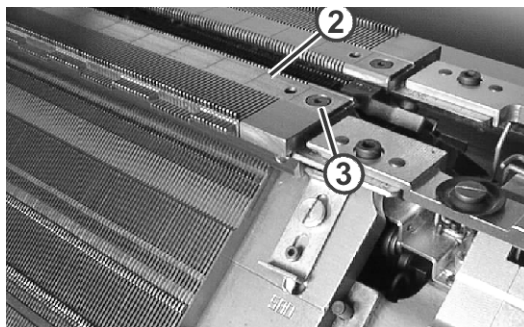
Fig. 5-23 Fontura adicional
