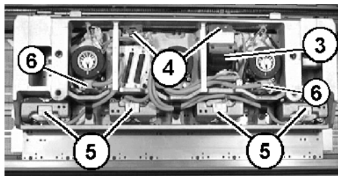
Fig. 6-41 Clavijas de los sistemas de selección
