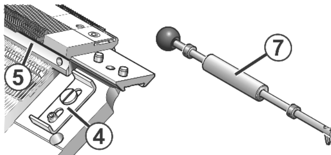
Fig. 5-21 Limpieza a fondo de la fontura
