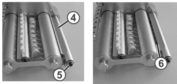
Fig. 4-12 Ajustar la distancia entre la guía de parada y el rodillo de fricción
