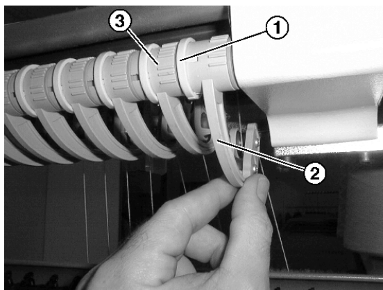
Fig. 4-11 Ajuste de la alimentación del hilo en el alimentador de fricción
