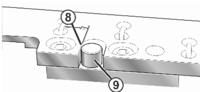
Fig. 6-21 Posicionamiento de las ligaduras
