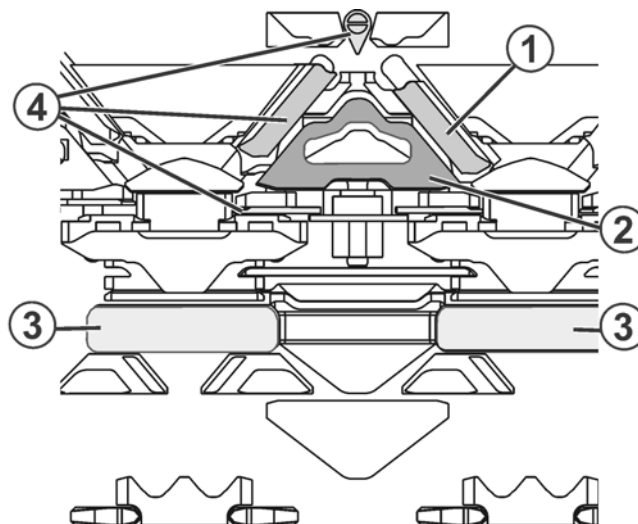
Fig. 2-17 Sistema de tisaje
