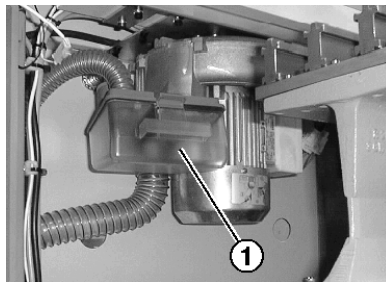
Fig. 5-4 Depósito de pelusas de la aspiración
