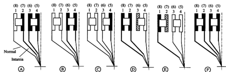
Fig. 6-54 Combinaciones posibles para guíahilos normales y guíahilos de intarsia
