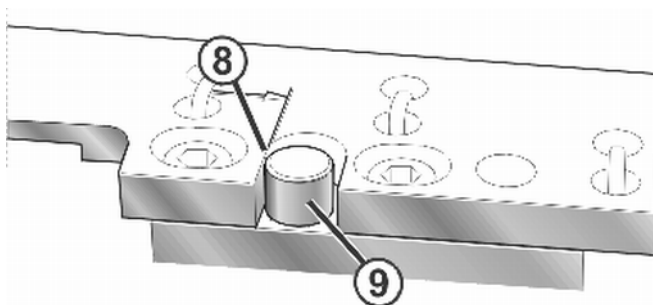
Fig. 6-14 Posicionamiento de las ligaduras
