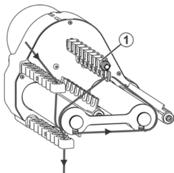
Fig. 4-10 Ajuste de la alimentación del hilo en el alimentador de fricción
