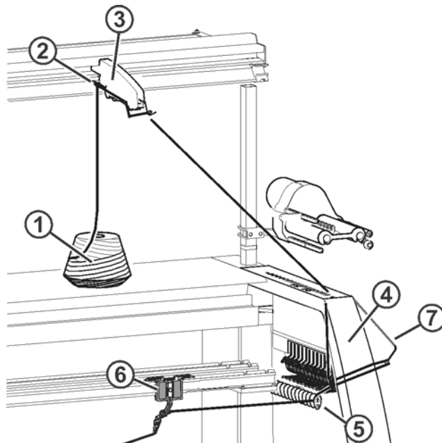
Fig. 2-2 Curso del hilo 2
