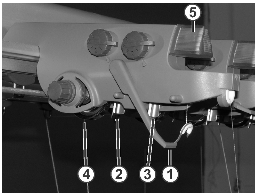
Fig. 2-5 Dispositivo del control del hilo
