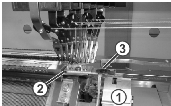
Fig. 4-8 Enhebrar el hilo
