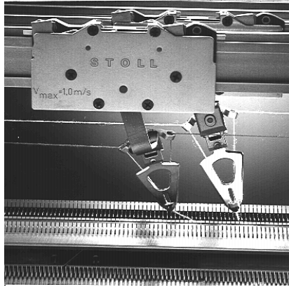
Fig. 2-11 Guíahilos de intarsia
