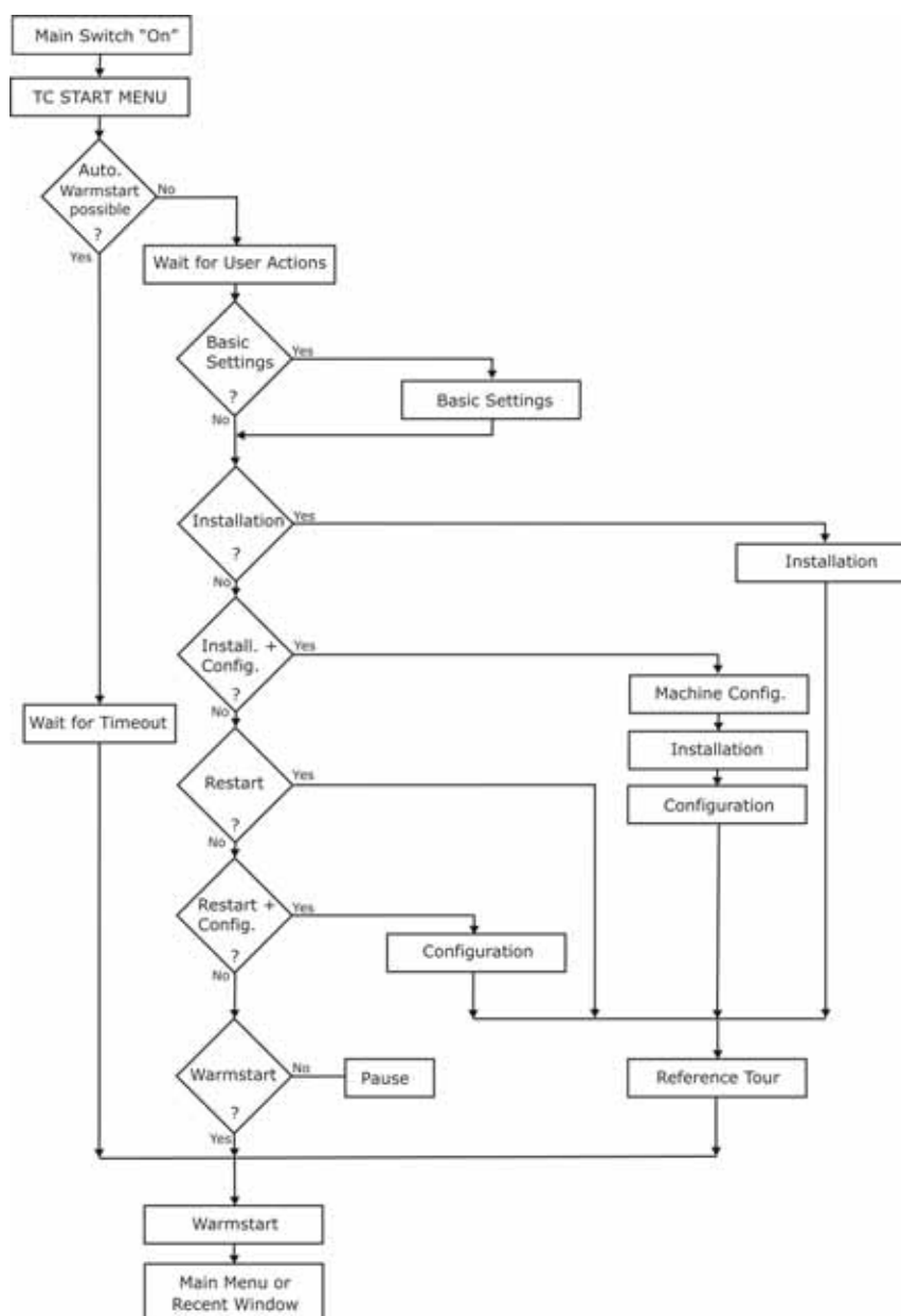
Fig. 7-1 Representación esquemática del procedimiento de inicialización
