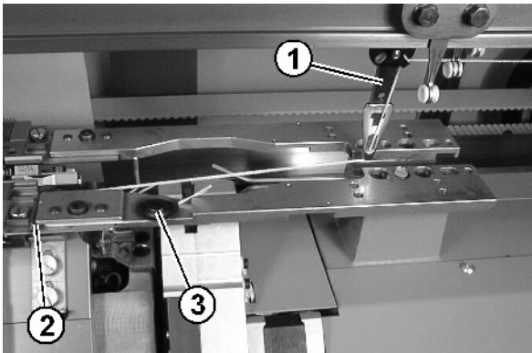
Fig. 3-16 Enhebrar el hilo
