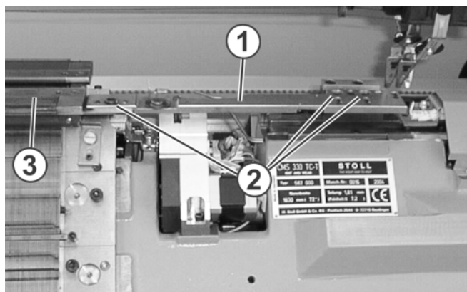
Fig. 5-20 Quitar las fonturas adicionales
