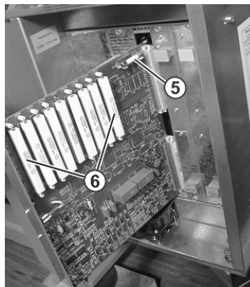
Fig. 6-68 Fusible de sobrecarga (5) para el accionamiento servo y el variador (2 AT) a la derecha del aparato de mando:
