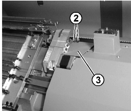
Fig. 6-49 Cubierta del dispositivo de pinzado y corte del hilo
