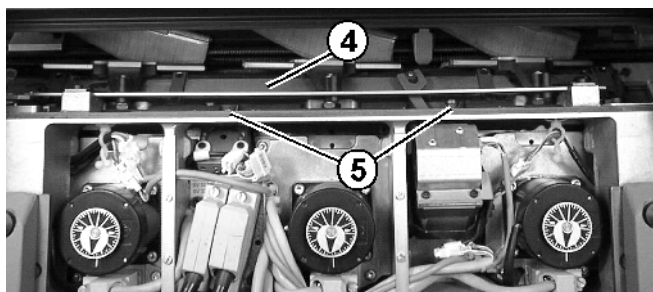
Fig. 6-29 Desmontar el cerrojo adicional
