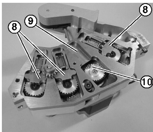
Fig. 5-32 Carcasa de la manivela
