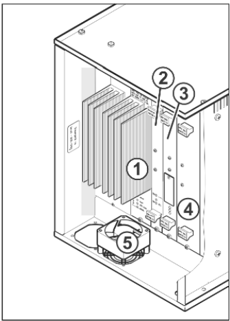
Fig. 6-63 Armario de mandos derecho
