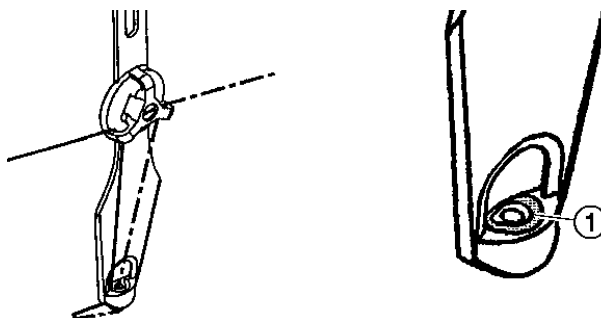
Fig. 4-75 Agujero alargado del guíahilos de vanisado
