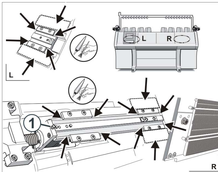
Fig. 5-46 Engrasar el dispositivo de variador
