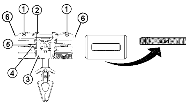
Fig. 4-74 Desmontaje de la plaquita de presión
