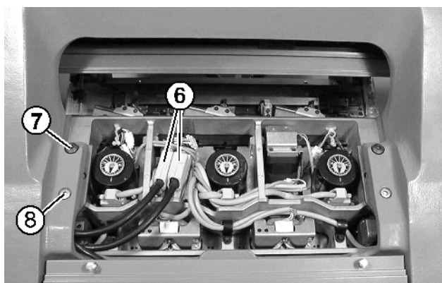
Fig. 6-30 Carro abierto
