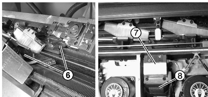
Fig. 2-29 Cerrojo adicional
