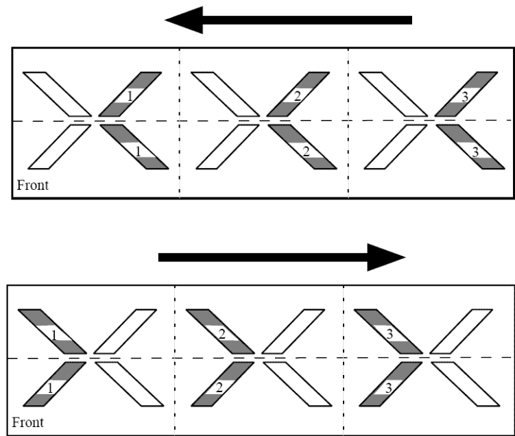
Fig. 4-62 Numeración de las levas de formación para una máquina de 3 sistemas
