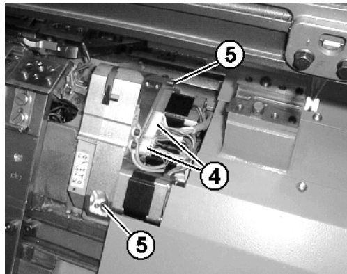
Fig. 6-50 Cable y tornillos del dispositivo de pinzado y corte del hilo
