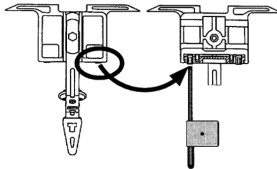
Fig. 4-69 Ajuste de la guía el guíahilos
