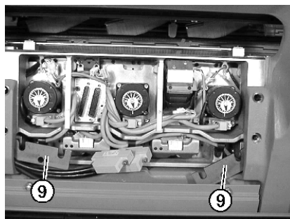
Fig. 6-37 Placas basculantes izquierda y derecha
