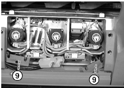
Fig. 6-31 Placas basculantes izquierda y derecha
