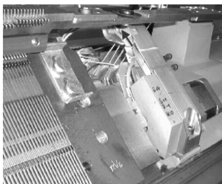
Fig. 5-27 Tensar la correa dentada en la dirección de la flecha
