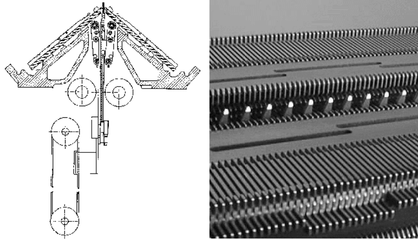
Fig. 2-35 Peine del estiraje
