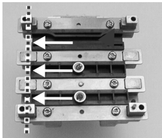
Fig. 6-47 Comprobación de la posición de montaje
