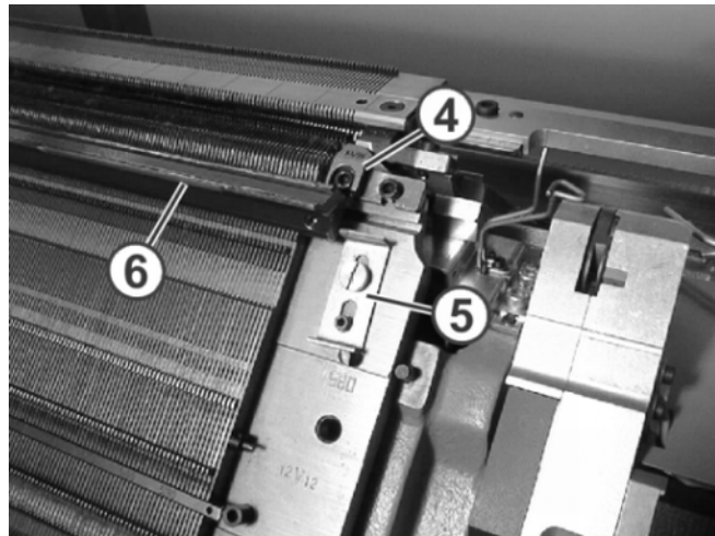
Fig. 6-12 Recambio de una platina
