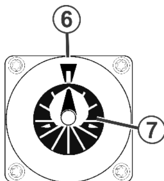
Fig. 6-44 Posición inicial del motor paso a paso
