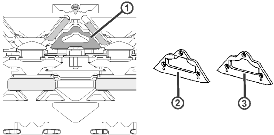
Fig. 2-18 Levas de desprendimiento
