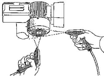
Fig. 5-6 Limpieza de la cubierta del motor
