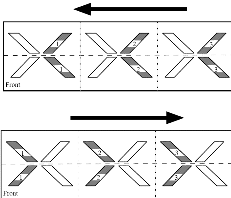
Fig. 4-62 Numérotation des cames de chute pour une machine à 3 systèmes
