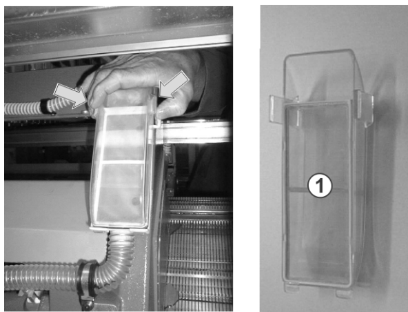
Fig. 5-1 Récepteur à peluches et filtre
