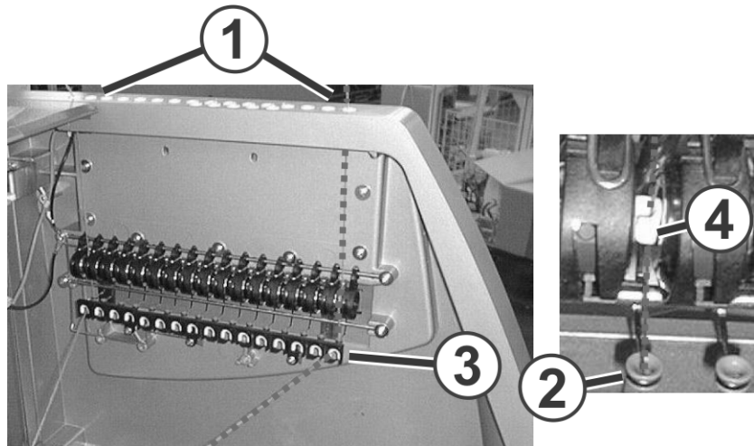
Fig. 3-13 Chemin du fil à travers le capot de sécurité latéral
