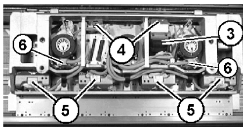
Fig. 6-41 Fiches des systèmes de sélection
