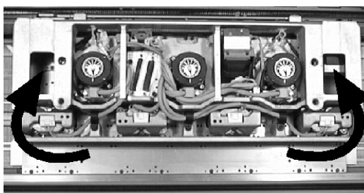
Fig. 6-38 Démontage de la pièce de chariot
