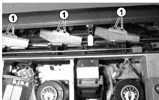
Fig. 4-66 Vis des brosses ouvre-clapets
