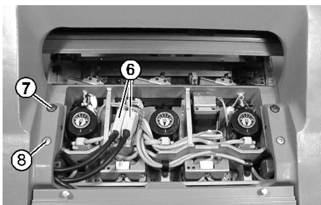
Fig. 6-30 Chariot ouvert
