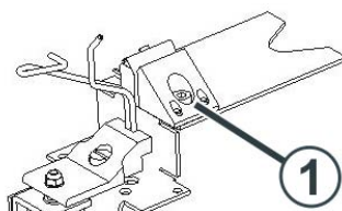
Fig. 4-64 Réglage de la pince-fil
