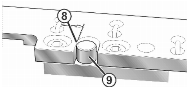
Fig. 6-14 Positionnement de la liaison
