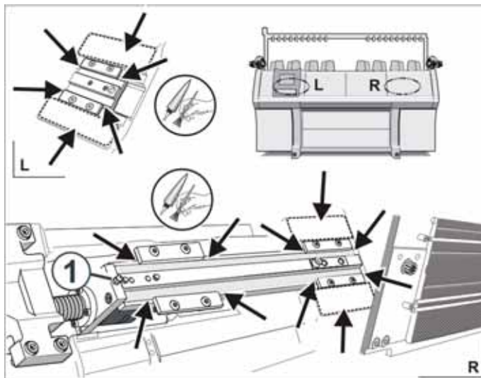
Fig. 5-46 Graisser le dispositif de chevalement
