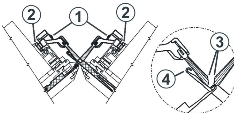
Fig. 4-63 Inclinaison des brosses ouvre-clapets
