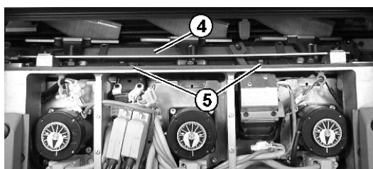
Fig. 6-35 Démontage de la came supplémentaire
