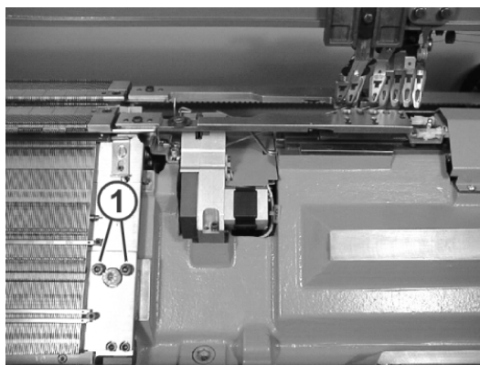
Fig. 6-15 Desserrer la fonture
