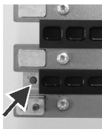
Fig. 6-45 Goupille du guidage de la crémaillère
