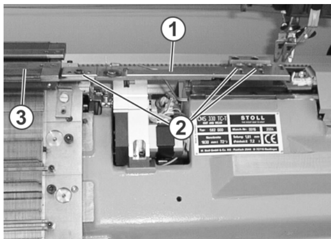
Fig. 6-11 Démontage des liaisons
