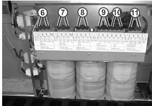
Fig. 6-69 Coupe-circuits au transformateur à l'arrière de la machine
