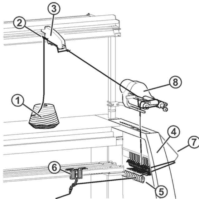
Fig. 2-3 Passage du fil 3
