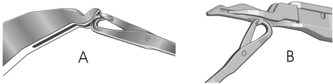
Fig. 4-51 Position de report de la pièce d'entraînement et du crochet d'aiguille
