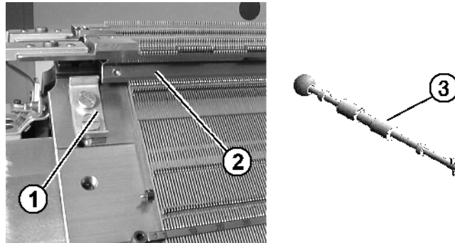
Fig. 6-5 Rail des aiguilles et crochet d'extraction
