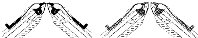
Fig. 2-19 Platines d'appui (à gauche: fermées, à droite: ouvertes)
