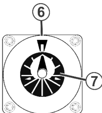
Fig. 6-44 Position de base du moteur pas à pas
