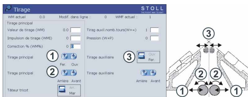
Fig. 3-36 Fenêtre "Tirage"
