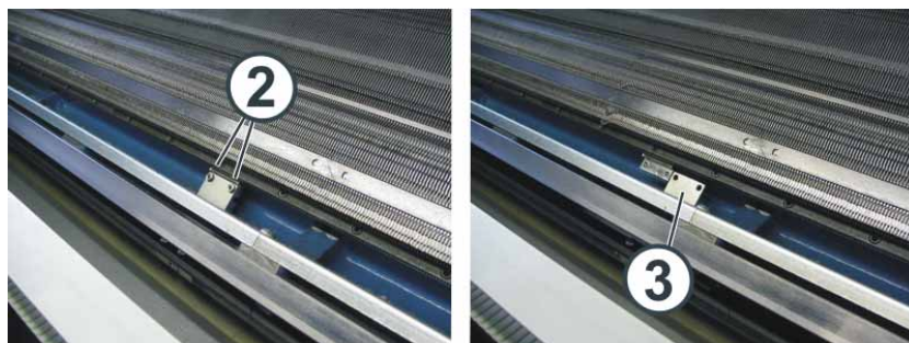
Fig. 6-18 Connexion du rail du générateur d'impulsions
