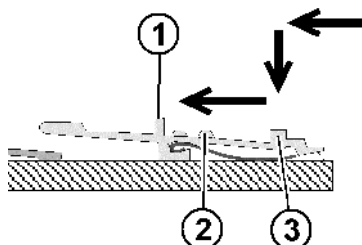
Fig. 6-8 Remplacement de la platine de sélection
