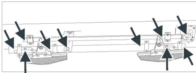
Fig. 5-48 Graissage du poussoir de commande, de la commande des brosses, de la came supplémentaire
