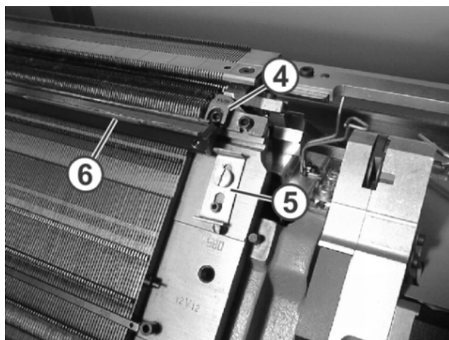
Fig. 6-12 Remplacement d'une platine
