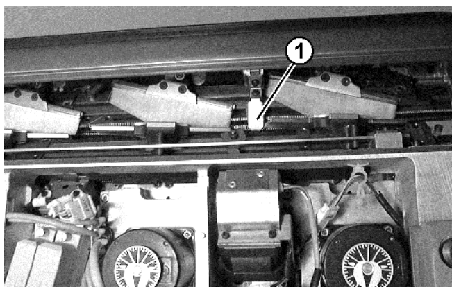
Fig. 2-23 Détecteur d'aiguilles
