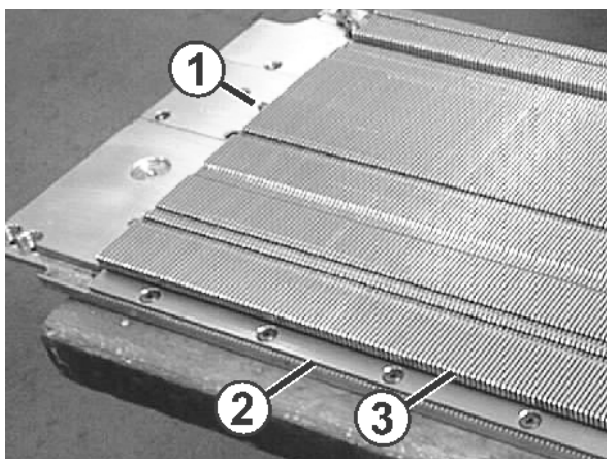
Fig. 6-26 Réparation d'une fonture assemblée
