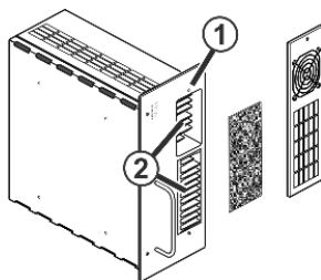
Fig. 5-17 Bloc d'alimentation du ventilateur
