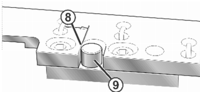
Fig. 6-21 Positionnement de la liaison
