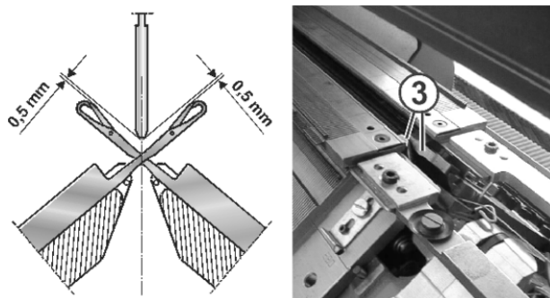
Fig. 4-67 Réglage des guide-fils
