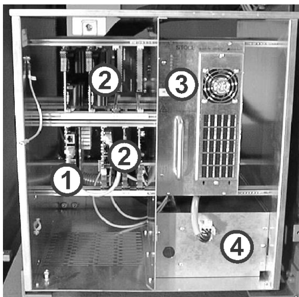
Fig. 6-62 Armoire de commande de gauche
