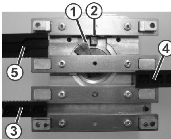
Fig. 6-46 Position de montage
