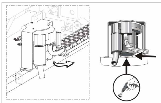
Fig. 5-2 Nettoyage du capot du moteur
