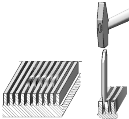
Fig. 6-23 Mettre les entretoises à la verticale
