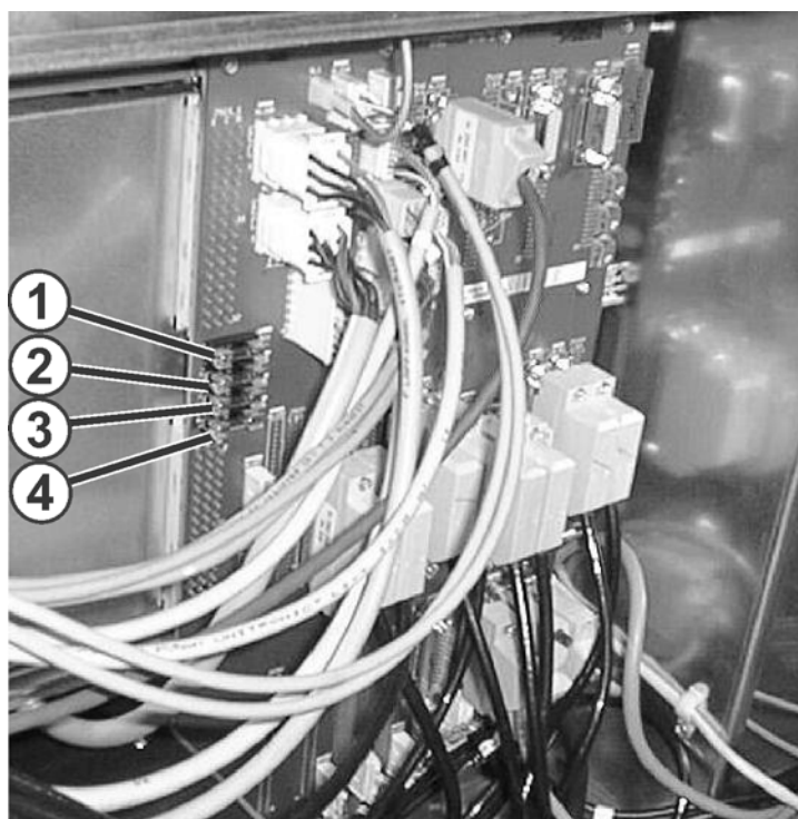
Fig. 6-66 Coupe-circuit à l'arrière de l'appareil de commande de gauche
