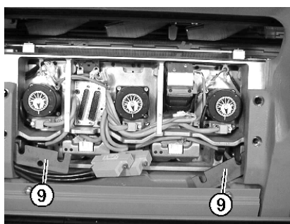
Fig. 6-37 plaque pivotante de gauche et de droite
