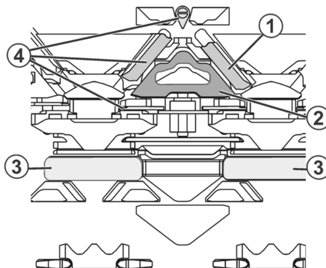
Fig. 2-17 Système de tricotage
