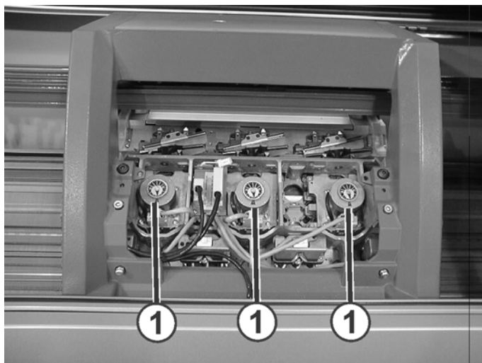
Fig. 2-20 Moteur pas à pas de réglage de la serre des mailles
