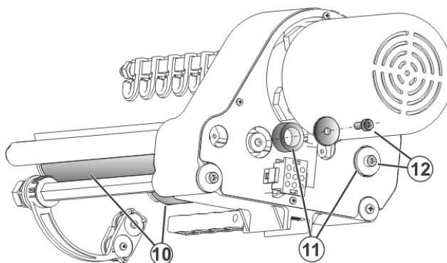
Fig. 6-61 Vis pour rouleaux à friction
