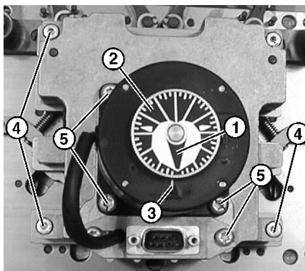
Fig. 6-43 Démontage du moteur pas à pas
