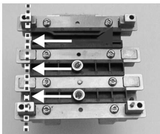
Fig. 6-47 Contrôle de la position de montage
