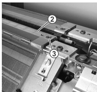
Fig. 5-23 Fonture supplémentaire
