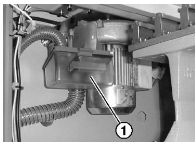
Fig. 5-4 Récipient à peluches de l'aspiration
