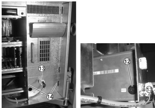
Fig. 6-67 Fusible de la batterie (12) en dessous du bloc d'alimentation
