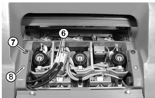
Fig. 6-36 chariot ouvert
