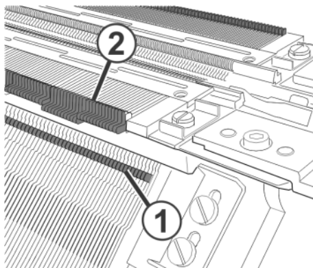
Fig. 5-39 Huiler les talons de la platine d'appui (1) et des pièces d'entraînement (2)
