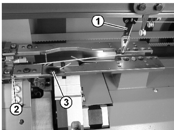
Fig. 3-16 Enfiler le fil
