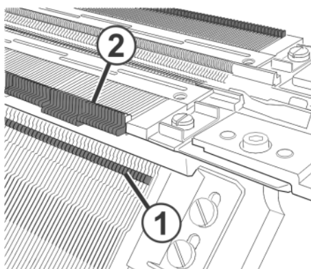
Fig. 5-49 Graissage des talons d'entraînement et les cames de report
