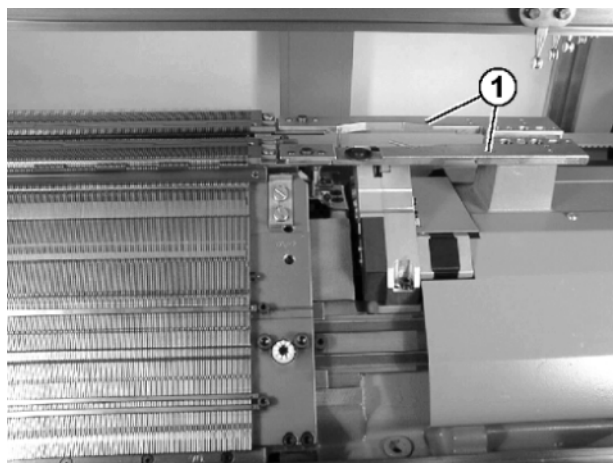
Fig. 6-48 Liaison de la fonture supplémentaire
