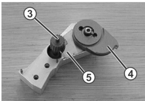
Fig. 5-25 Eléments du support de doigt
