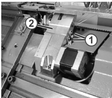
Fig. 5-24 Vis du support de doigt
