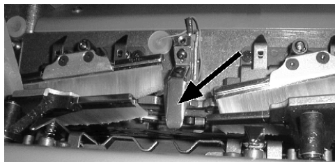
Fig. 6-34 Détecteur d'aiguilles
