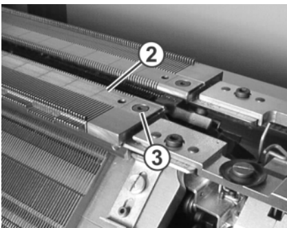
Fig. 6-10 Fonture supplémentaire
