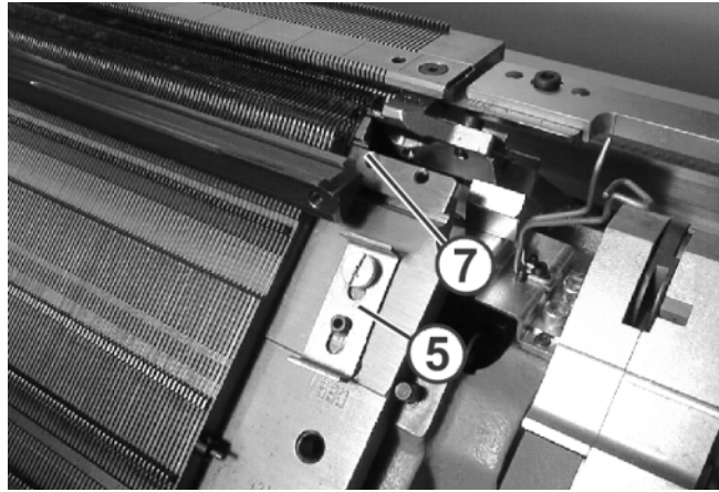
Fig. 6-13 Fil d'acier comme support de platine
