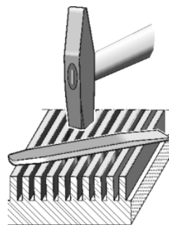
Fig. 6-24 Lisser la surface
