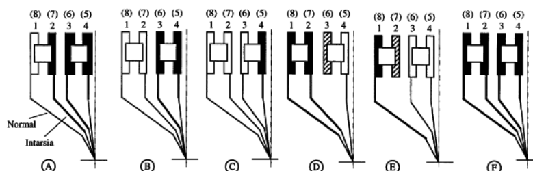
Fig. 6-54 Possibilités de combinaison pour guide-fil normaux et guide-fil d'intarsia
