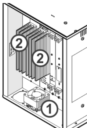
Fig. 5-16 Appareil de commande
