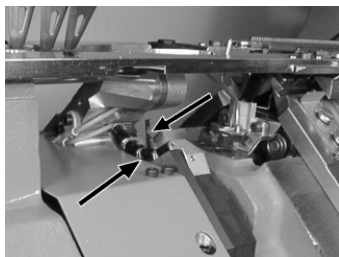
Fig. 5-19 Pignons de pinçage
