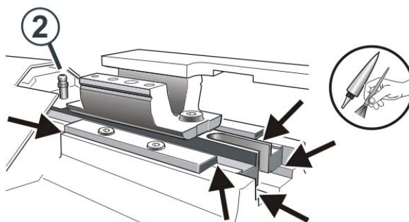
Fig. 5-47 Graisser le dispositif de chevalement des fontures auxiliaires
