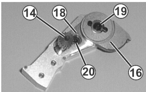
Fig. 5-34 Support de doigt
