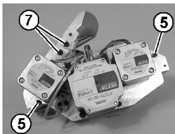
Fig. 5-29 Dispositif de pincage et de coupe
