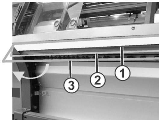
Fig. 2-38 Barre d'embrayage
