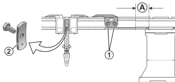
Fig. 6-53 Vis du limiteur de guide-fils
