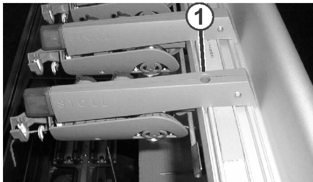
Fig. 6-58 Démontage d'un dispositif de contrôle du fil
