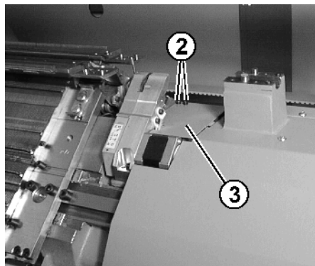
Fig. 6-49 Couvercle du dispositif de pinçage et de coupe du fil
