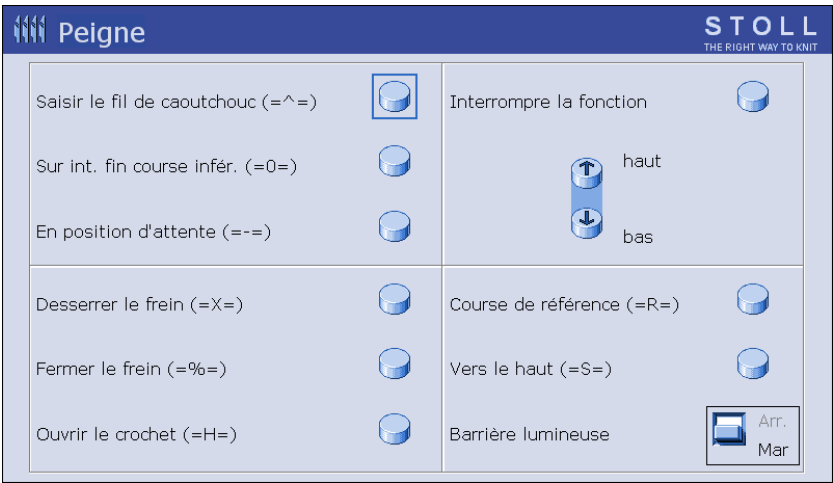
Fig. 4-18 Fenêtre "Peigne"
