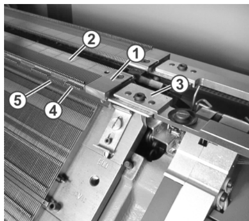
Fig. 2-28 Fonture supplémentaire
