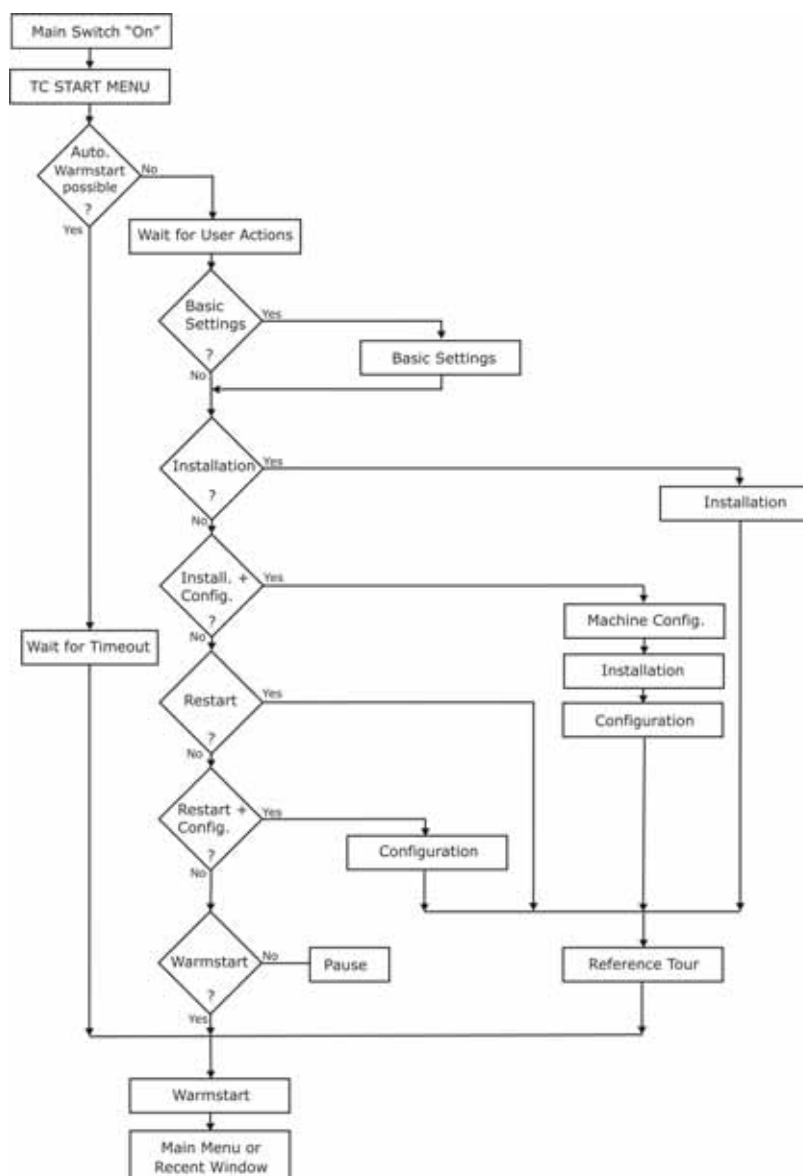
Fig. 7-1 Représentation schématique du processus de démarrage
