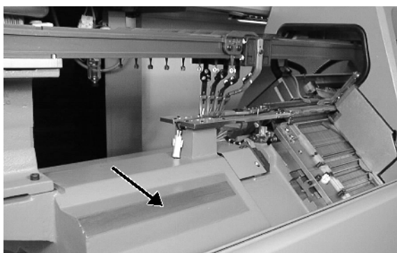
Fig. 6-39 Surface d'appui de gauche pour pièce de chariot
