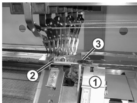
Fig. 4-8 Enfiler le fil
