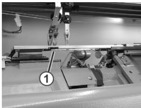
Fig. 2-22 Arrêt par chocs pour fontures supplémentaires
