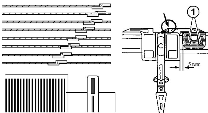
Fig. 4-68 Réglage des limiteurs de guide-fils
