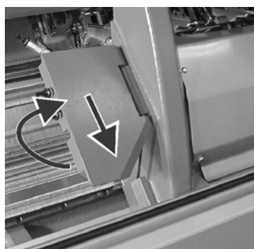
Fig. 6-2 Position de montage de la lubrification centrale
