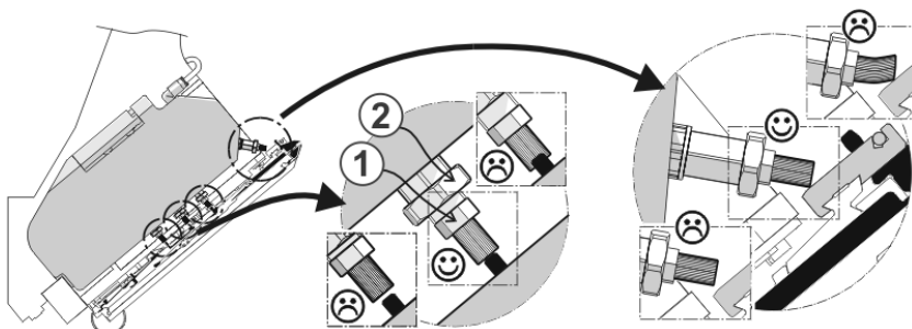
Fig. 4-70 Brosses de la lubrification centrale
