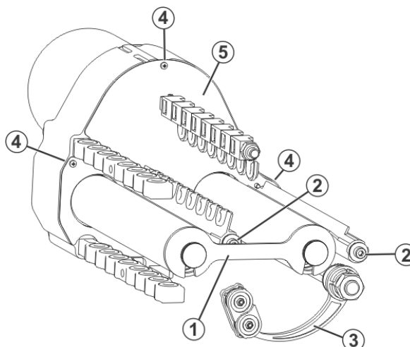
Fig. 6-59 Fournisseur à friction
