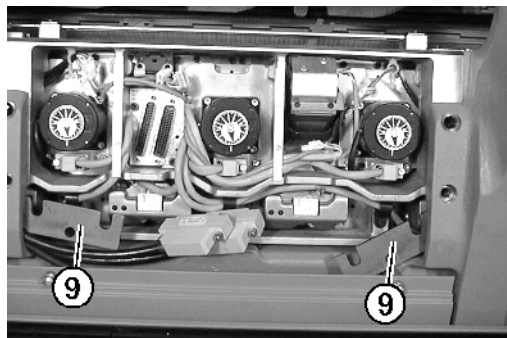
Fig. 6-31 plaque pivotante de gauche et de droite
