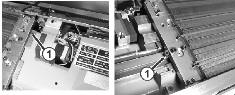
Fig. 6-20 Montage des fontures avant et arrière
