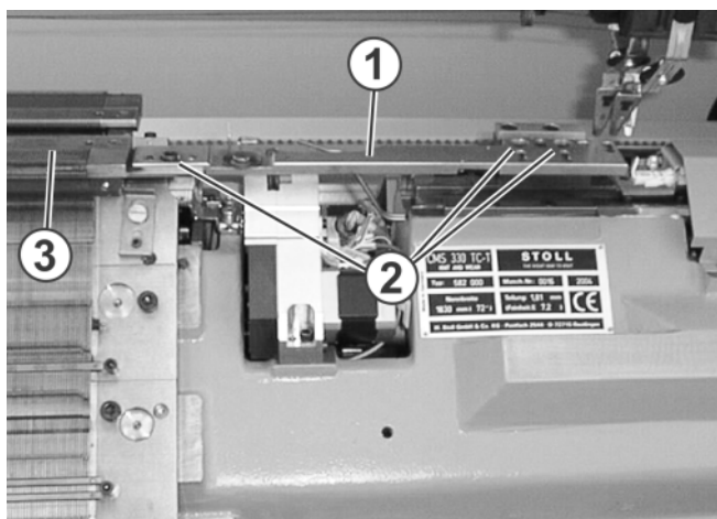
Fig. 6-19 Démontage des fontures supplémentaires
