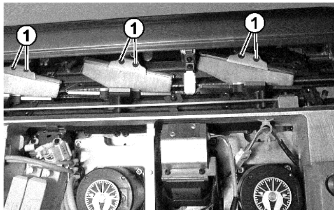
Fig. 4-71 Vis des brosses ouvre-clapets
