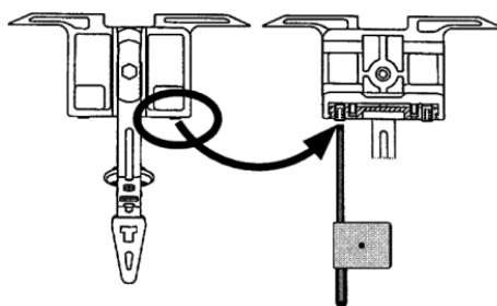
Fig. 4-69 Réglage du guidage du guide-fil
