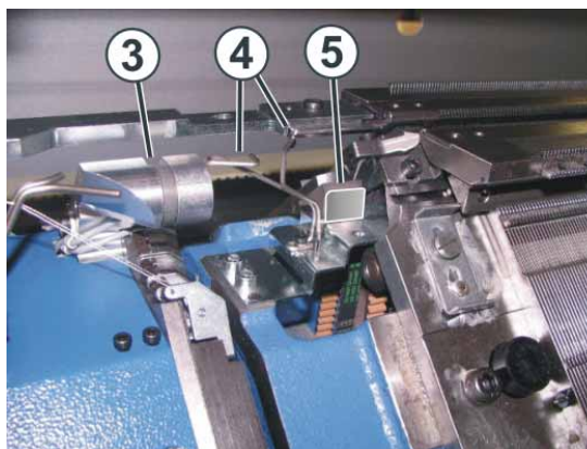
Fig. 2-10 Système de guidage du fil
