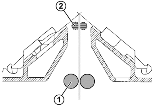
Fig. 2-34 Tirage auxiliaire
