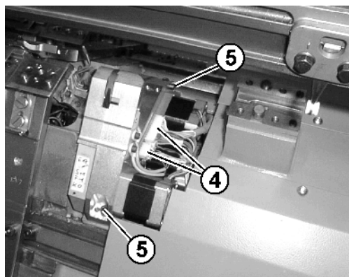
Fig. 6-50 Câble et vis du dispositif de pinçage et de coupe du fil
