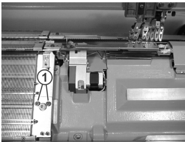
Fig. 6-17 Desserrer la fonture
