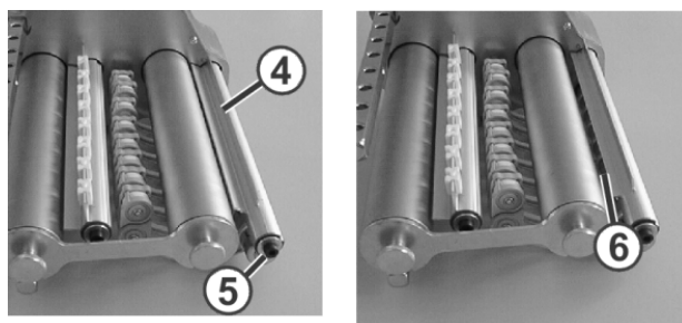
Fig. 4-12 Régler la distance entre le rail d'arrêt et le rouleau à friction.
