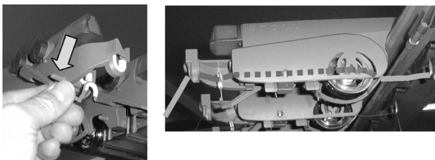
Fig. 3-11 Chemin du fil à travers le dispositif de contrôle du fil
