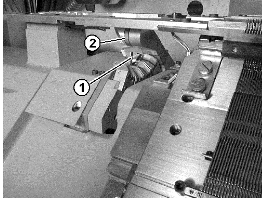
Fig. 2-9 Dispositif de pince et de coupe
