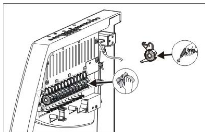
Fig. 5-11 Nettoyage du frein permanent
