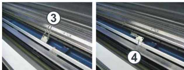
Fig. 6-16 Connexion du rail du générateur d'impulsions
