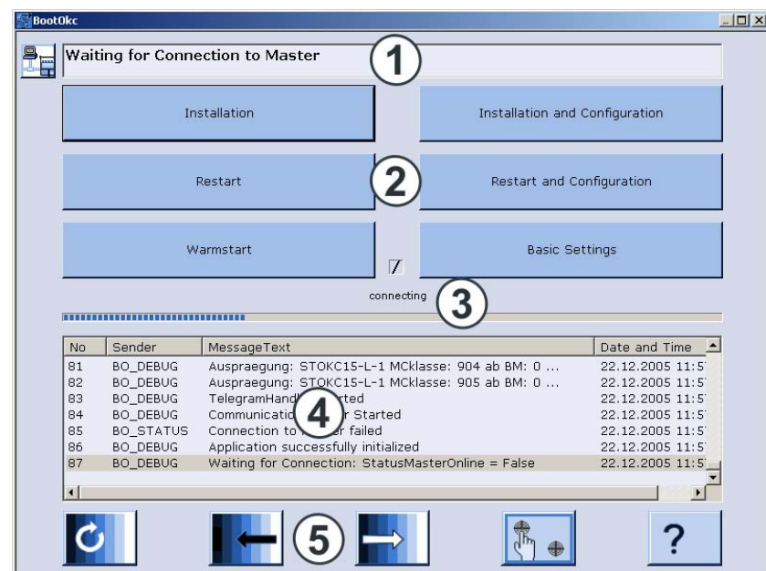
Fig. 7-3 Fenêtre "BootOkc"
