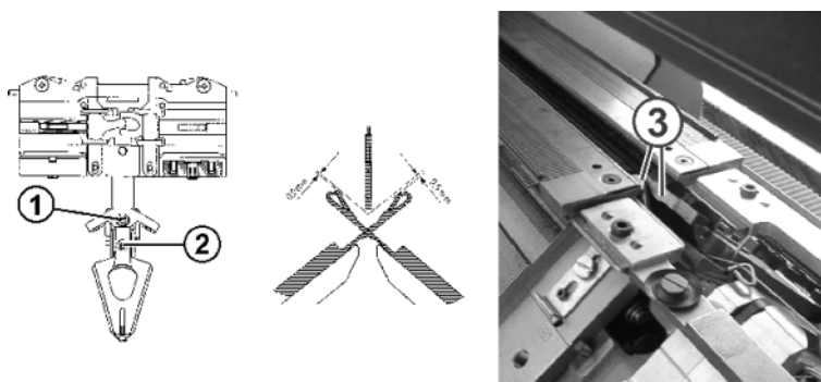
Fig. 4-72 Réglage des guide-fils intarsia
