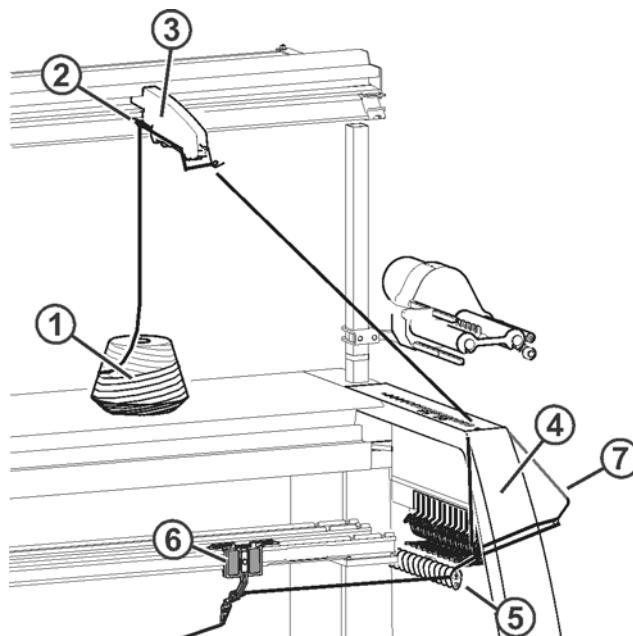
Fig. 2-2 Passage du fil 2
