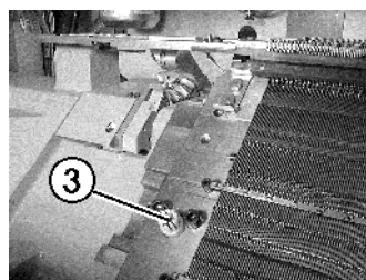
Fig. 2-16 Brosses de nettoyage des systèmes de sélection
