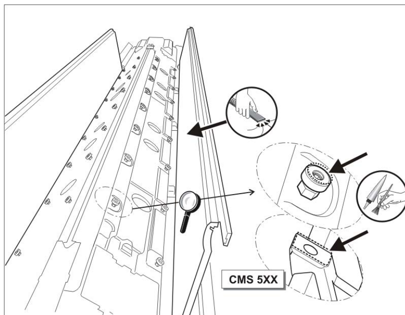
Fig. 5-50 Graissage des pièces d'ajustage
