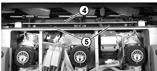
Fig. 6-29 Démontage de la came supplémentaire
