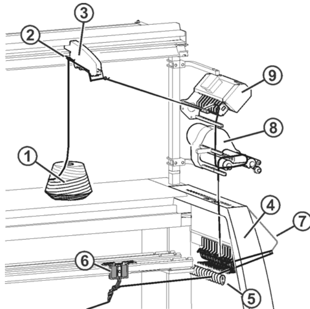
Fig. 2-4 Passage du fil 4
