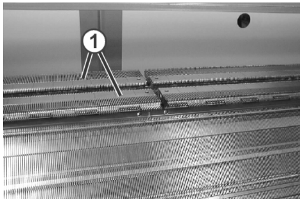
Fig. 2-27 Fontures supplémentaires divisées
