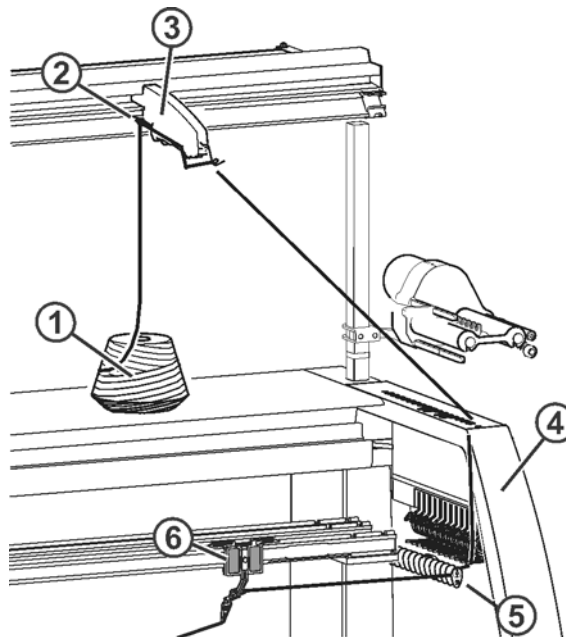
Fig. 2-1 Passage du fil 1
