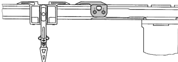
Fig. 6-55 Limiteur des guide-fils et renvoi du fil
