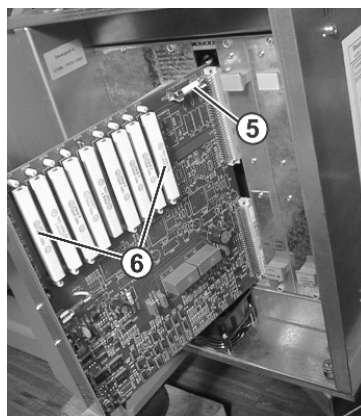
Fig. 6-68 Coupe-circuit de charge (5) pour servocommande et chevalement à l'appareil de commande de droite
