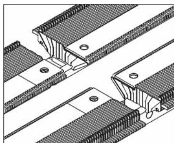
Fig. 5-14 Nettoyer la jonction
