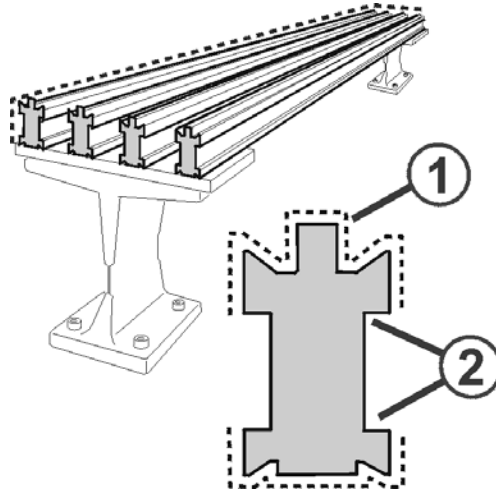
Fig. 5-45 Graissage des barres de guide-fils
