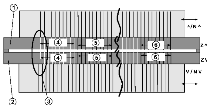
Fig. 4-55 Position de base des fontures par rapport aux fontures supplémentaires
