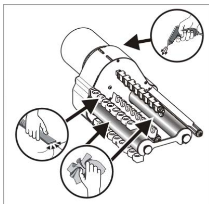
Fig. 5-12 Nettoyage du fournisseur à friction
