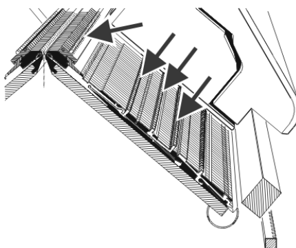
Fig. 2-16 Points de lubrification de la lubrification centrale
