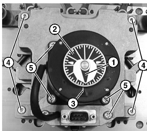
Fig. 6-33 Démontage du moteur pas à pas
