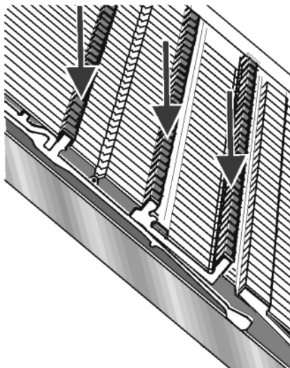
Fig. 5-26 Graissage des talons de la pièce d'accouplement et du verrou intermédiaire
