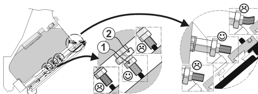
Fig. 4-63 Brosses de la lubrification centrale
