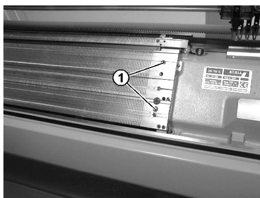
Fig. 6-12 Desserrer la fonture
