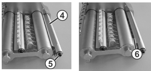
Fig. 4-10 Régler la distance entre le rail d'arrêt et le rouleau à friction.
