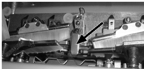
Fig. 6-25 Détecteur d'aiguilles
