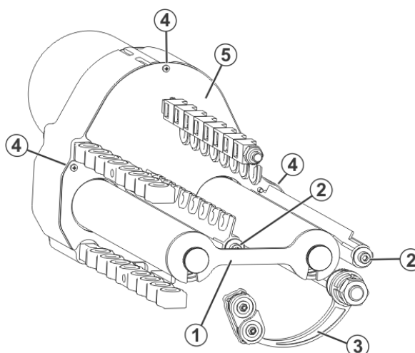
Fig. 6-44 Fournisseur à friction
