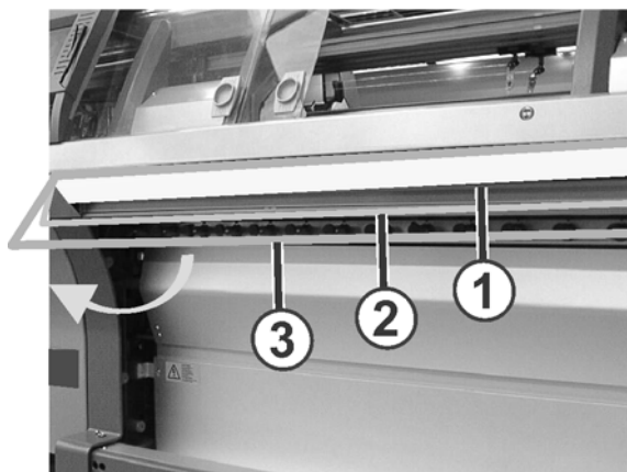
Fig. 2-29 Barre d'embrayage
