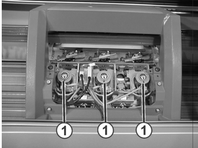
Fig. 2-21 Moteur pas à pas de réglage de la serre des mailles
