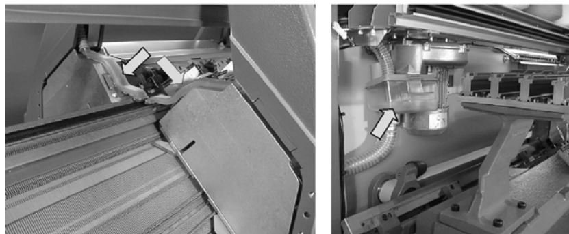
Fig. 2-13 Elimination de la peluche et récipient à peluches (modèle 000)
