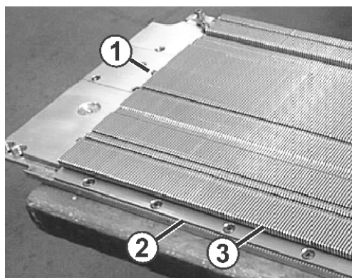
Fig. 6-19 Réparation d'une fonture assemblée
