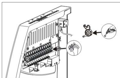
Fig. 5-10 Nettoyage du frein permanent
