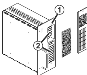
Fig. 5-14 Bloc d'alimentation du ventilateur
