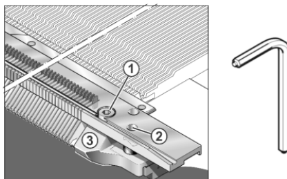
Fig. 6-8 Démontage du limiteur(3)
