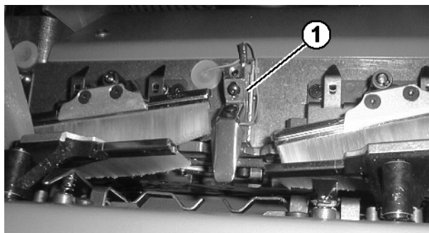
Fig. 2-23 Détecteur d'aiguilles
