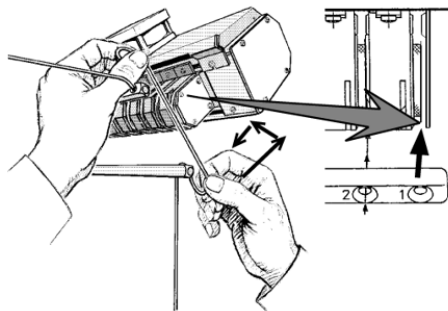
Fig. 3-13 Chemin du fil dans l'appareil STIXX
