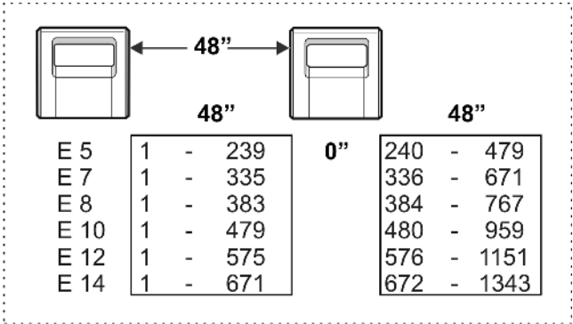
Fig. 4-54 Zone d'aiguilles largeur de couplage 48"
