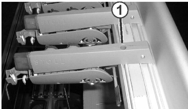
Fig. 6-43 Démontage d'un dispositif de contrôle du fil
