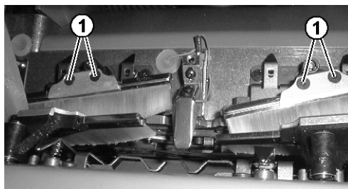
Fig. 4-64 Vis des brosses ouvre-clapets
