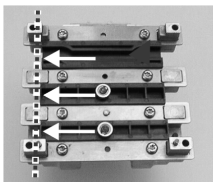
Fig. 6-37 Contrôle de la position de montage
