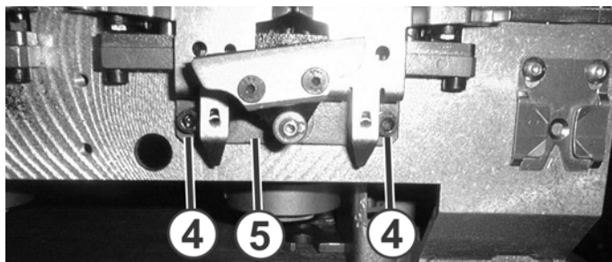
Fig. 6-32 Commande des platines d'appui
