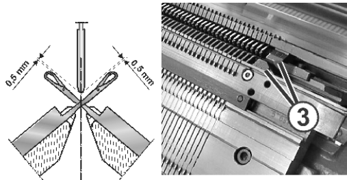
Fig. 4-61 Réglage des guide-fils
