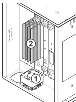
Fig. 5-13 Appareil de commande
