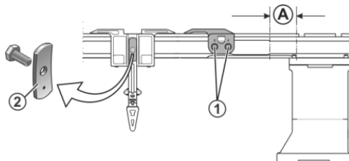
Fig. 6-38 Vis du limiteur de guide-fils
