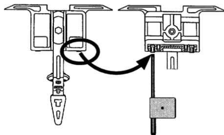
Fig. 4-62 Réglage du guidage du guide-fil
