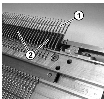
Fig. 5-8 Nettoyage de la fonture
