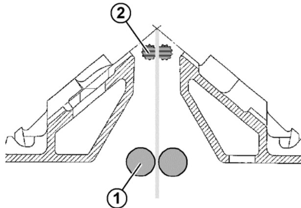
Fig. 2-27 Tirage auxiliaire
