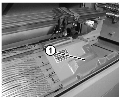
Fig. 6-28 Surface d'appui de la pièce de chariot
