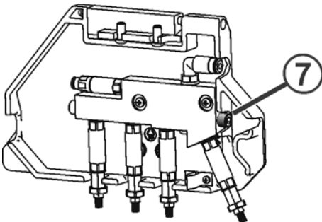
Fig. 6-48 Désaérer la lubrification centrale
