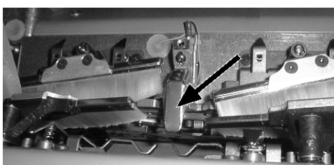
Fig. 6-21 Détecteur d'aiguilles
