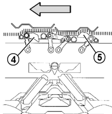
Fig. 2-20 Verrou des platines
