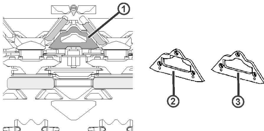
Fig. 2-18 Cames d'ascension
