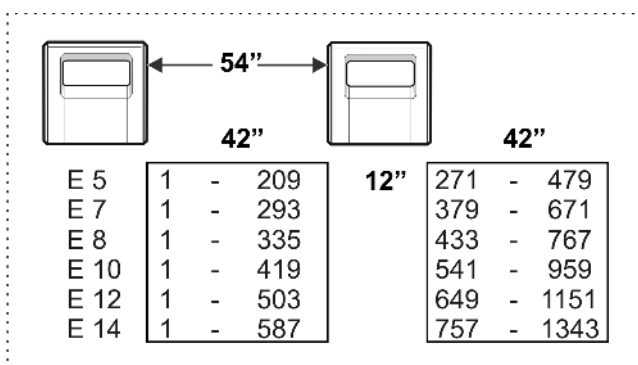
Fig. 4-51 Zone d'aiguilles largeur de couplage 54"
