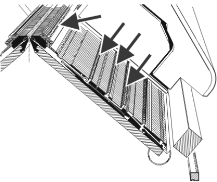
Fig. 5-18 Points de lubrification de la lubrification centrale
