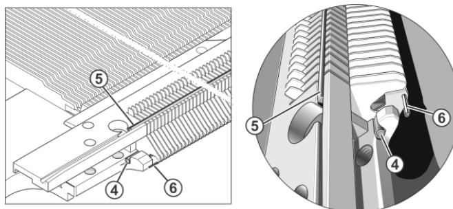
Fig. 6-9 Remplacement d'une platine
