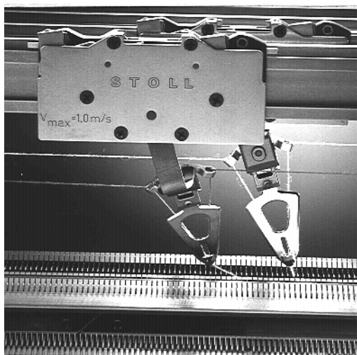
Fig. 2-9 Guide-fils intarsia
