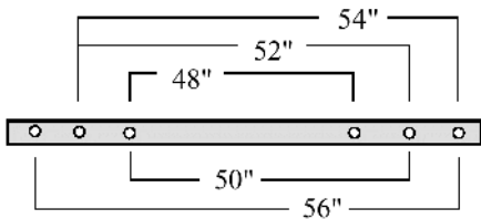
Fig. 4-48 Largeurs de couplage pour la CMS 933
