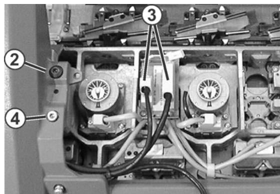
Fig. 6-23 Chariot ouvert
