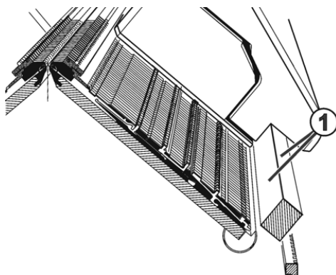
Fig. 5-24 Huilage de la barre de guidage du chariot
