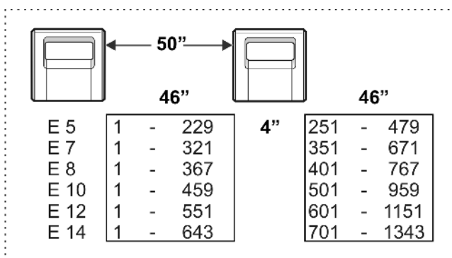
Fig. 4-53 Zone d'aiguilles largeur de couplage 50"
