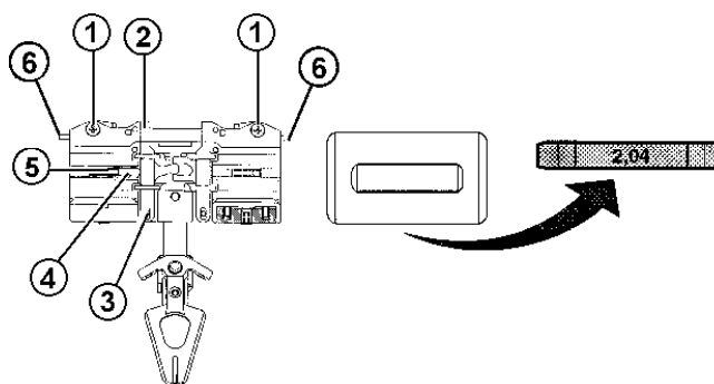
Fig. 4-67 Démontage de la plaquette de pression
