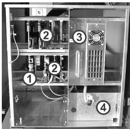
Fig. 6-49 Armoire de commande de gauche
