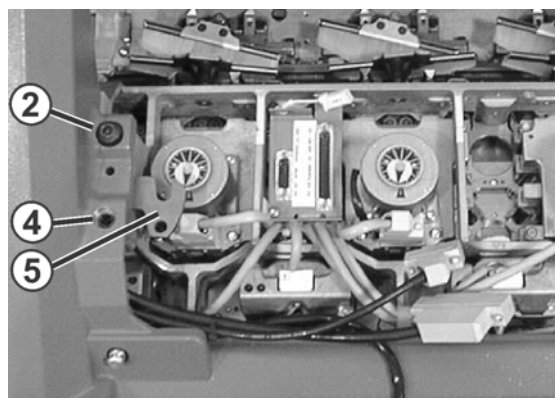
Fig. 6-26 Plaque pivotante
