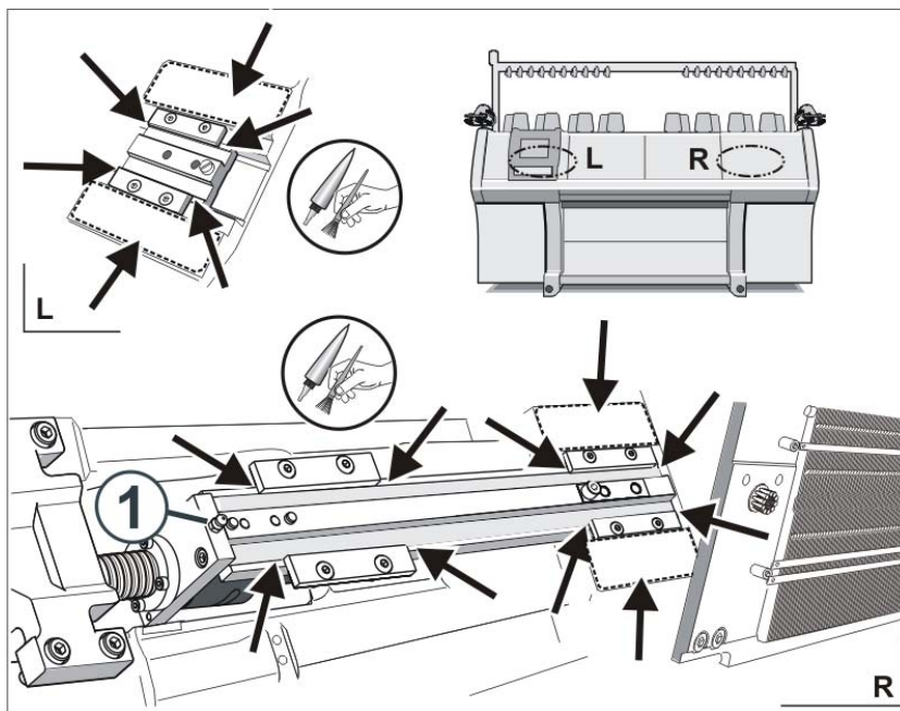
Fig. 5-29 Graisser le dispositif de chevalement
