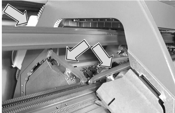
Fig. 2-12 Elimination de la peluche et récipient à peluches (à partir du modèle 001)
