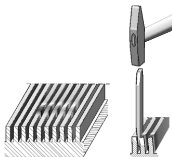
Fig. 6-16 Mettre les entretoises à la verticale
