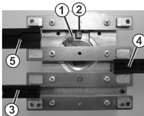
Fig. 6-36 Position de montage
