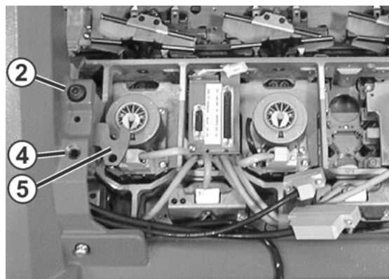
Fig. 6-22 Plaque pivotante
