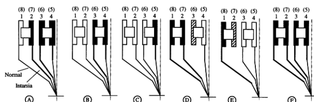
Fig. 6-39 Possibilités de combinaison pour guide-fil normaux et guide-fil d'intarsia
