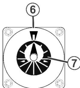
Fig. 6-34 Position de base du moteur pas à pas
