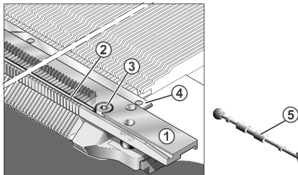
Fig. 5-15 Nettoyage approfondi de la fonture
