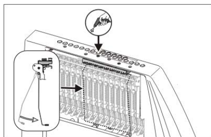
Fig. 5-9 Nettoyage du pince-fil actif
