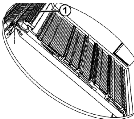
Fig. 5-22 Huilage de la fonture des platines
