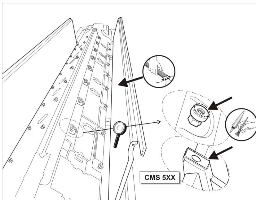
Fig. 5-30 Graissage des supports des fontures
