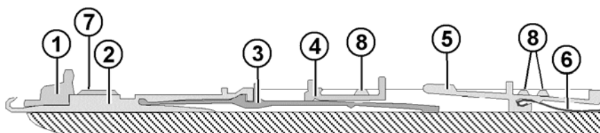
Fig. 2-24 Fonture
