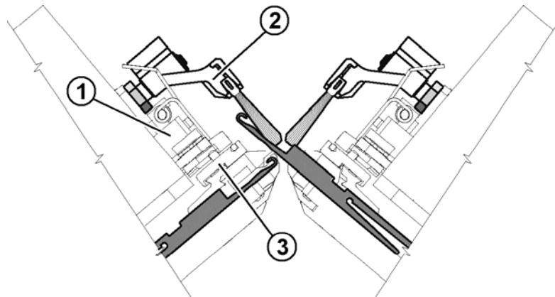
Fig. 2-19 Unité de commande des platines
