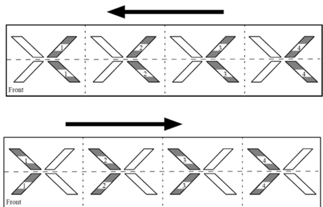
Fig. 4-43 Numérotation des cames de chute pour une machine à 4 systèmes
