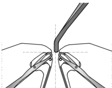
Fig. 4-59 Réglage du détecteur d'aiguilles
