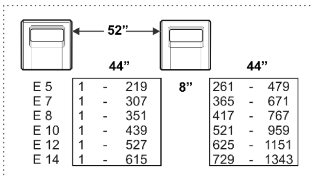
Fig. 4-52 Zone d'aiguilles largeur de couplage 52"
