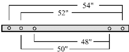
Fig. 4-47 Largeurs de couplage pour la CMS 922
