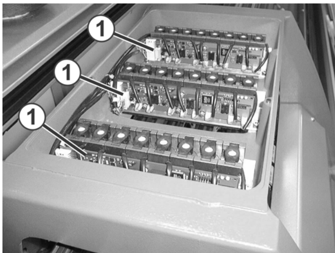
Fig. 6-52 Carte électronique pour commander les aimants des guide-fils
