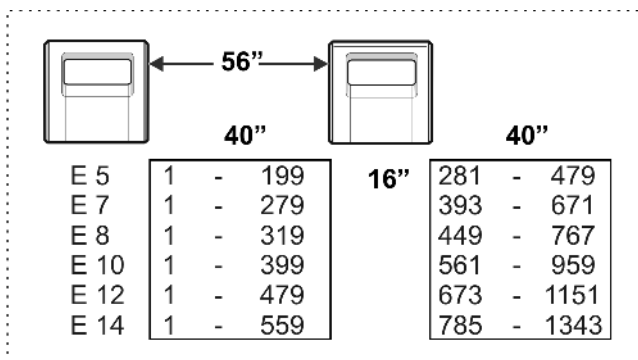
Fig. 4-50 Zone d'aiguilles largeur de couplage 56"
