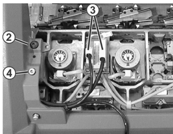
Fig. 6-27 Chariot ouvert
