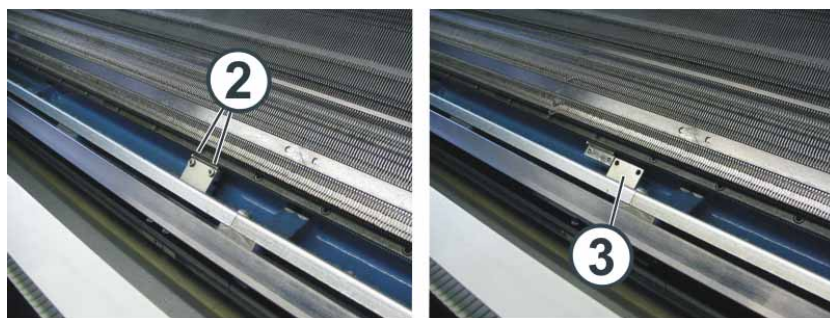
Fig. 6-13 Connexion du rail du générateur d'impulsions
