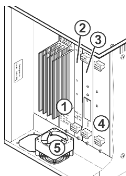
Fig. 6-50 Armoire de commande de droite
