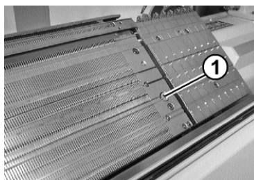
Fig. 2-14 Brosses de nettoyage des systèmes de sélection
