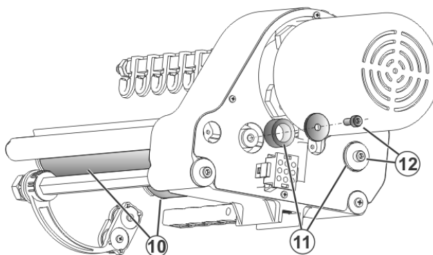
Fig. 6-46 Vis pour rouleaux à friction
