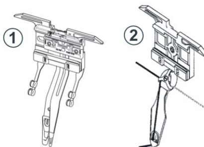
Fig. 2-10 Guide-fil à vaniser
