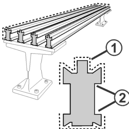
Fig. 5-23 Huilage des barres de guide-fils
