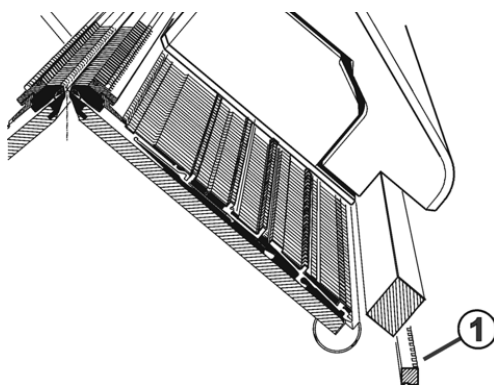
Fig. 5-25 Graissage des rails du générateur d'impulsions
