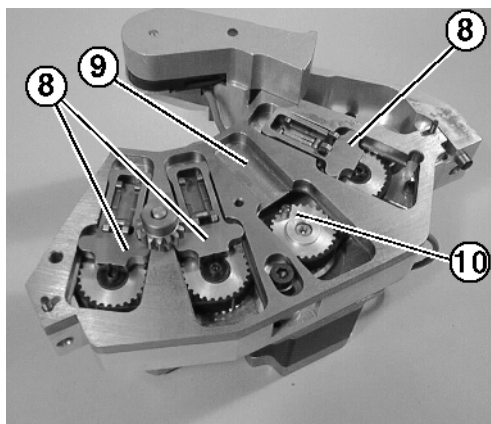
Fig. 5-25 Boîte de manivelle
