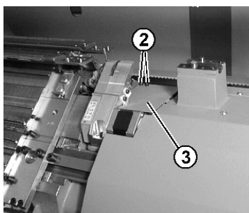
Fig. 6-38 Couvercle du dispositif de pince et de coupe du fil
