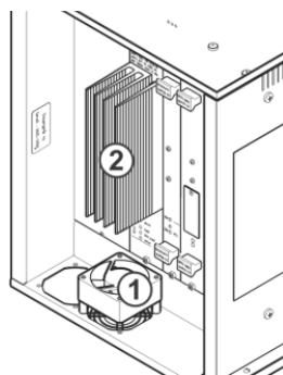
Fig. 5-13 Appareil de commande
