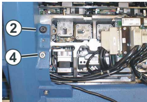
Fig. 6-26 Chariot ouvert
