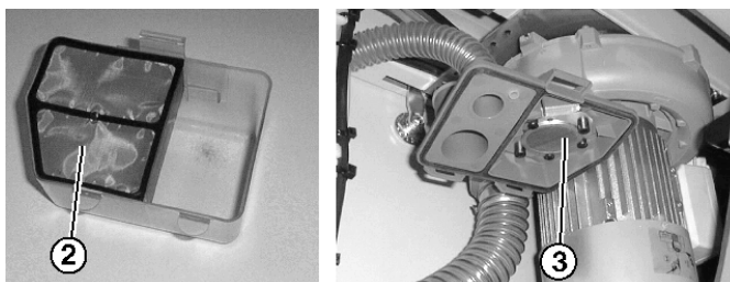
Fig. 5-5 Récipient à peluches et filtre
