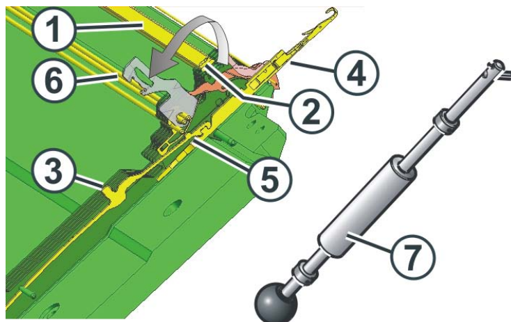
Fig. 6-5 Remplacement de l'aiguille et de la pièce d'accouplement
