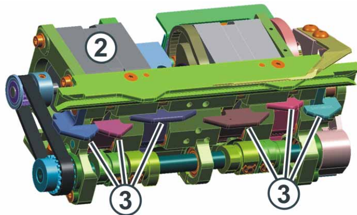
Fig. 2-22 Commande de la platine d'appui
