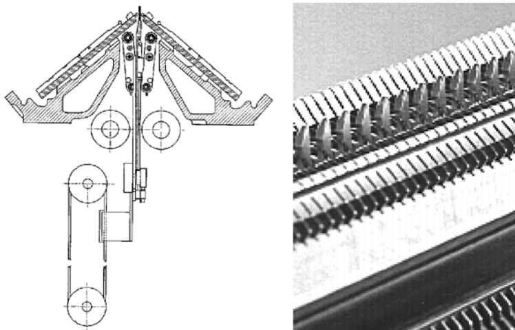
Fig. 2-30 Tirage du peigne
