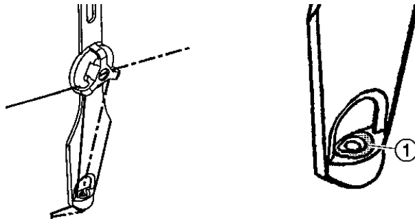
Fig. 4-64 Trou allongé du guide-fil à vaniser
