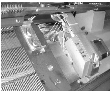
Fig. 5-20 Tendre la courroie à crans dans la direction de la flèche
