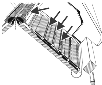
Fig. 5-30 Points de lubrification de la lubrification centrale
