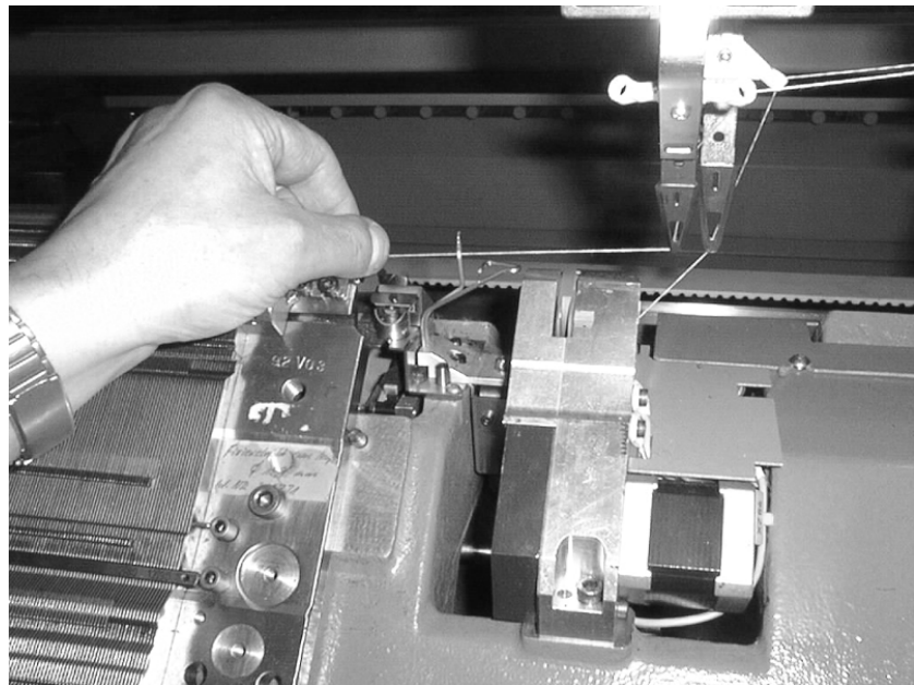
Fig. 3-16 Enfiler le fil
