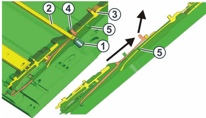
Fig. 6-7 Remplacement du verrou intermédiaire
