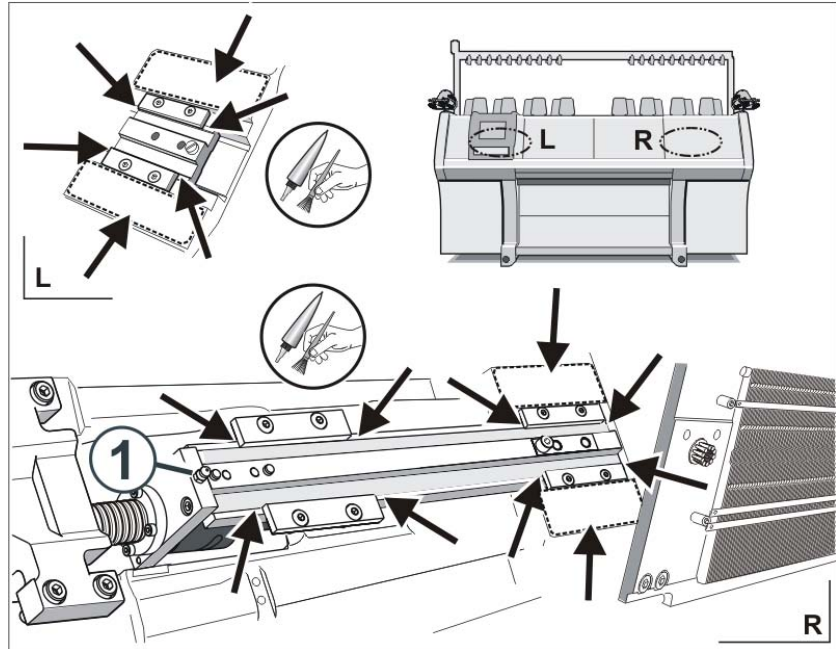
Fig. 5-41 Graisser le dispositif de chevalement
