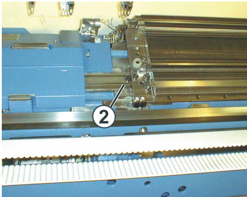
Fig. 6-19 Montage de la fonture arrière
