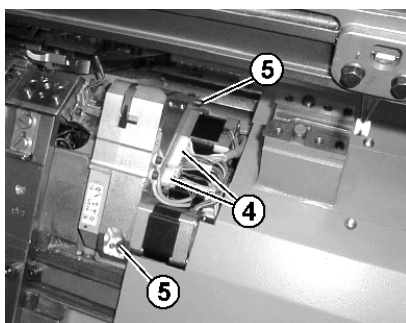
Fig. 6-39 Câble et vis du dispositif de pince et de coupe du fil
