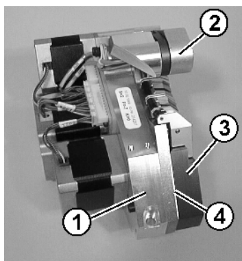
Fig. 5-21 Boîtier de l'unité de pinçage et de coupe
