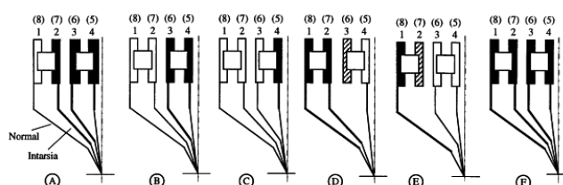
Fig. 6-43 Possibilités de combinaison pour guide-fil normaux et guide-fil d'intarsia
