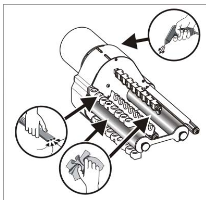
Fig. 5-11 Nettoyage du fournisseur à friction
