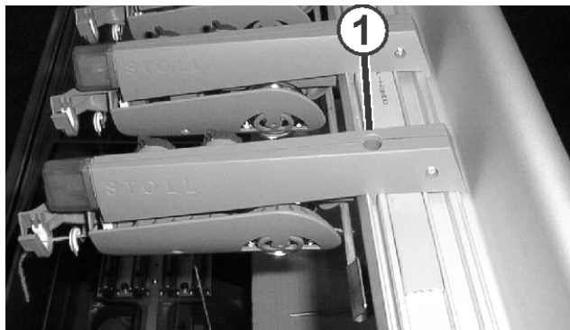
Fig. 6-47 Démontage d'un dispositif de contrôle du fil
