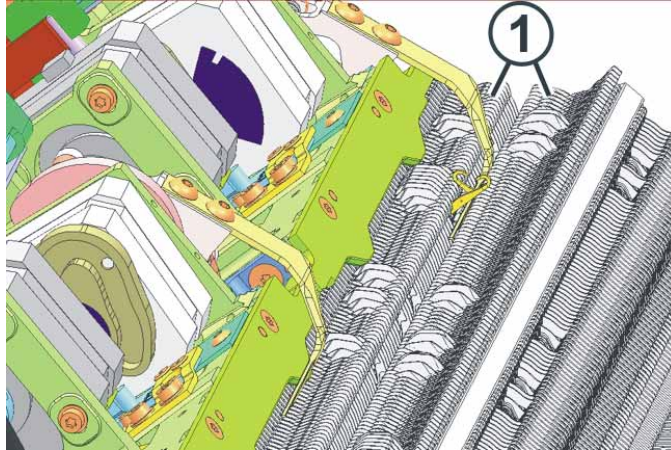
Fig. 2-21 Platines d'appui
