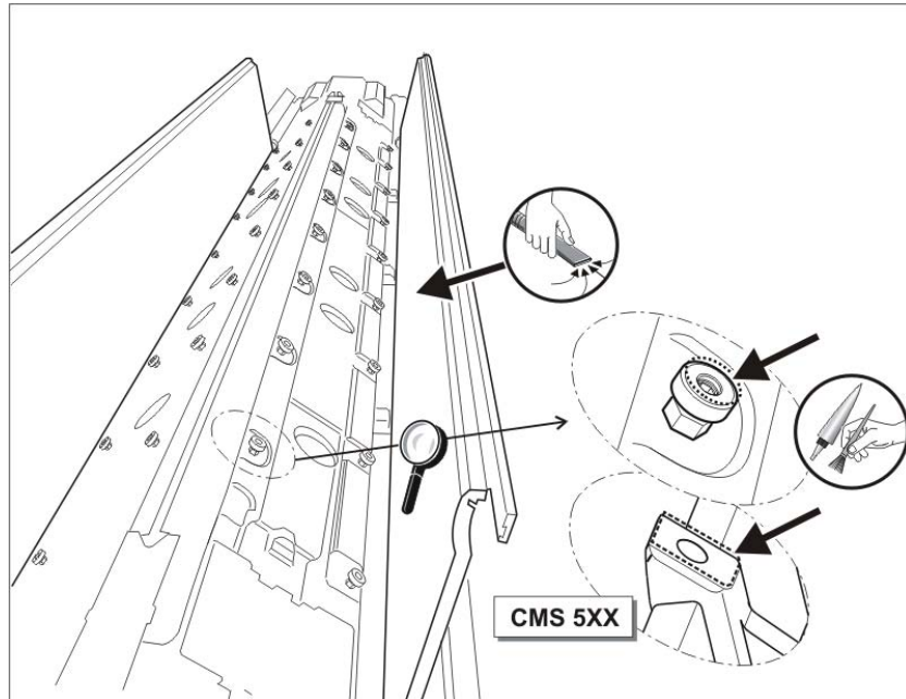
Fig. 5-42 Graissage des pièces d'ajustage
