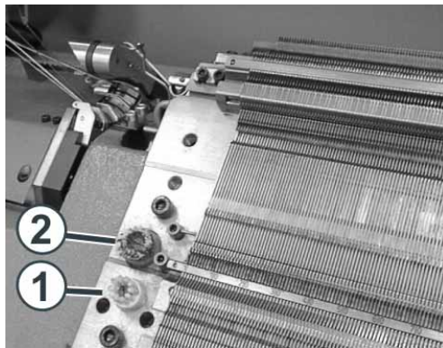
Fig. 2-15 Brosses de nettoyage des systèmes de sélection Après un nombre programmable de rangées de tricotage, le chariot effectue une course de nettoyage sur l'ensemble de la fonture, au cours de laquelle les peluches sont aspirées de la fonture. Des brosses sont fixées extérieurement à la fonture.
