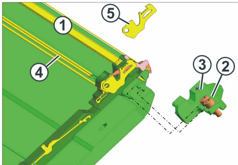
Fig. 6-12 Remplacement d'un guidage des aiguilles
