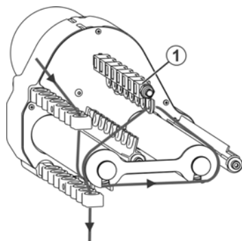
Fig. 4-9 Réglage de l'approvisionnement en fil du fournisseur à friction
