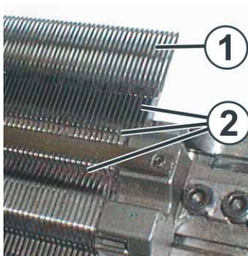
Fig. 5-8 Nettoyage de la fonture
