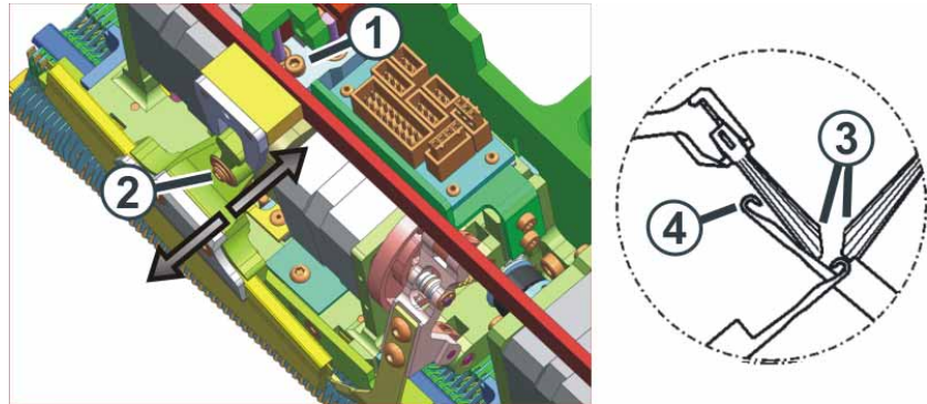
Fig. 4-48 Inclinaison des brosses ouvre-clapets
