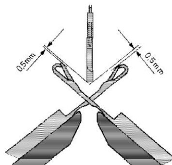
Fig. 4-56 Réglage des guide-fils
