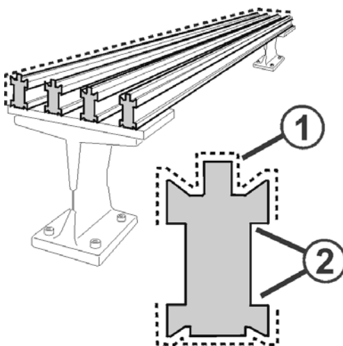
Fig. 5-35 Huilage des barres de guide-fils
