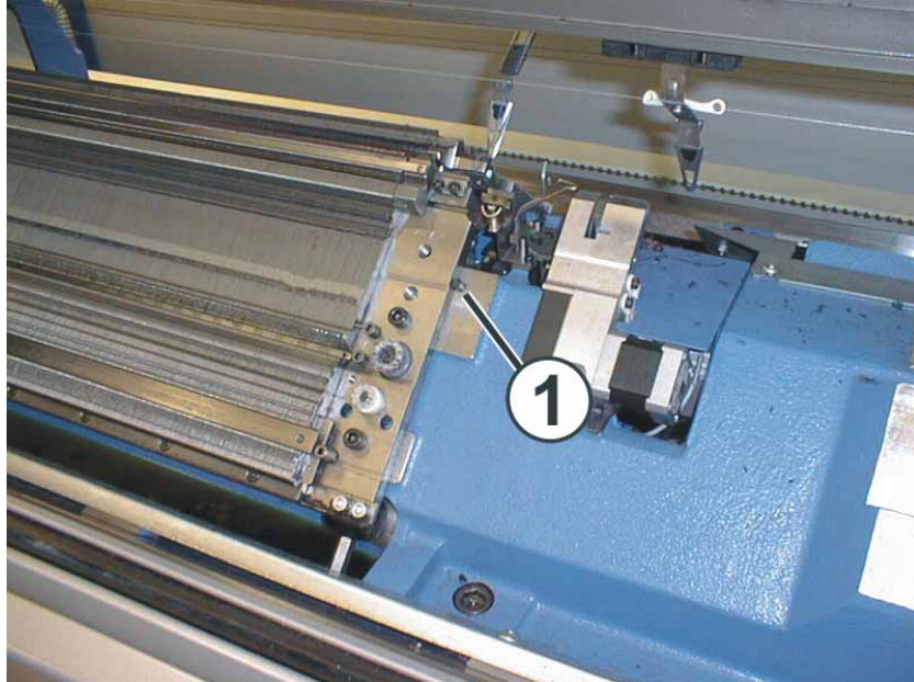
Fig. 6-18 Montage de la fonture avant
