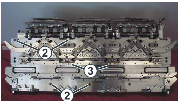
Fig. 6-36 Vis du corps en fonte au plateau porte-cames
