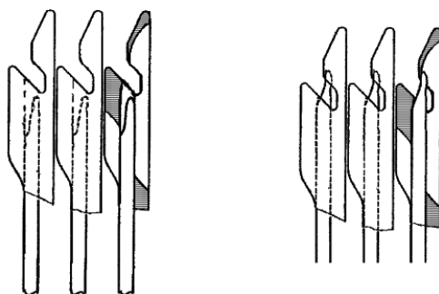
Fig. 2-31 Crochet du peigne du tirage du peigne avec coulisses (en position ouverte à gauche, en position fermée à droite)
