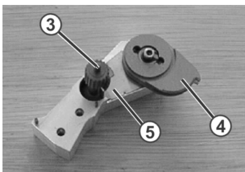
Fig. 5-18 Éléments du support de doigt
