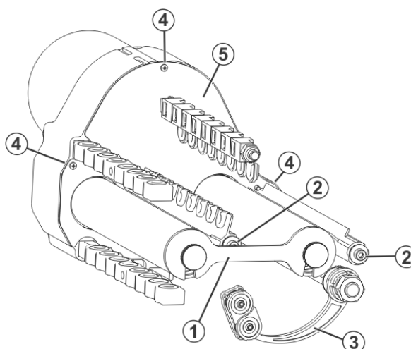
Fig. 6-48 Fournisseur à friction
