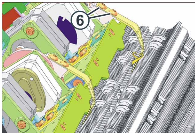
Fig. 6-30 Presse-maillages actif
