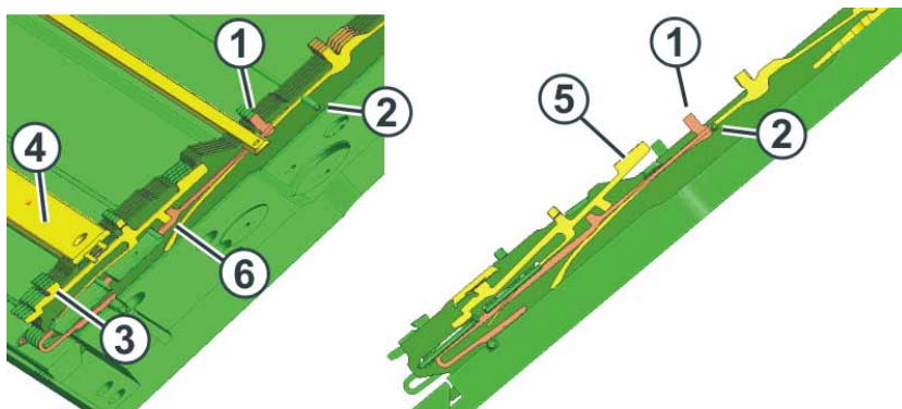
Fig. 6-8 Remplacement de la platine de sélection
