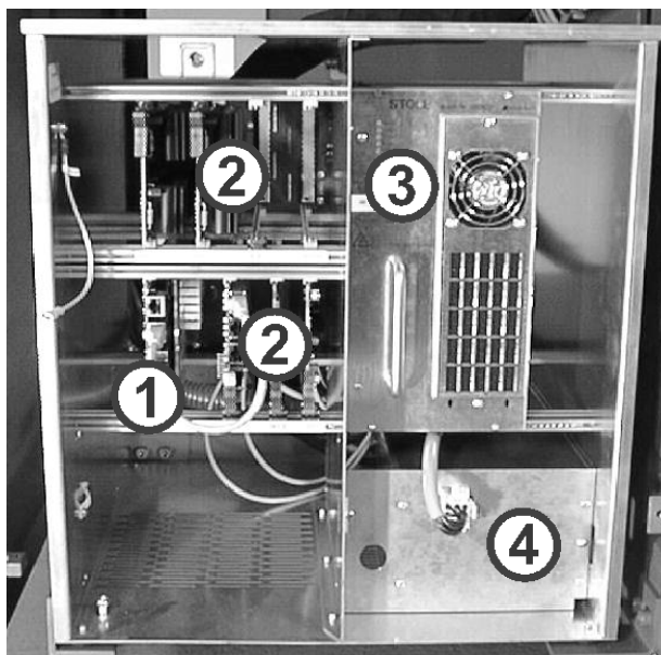
Fig. 6-53 Armoire de commande de gauche
