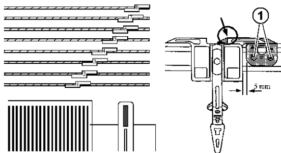
Fig. 4-57 Réglage des limiteurs de guide-fils
