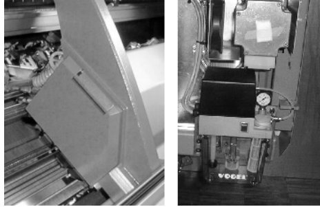
Fig. 2-16 Lubrification centrale au chariot, à droite: Alimentation en huile Elle lubrifie à l'huile les talons de travail des platines d'appui, de la pièce d'accouplement et du verrou intermédiaire. Tous les autres points de lubrification doivent être graissés manuellement.
