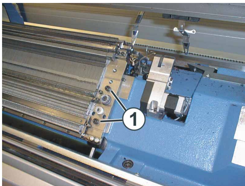
Fig. 6-14 Desserrer la fonture
