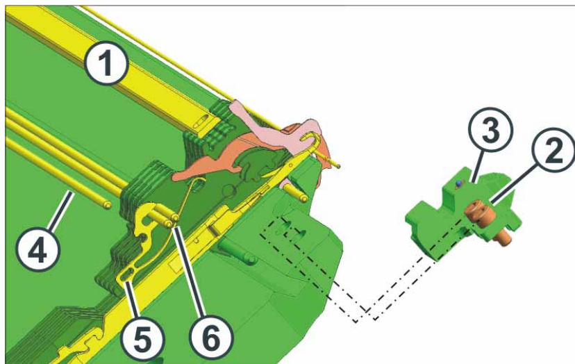
Fig. 6-10 Remplacement d'un ressort de la platine d'appui
