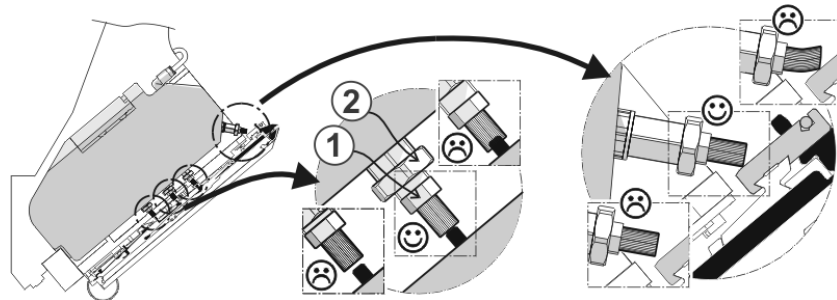
Fig. 4-59 Brosses de la lubrification centrale
