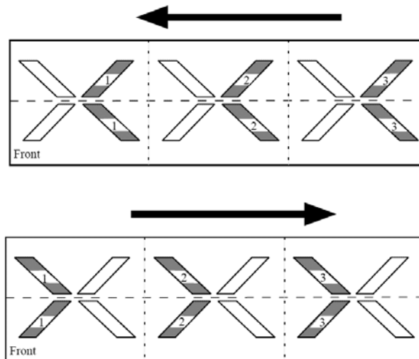
Fig. 4-47 Numérotation des cames de chute pour une machine à 3 systèmes
