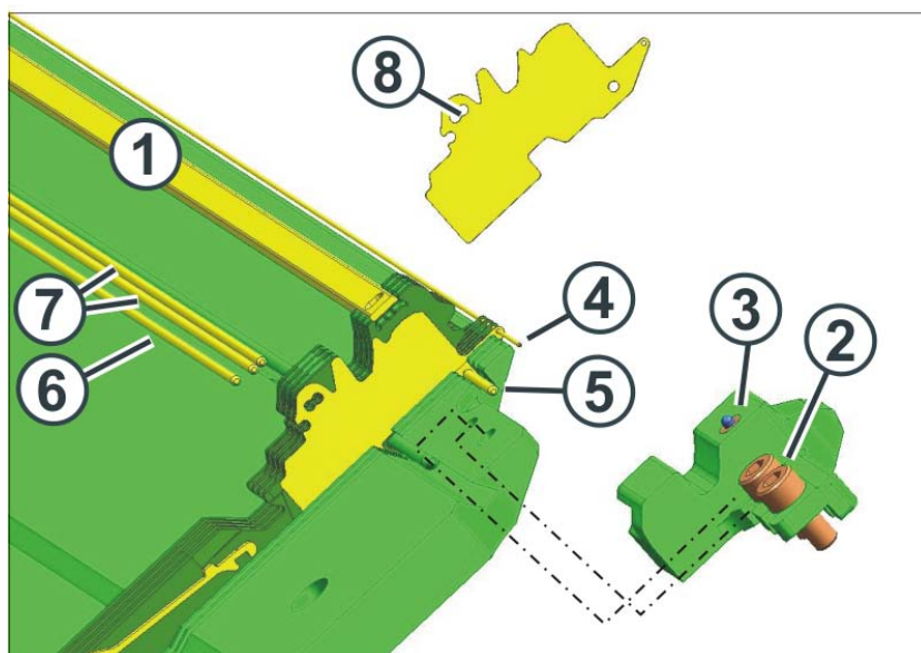
Fig. 6-13 Remplacement d'un support du fil métallique
