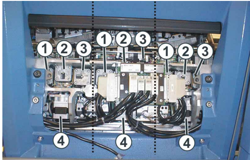
Fig. 2-20 Moteurs pas à pas dans le chariot
