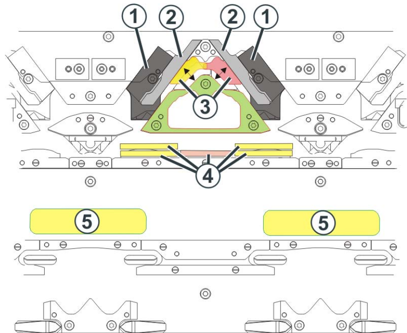
Fig. 2-19 Chute de tricotage
