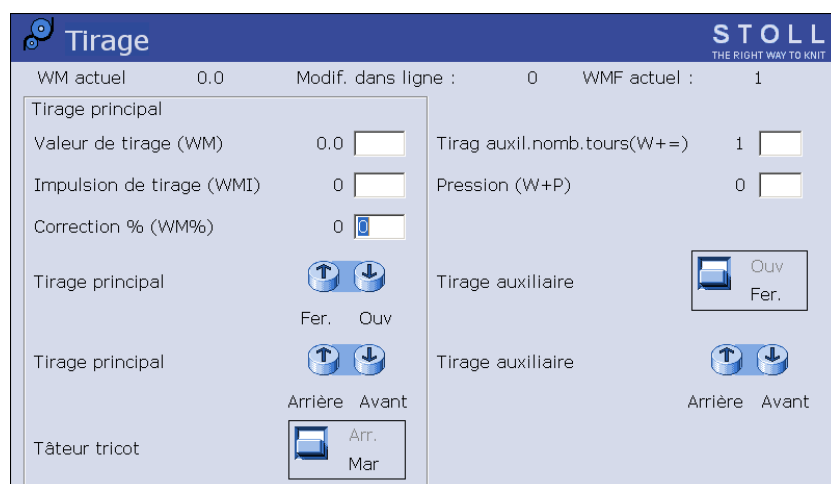
Fig. 4-14 Fenêtre "Tirage"
