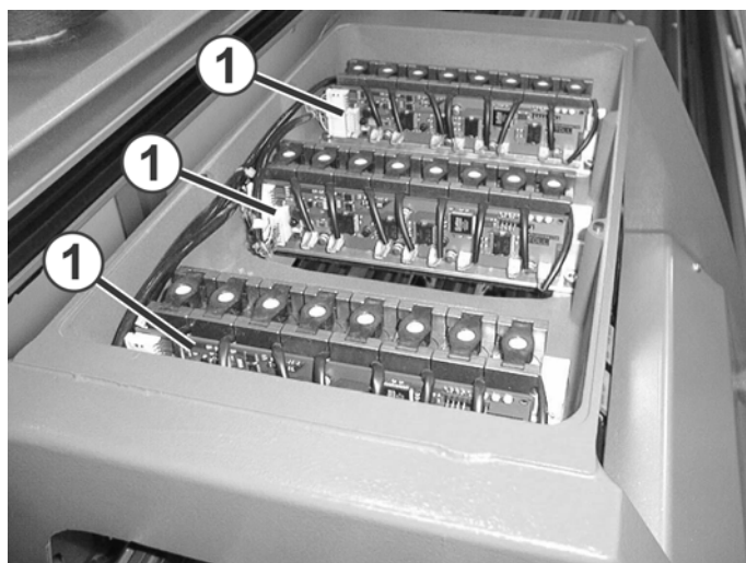
Fig. 6-56 Carte électronique pour commander les aimants des guide-fils
