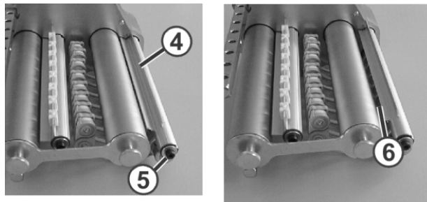
Fig. 4-11 Régler la distance entre le rail d'arrêt et le rouleau à friction.
