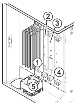
Fig. 6-54 Armoire de commande de droite
