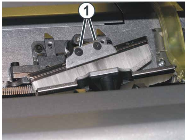
Fig. 4-55 Vis des brosses ouvre-clapets
