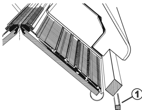
Fig. 5-37 Graissage des rails du générateur d'impulsions
