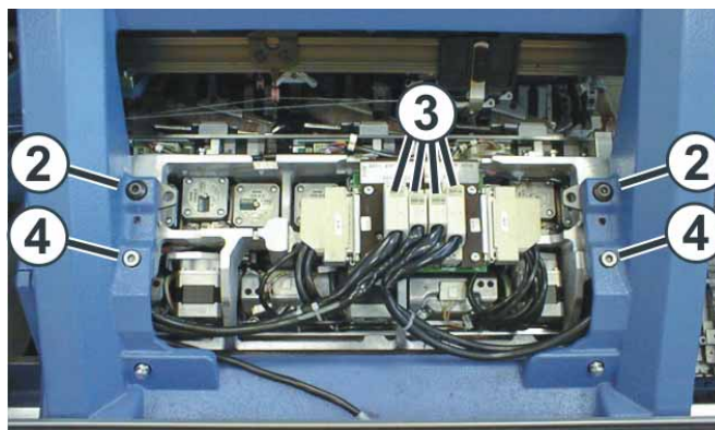
Fig. 6-34 Fixation du chariot à la pièce de chariot
