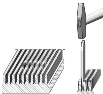
Fig. 6-21 Mettre les entretoises à la verticale
