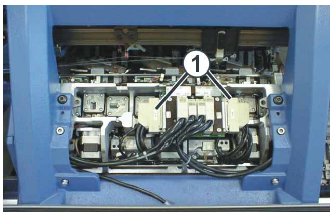
Fig. 6-35 Fiches (moteurs pas à pas, systèmes de sélection)
