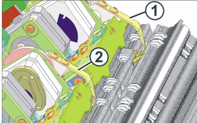
Fig. 2-18 Presseur avec moteur pas à pas
