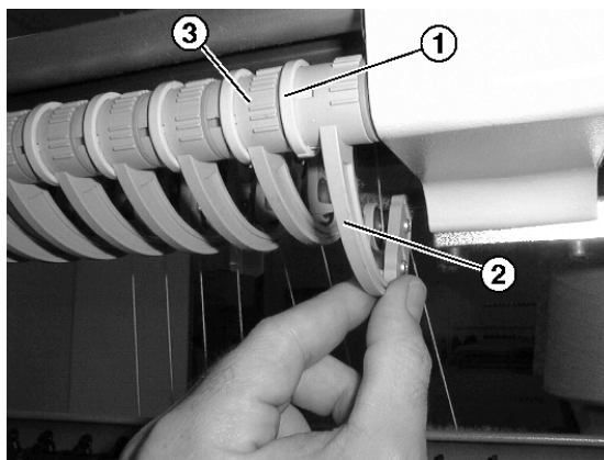
Fig. 4-10 Réglage de l'approvisionnement en fil du fournisseur à friction
