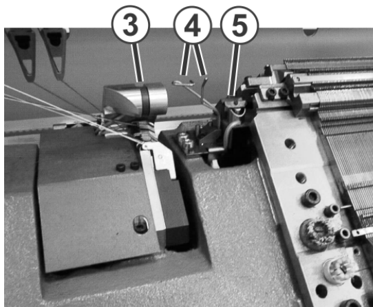
Fig. 2-10 Système de guidage du fil
