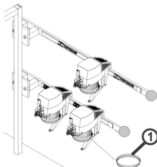
Fig. 4-12 Fournisseur à accumulation SFE
