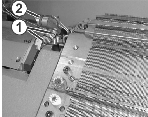
Fig. 2-9 Dispositif de pince et de coupe
