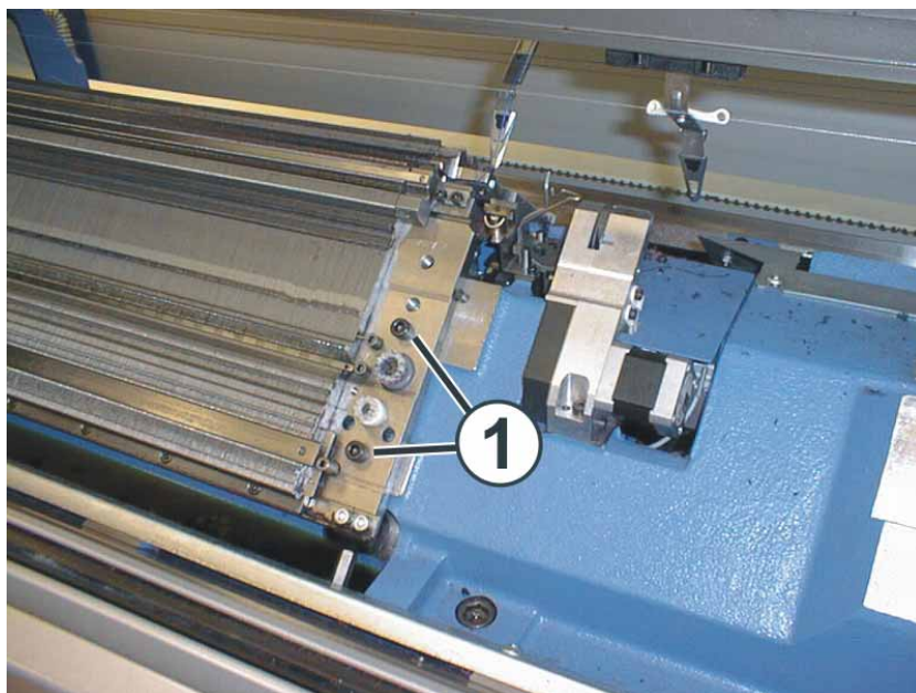
Fig. 6-16 Desserrer la fonture
