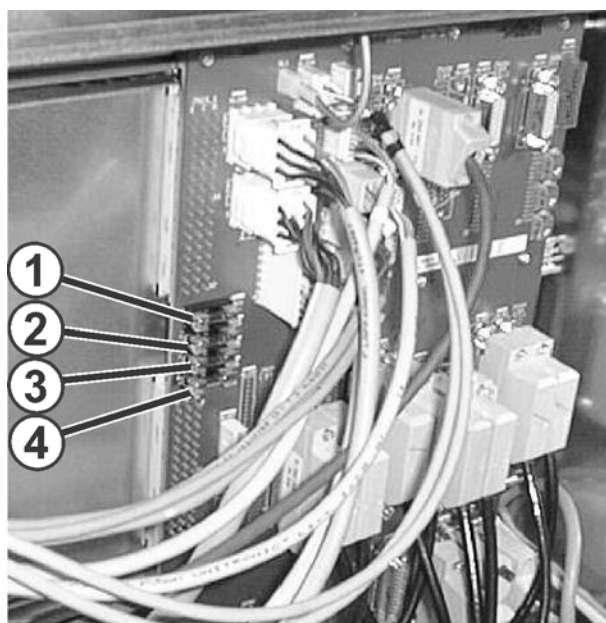
Fig. 6-57 Coupe-circuit à l'arrière de l'appareil de commande de gauche
