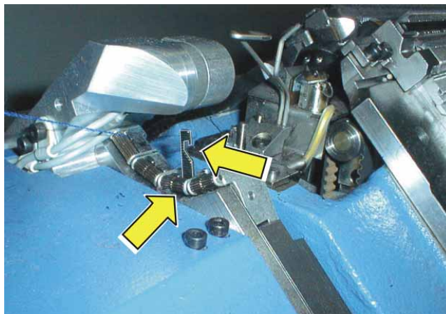
Fig. 5-16 Aiguilles de pince et de coupe et pignons de pince
