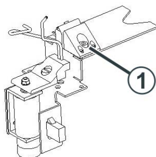
Fig. 4-49 Réglage de la pince-fil
