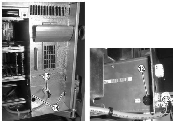
Fig. 6-58 Fusible de la batterie (12) en dessous du bloc d'alimentation
