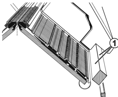
Fig. 5-36 Huilage de la barre de guidage du chariot
