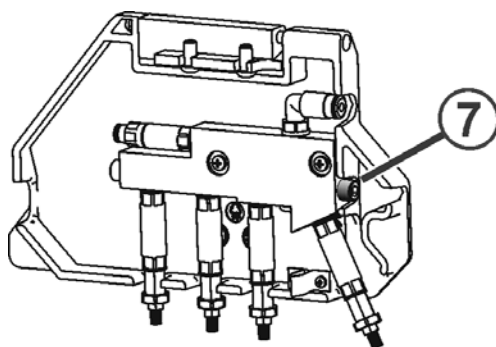
Fig. 6-52 Désaérer la lubrification centrale
