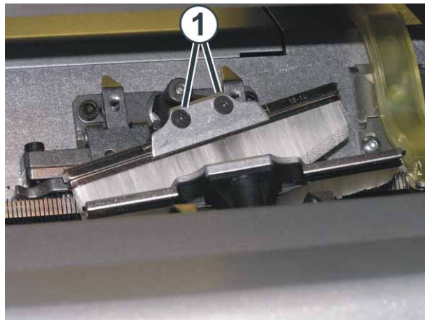
Fig. 4-60 Vis des brosses ouvre-clapets
