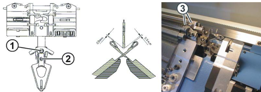
Fig. 4-61 Réglage des guide-fils intarsia
