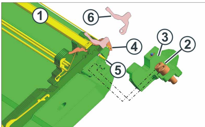
Fig. 6-11 Remplacement d'un conducteur de fil de la platine
