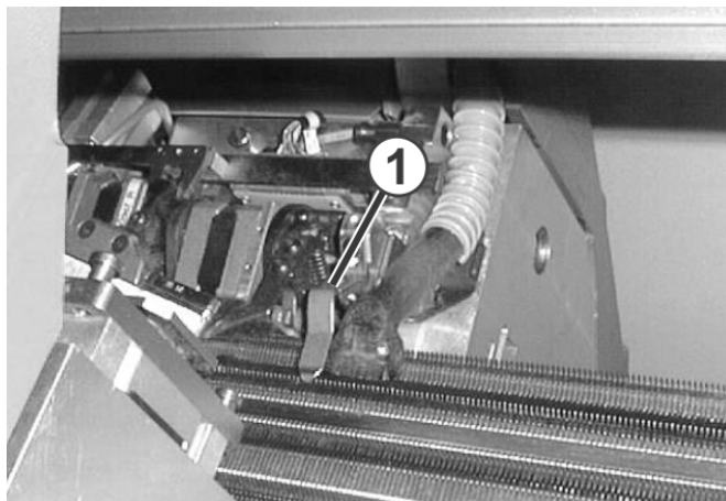
Fig. 6-29 Détecteur d'aiguilles
