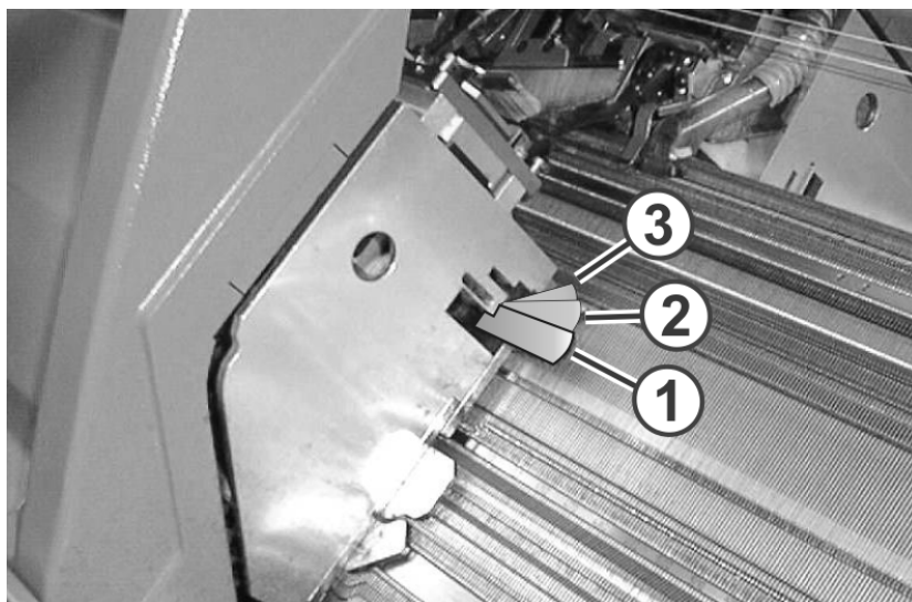
Fig. 2-23 Levier à cran au chariot
