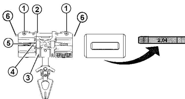
Fig. 4-63 Démontage de la plaquette de pression
