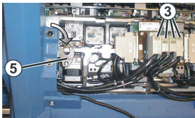
Fig. 6-27 Plaque pivotante
