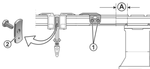
Fig. 6-42 Vis du limiteur de guide-fils
