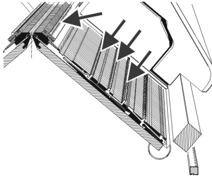
Fig. 2-17 Points de lubrification de la lubrification centrale
