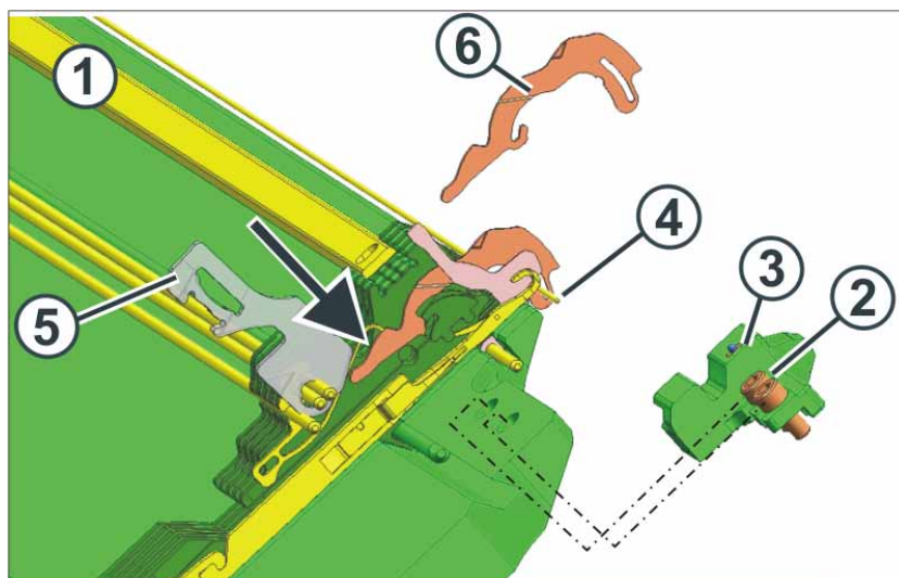
Fig. 6-9 Remplacement d'une platine d'appui
