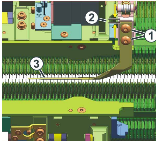
Fig. 4-50 Réglage des presse-mailles
