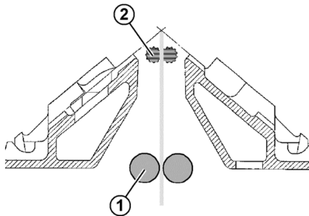
Fig. 2-29 Tirage auxiliaire
