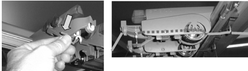
Fig. 3-11 Chemin du fil à travers le dispositif de contrôle du fil
