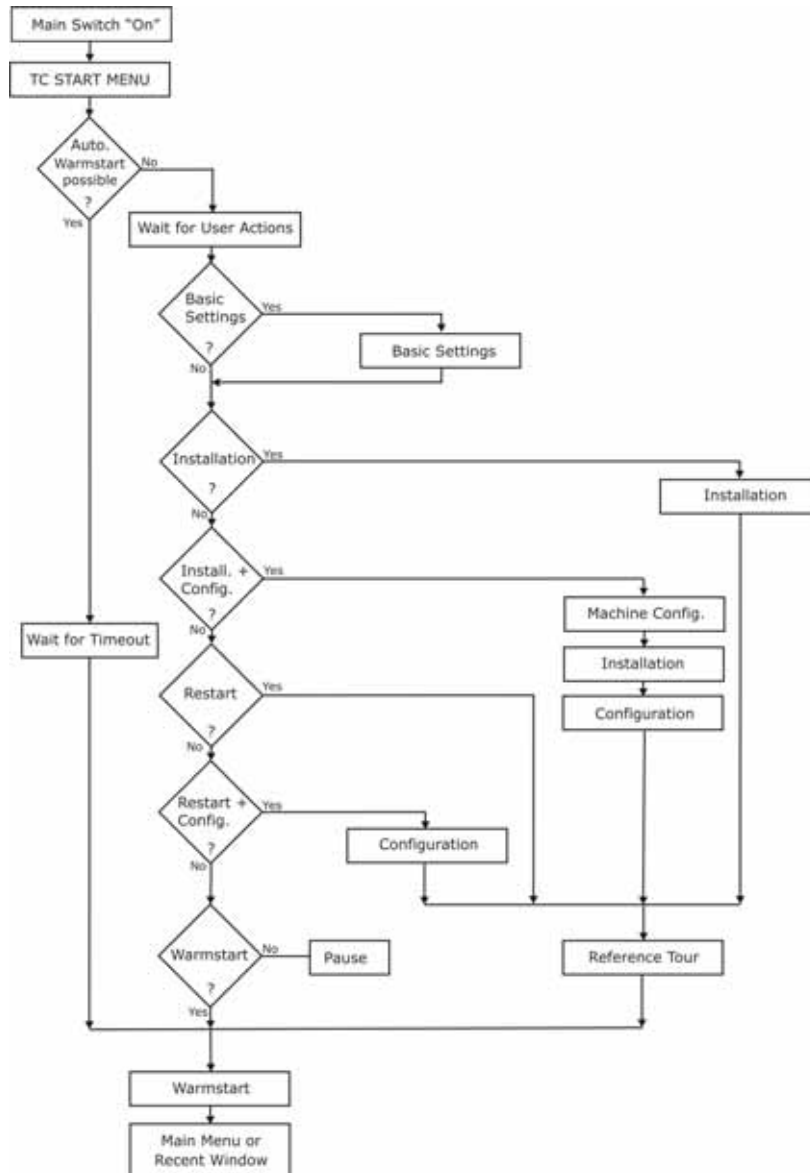
Fig. 7-1 Représentation schématique du processus de démarrage
