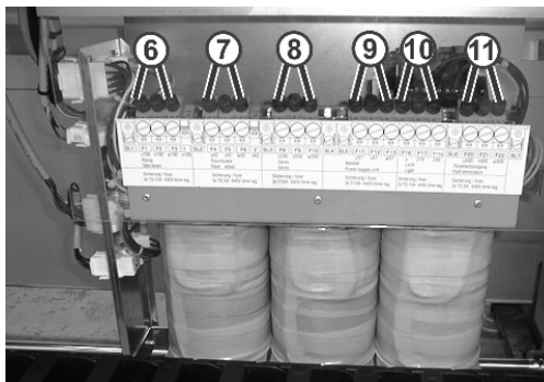
Fig. 6-60 Coupe-circuits au transformateur à l'arrière de la machine
