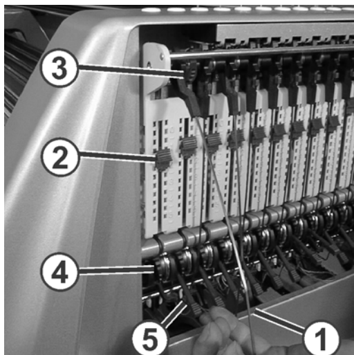
Fig. 4-8 Réglage de la tension du fil
