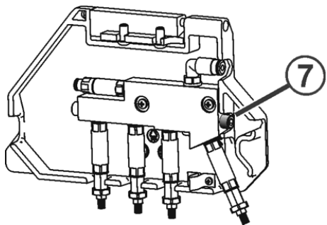
中央润滑装置油路脱气
