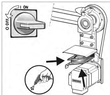
主驱动风扇
