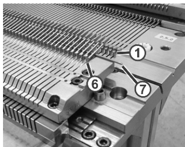
提起选针片
