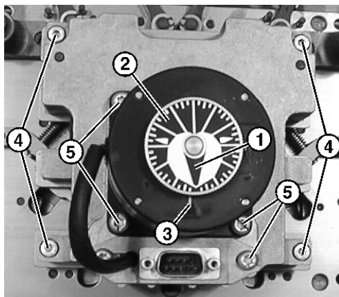
卸下密度马达
