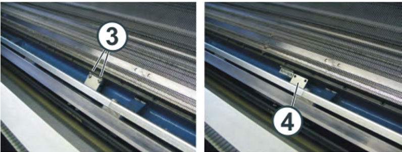
脉冲发生器导轨的连接
