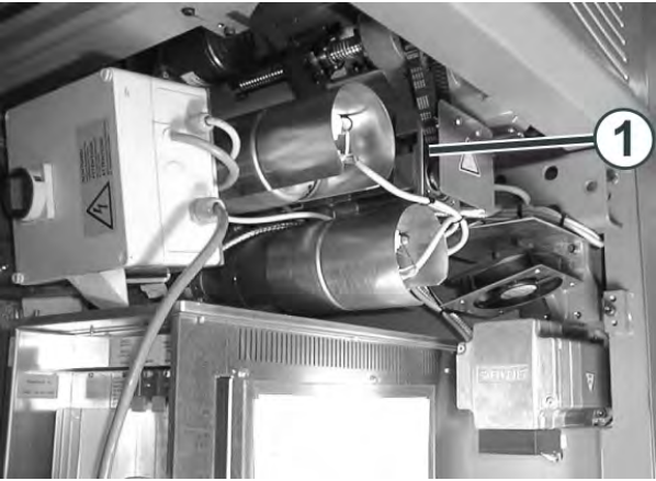
横移马达
