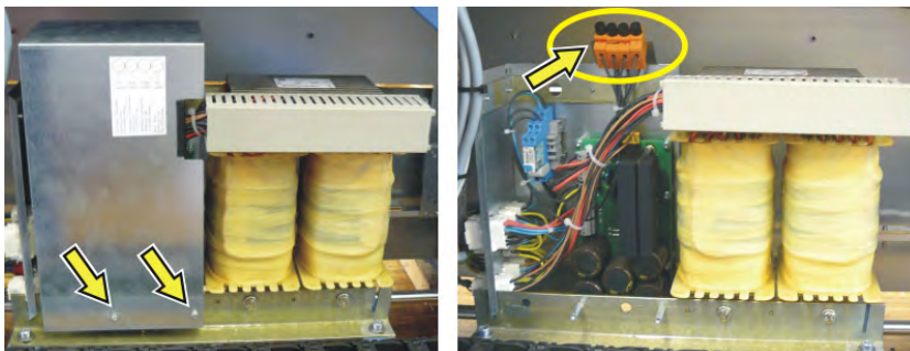
机器后面变压器上的保险管
