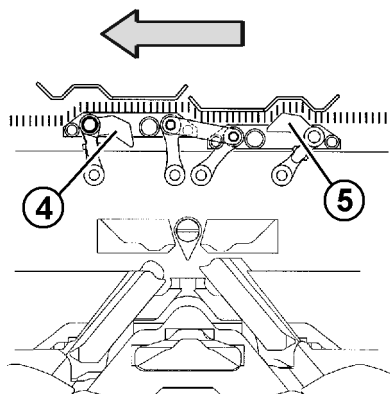
沉降片压板
