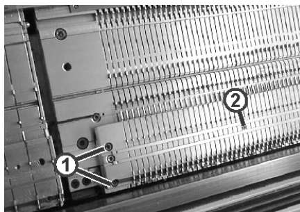
松开选针片床
