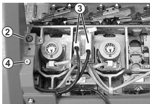
打开的机头
