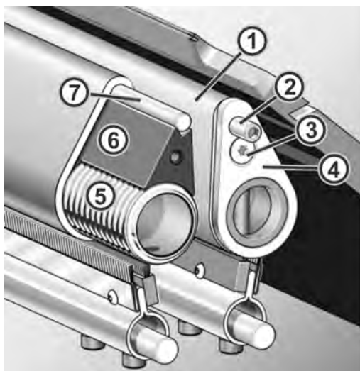
皮套牵拉，右视图
