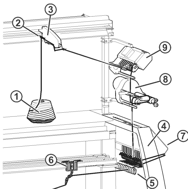
穿纱路径 4
