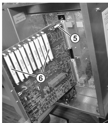
控制箱上伺服驱动和横移的镇流保险
