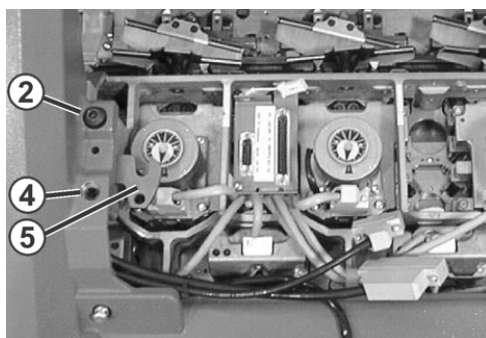
摆动板
