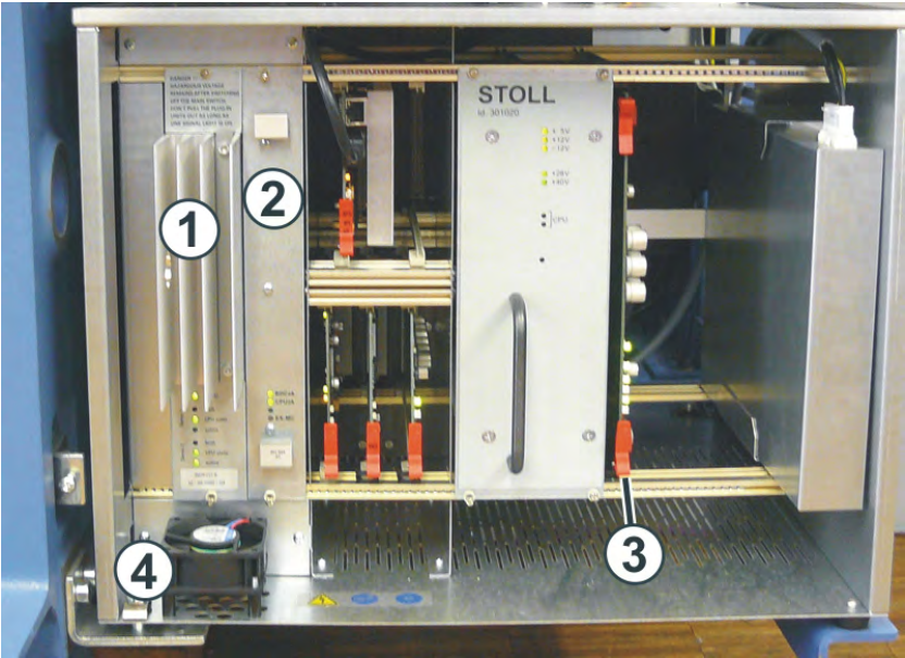
右控制箱
