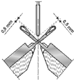
调节导纱器
