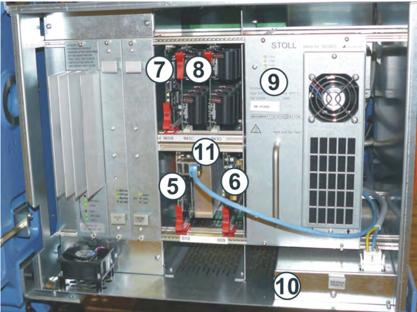
右控制箱
