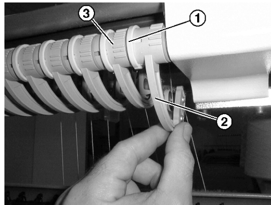
调节送纱器的送纱量
