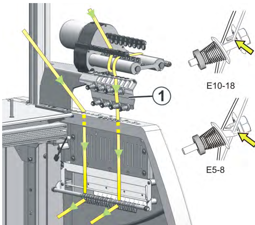
永久制动装置的穿纱路径
