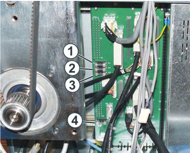
右侧控制箱背面的保险管（为便于观察，风扇被卸下）
