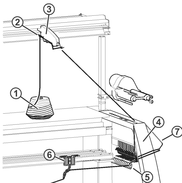
穿纱路径 2
