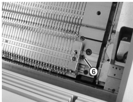
安装选针片床
