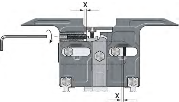
调节左侧的距离 ( 距离在右侧标尺上可见 )
