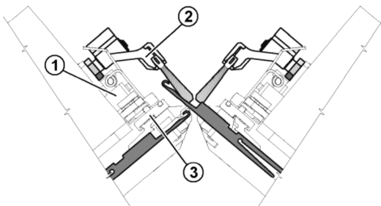
沉降片控制装置
