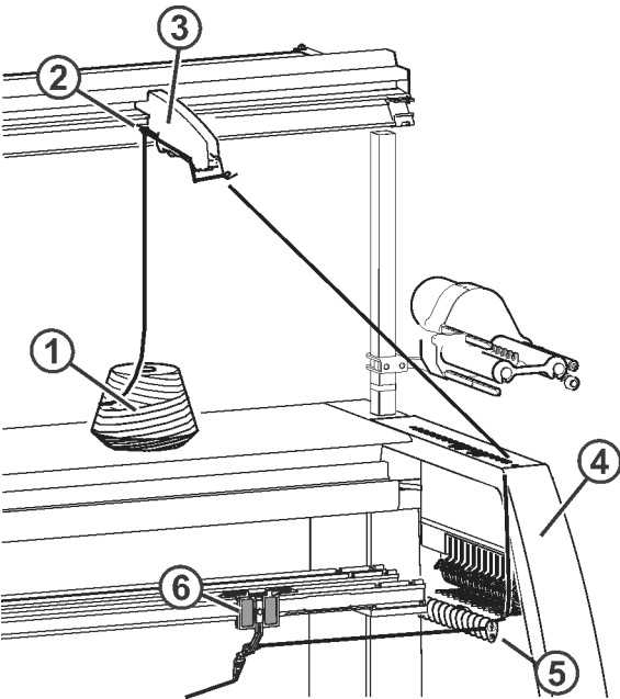
穿纱路径 1
