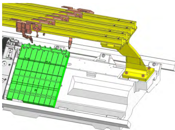
导纱器限位块的交错排列
