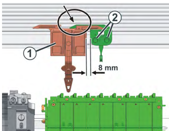
调节导纱器限位块
