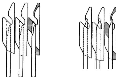
牵拉梳钩子以及滑片（左侧为开启状态，右侧为关闭状态）
