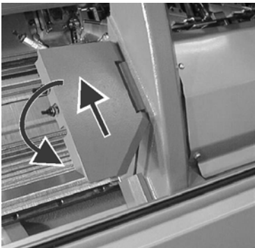
将中央润滑装置旋至工作位置
