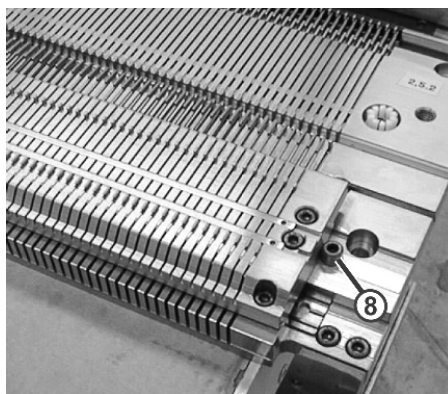
安装选针片床
