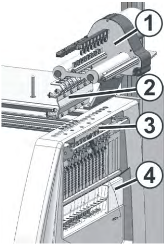
侧面导纱装置
