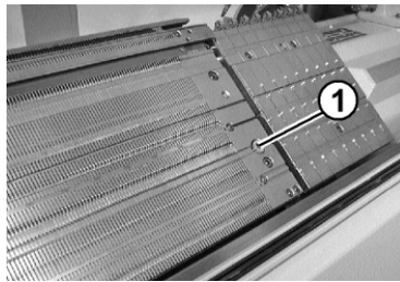
用于清洁选针系统的毛刷
