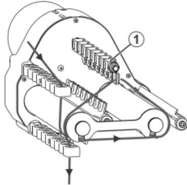
调节送纱器的送纱量
