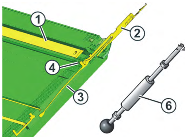
Cambio de aguja y de pieza de acoplamiento
