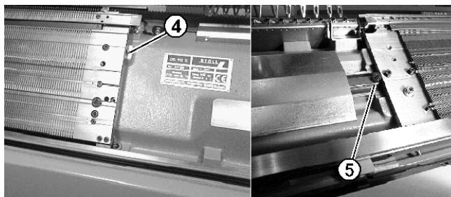
Montaje de la fontura anterior y posterior
