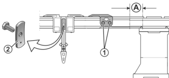
Tornillos del tope de guiahilos
