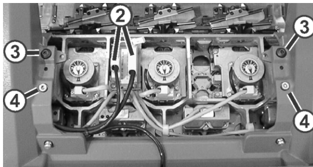
Fijación del carro en la parte del carro
