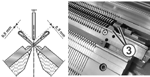
Ajuste de los guiahilos
