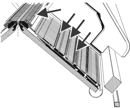
Puntos de lubricación de la lubricación central
