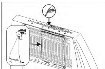
Limpieza del pinzahilos activo
