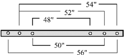
Anchuras de acoplamiento en la CMS 933
