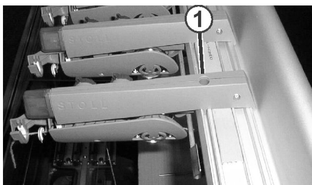
Desmontaje de una unidad de control del hilo
