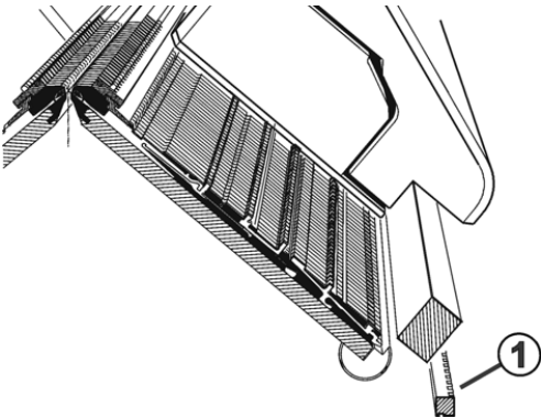
Engrase de las barras ranuradas del generador de impulsos
