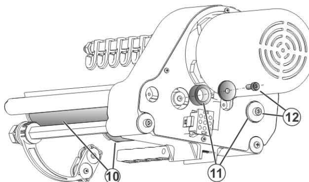
Tornillos para el rodillo de fricción
