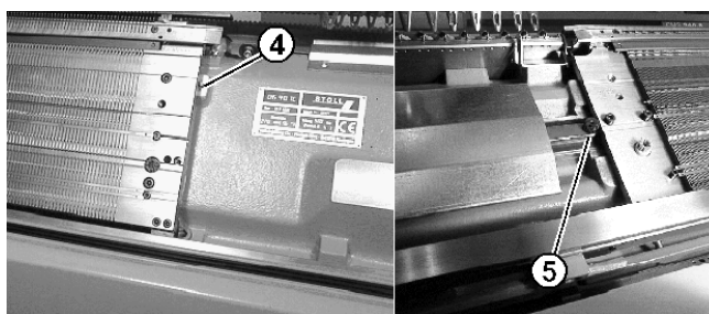
Установка передней и задней игольницы
