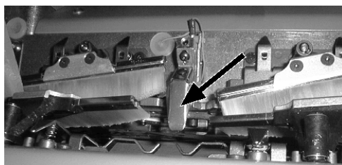
Контролер игл
