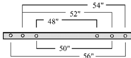
Расстояния стыковки на CMS 933
