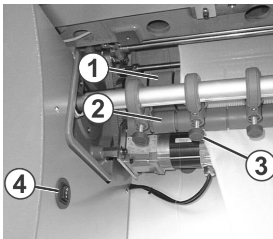
Главная оттяжка
