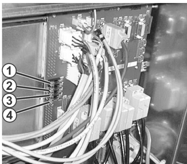
Предохранители на задней стороне левого устройства управления
