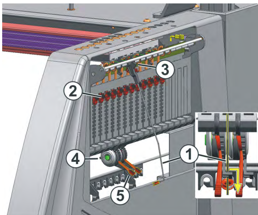
Настройка натяжения нити
