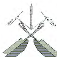
Настройка интарсийных нитеводителей
