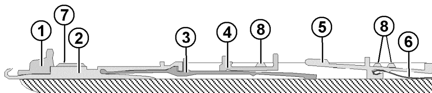
Игольница (Схематическое изображение)
