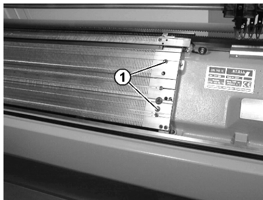
Отвинчивание игольницы
