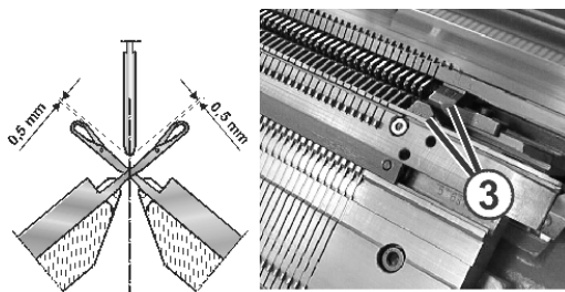
Настройка нитеводителей
