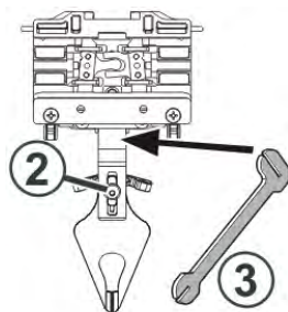
Настройка интарсийных нитеводителей
