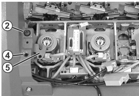
Поворотная пластина
