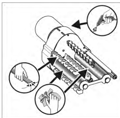
Чистка фрикционного фурнессера
