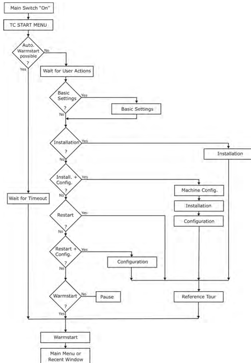
Schematische Darstellung des Bootvorgangs
