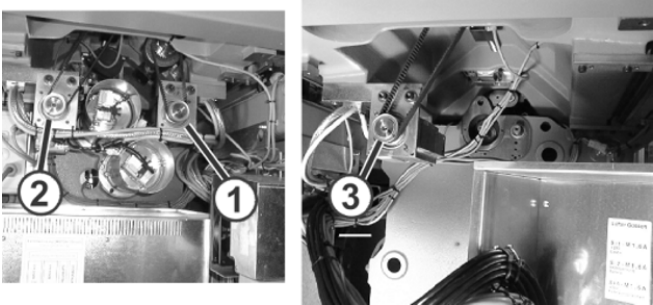
Versatzmotoren
