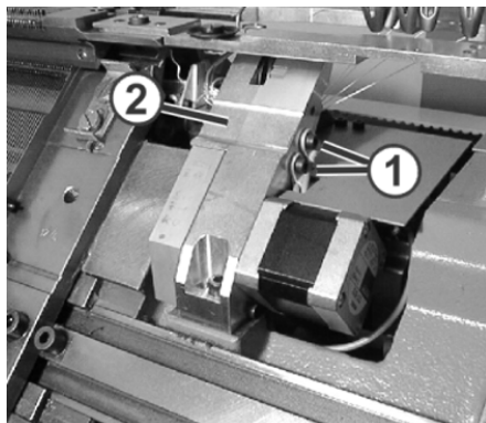
Schrauben des Fingerträgers
