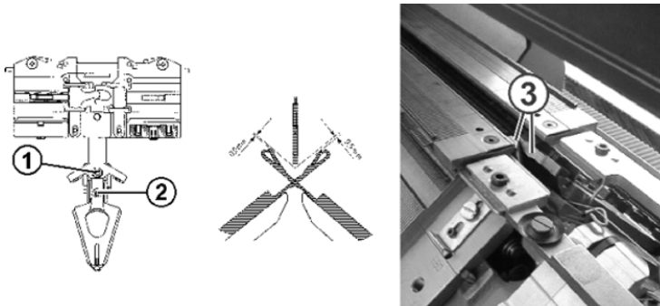
Einstellen der Intarsiafadenführer
