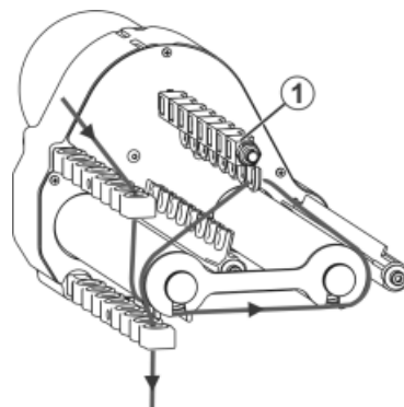
Einstellung der Fadenlieferung am Friktionsfournisseur
