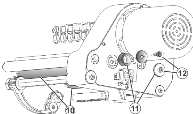
Schrauben für Friktionswalzen
