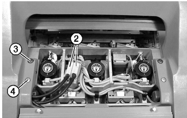
Befestigung des Schlittenwagens am Schlittenteil
