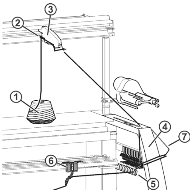
Fadenverlauf 2
