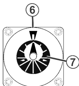
Grundstellung Schrittmotor
