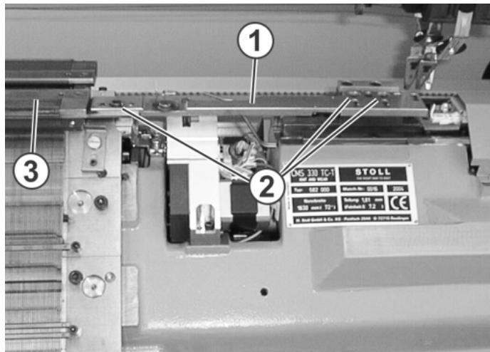
Abnehmen der Zusatzbetten
