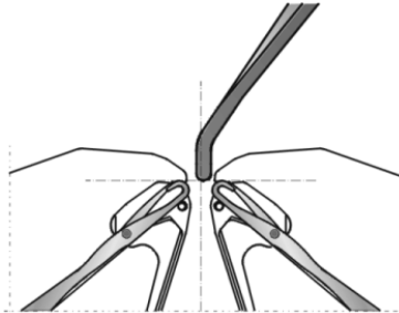
Einstellen des Nadelwächters
