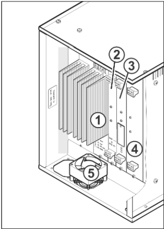
Steuerschrank rechts
