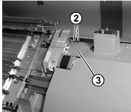
Abdeckung der Fadenklemm- und Schneideinrichtung
