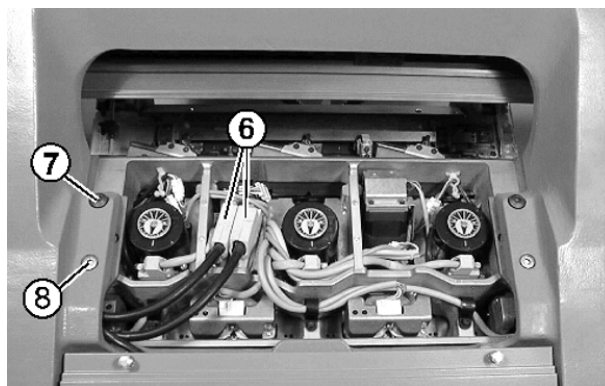
Geöffneter Schlittenwagen
