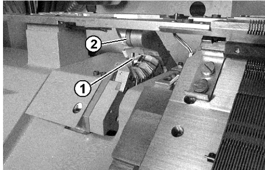
Fadenklemm- und Schneideinrichtung
