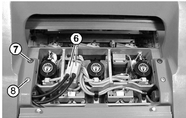
geöffneter Schlittenwagen
