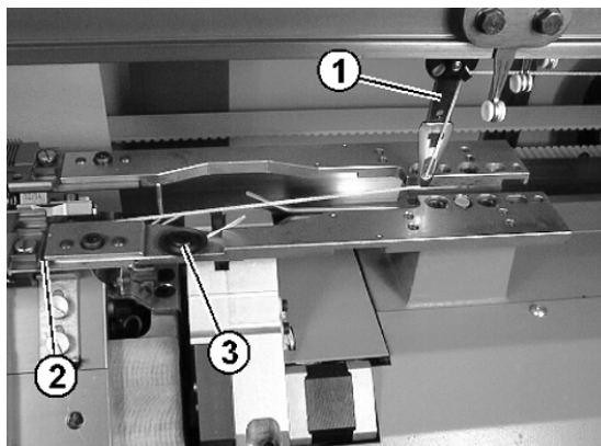
Faden einfädeln
