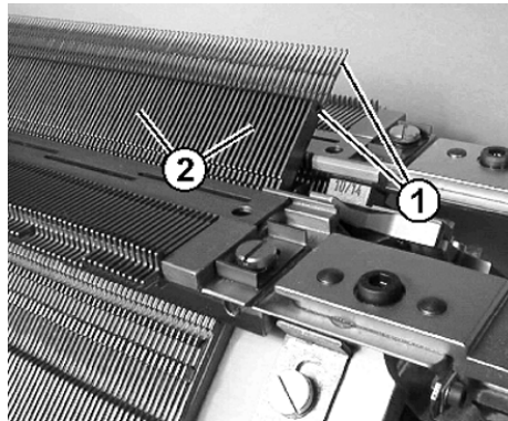
Reinigen des Nadelbetts
