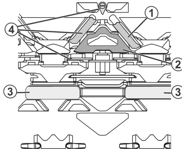
Stricksystem
