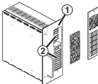
Lüfter Netzteil
