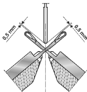
Einstellen der Fadenführer
