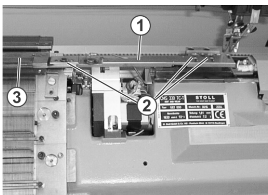
Abnehmen der Zusatzbetten
