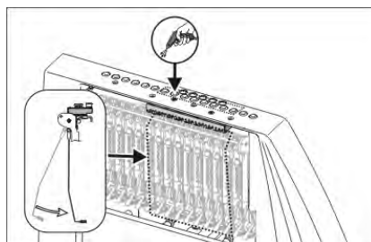
Reinigen der aktiven Fadenklemme
