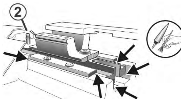
Versatzeinrichtung der Zusatzbetten fetten
