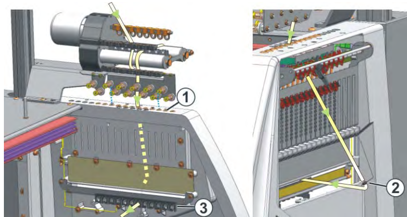
Weg des Fadens durch die seitliche Sicherheitshaube
