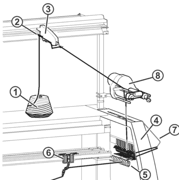
Fadenverlauf 3
