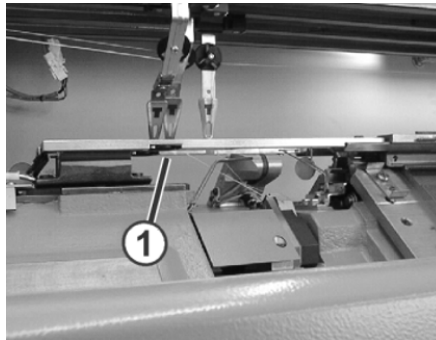
Stoßabstellung für Zusatzbetten
