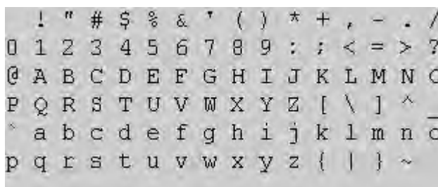
ASCII-Zeichensatz
