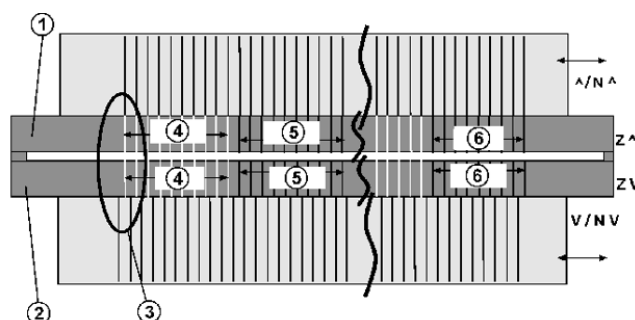
Grundstellung der Nadelbetten zu den Zusatzbetten
