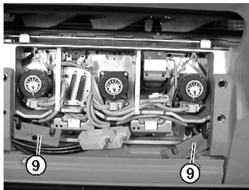
Linke und rechte Schwenkplatte
