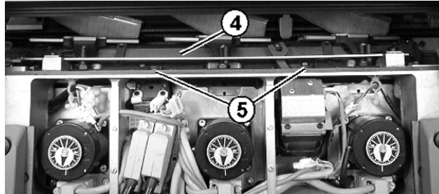
Ausbauen des Zusatzschlosses
