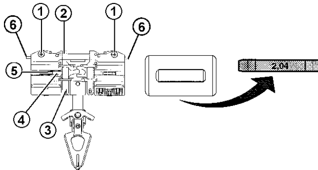
Ausbau des Druckplättchens
