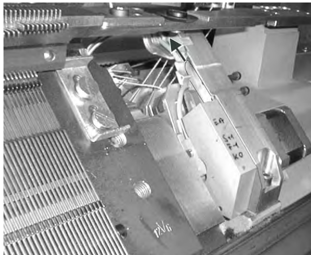
Zahnriemen in Pfeilrichtung spannen
