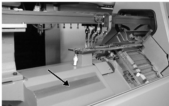
Auflagefläche links für Schlittenteil
