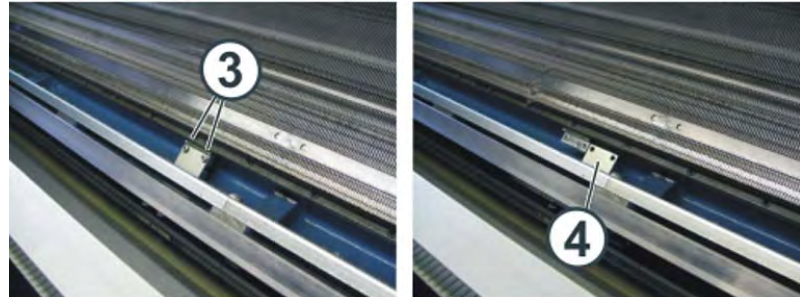
Anbindung der Impulsgeberschiene
