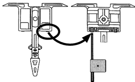
Einstellen der Führung des Fadenführers
