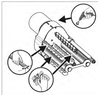
Reinigen des Friktionsfournisseurs
