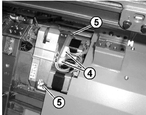
Kabel und Schrauben der Fadenklemm- und Schneideinrichtung
