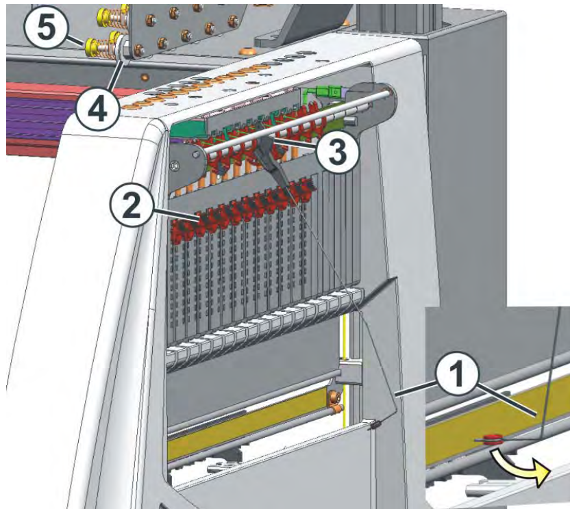
Einstellen der Fadenspannung
