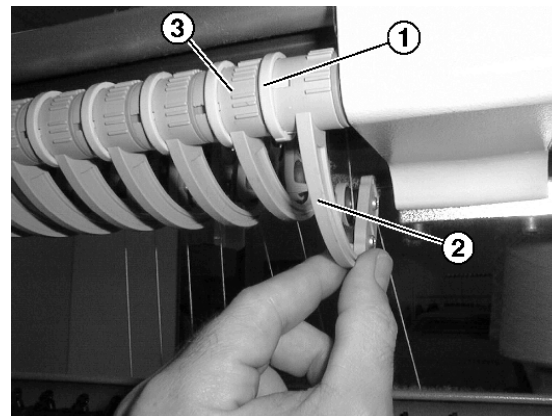
Einstellung der Fadenlieferung am Friktionsfournisseur
