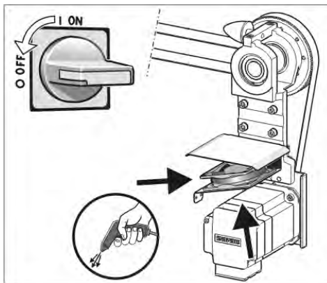
Lüfter Hauptantrieb
