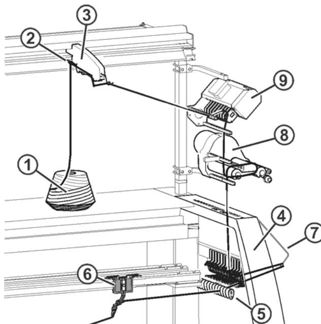
Fadenverlauf 4
