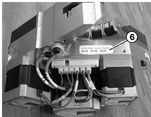
Aufkleber Korrekturwerte
