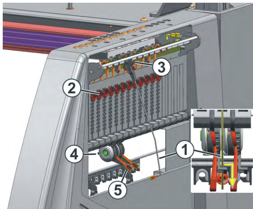
Einstellen der Fadenspannung
