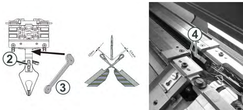
Einstellen der Intarsiafadenführer
