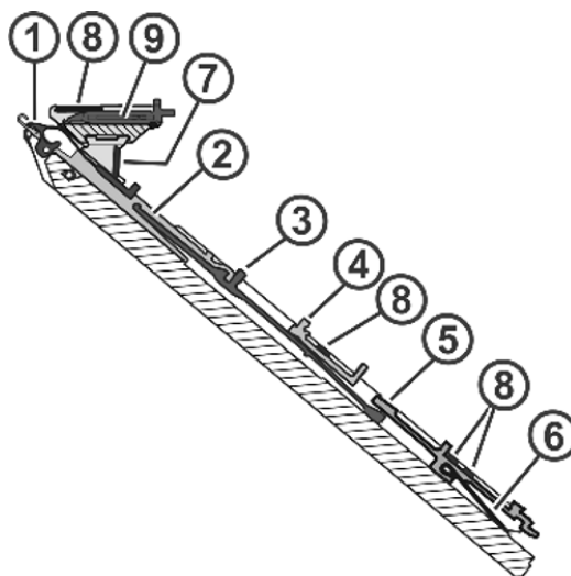
Nadelbett (Schematische Darstellung)
