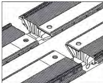
Verbindungsstelle reinigen
