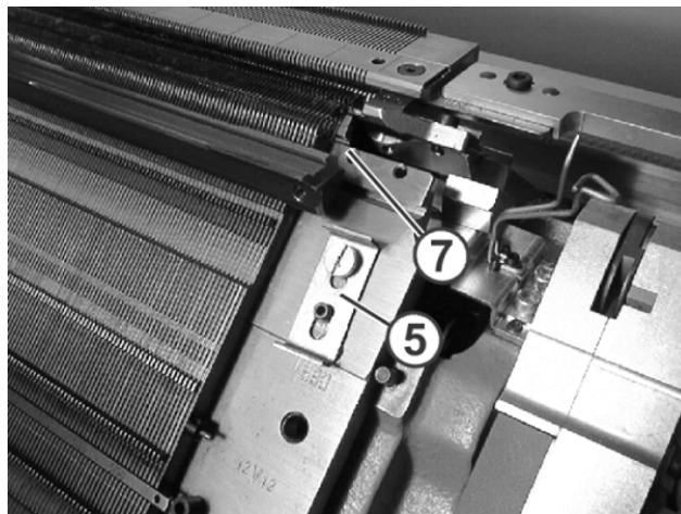
Draht als Platinenhalterung
