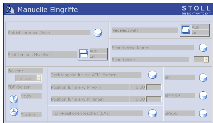
Gesperrtes Fenster "Manuelle Eingriffe"
