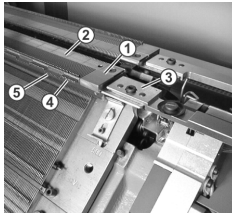
Zusatzbett
