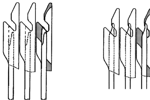
Kammhaken des Kammabzugs mit Schiebern (links offen, rechts geschlossen)
