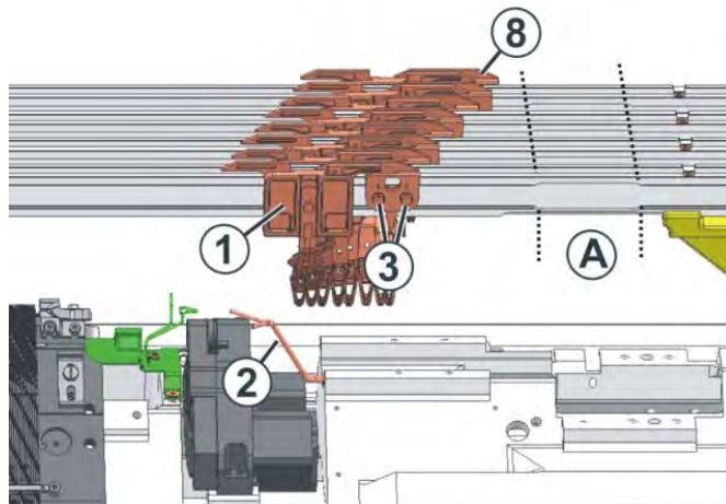
Einstellen der Fadenführerbegrenzer
