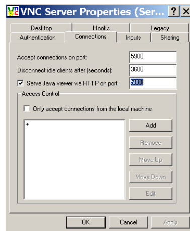
Fenster "VNC Server Properties (Service-Mode)" mit der Registerkarte "Connections"
