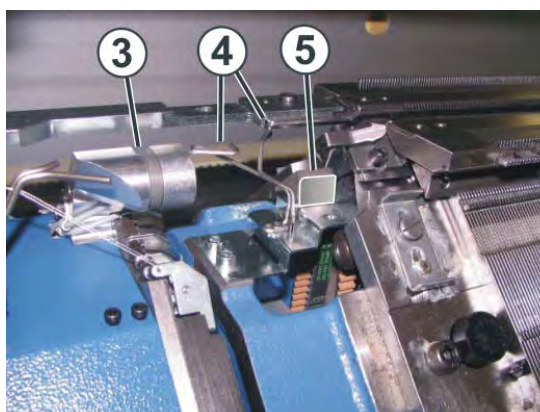
Fadenleitsystem
