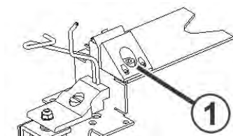
Einstellen der Fadenklemme
