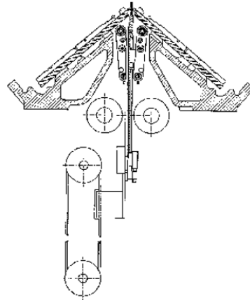
Kammabzug
