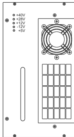
Netzteil
