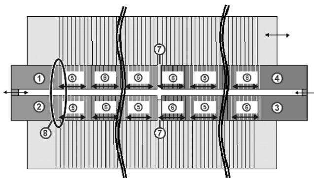
Grundstellung der Nadelbetten zu den Zusatzbetten
