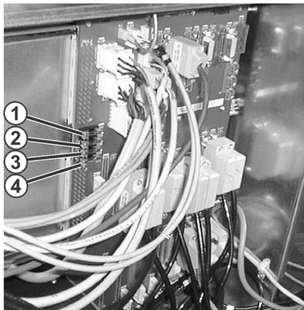
Sicherungen auf Rückseite des linken Steuergerätes
