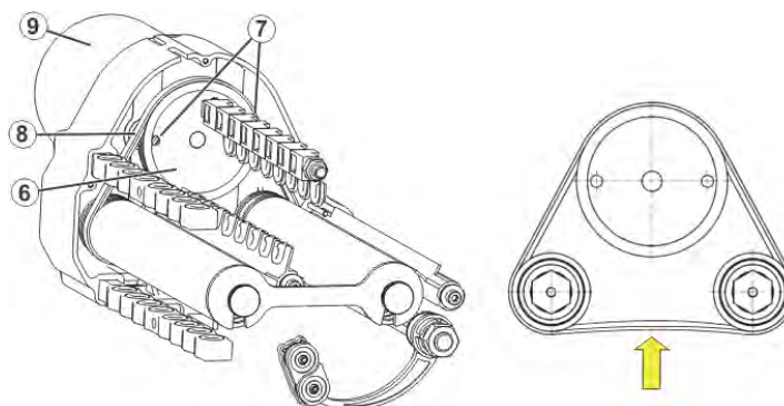
Antriebsriemen
