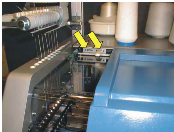
USB-Buchsen
