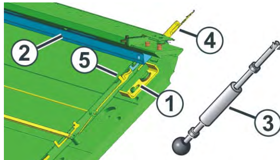
Nadelschiene und Ausziehhaken
