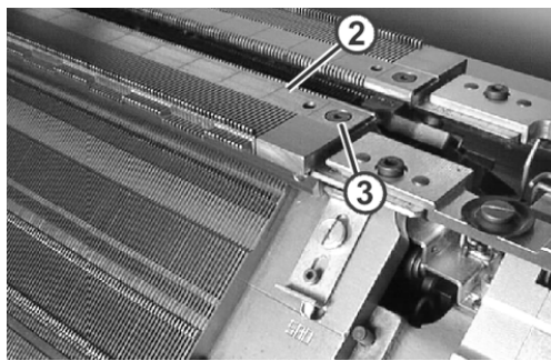
Zusatzbett
