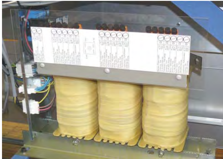
Sicherungen am Transformator auf Maschinenrückseite
