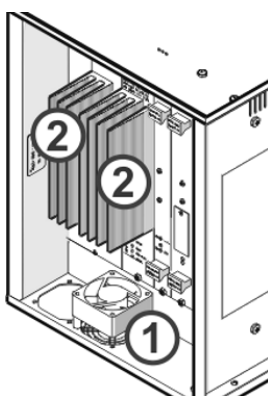
Steuergerät
