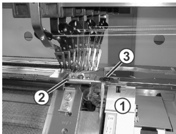
Faden einfädeln
