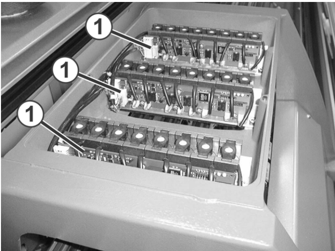
Elektronikkarten zur Steuerung der Fadenführermagnete
