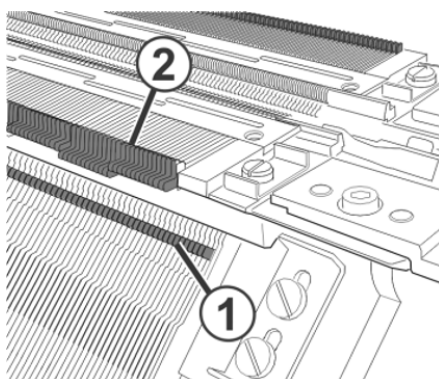
Ölen der Füße der Niederhalteplatte (1) und der Umhängeteile (2)
