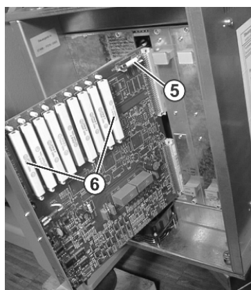
Ballastsicherung (5) für Servo-Antrieb und Versatz am Steuergerät rechts
