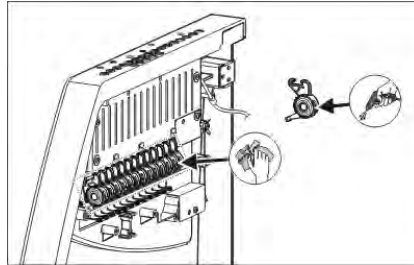
Reinigen der Permanentbremse
