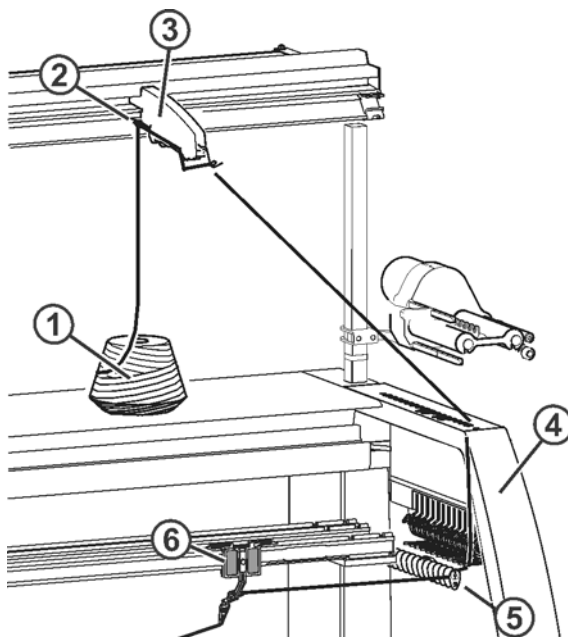
Fadenverlauf 1
