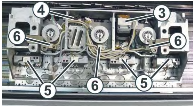
Stecker der Auswahlssysteme
