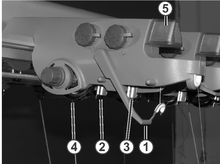
Fadenkontrolleinheit
