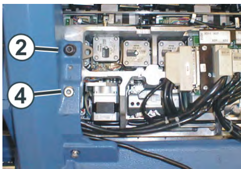
打开的机头
