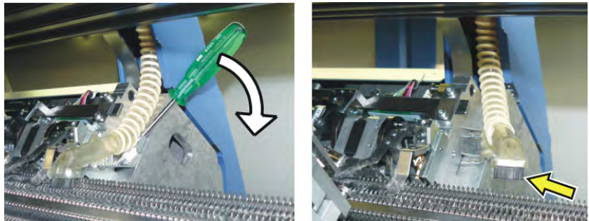
吸管
