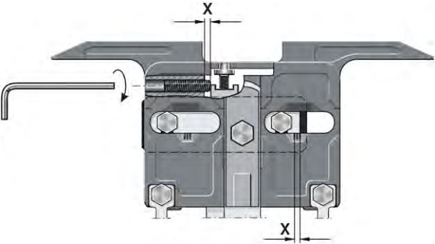
调节左侧的距离 (距离在右侧标尺上可见)
