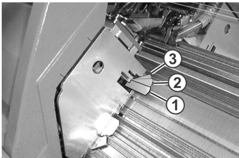
机头上的锁定杆
