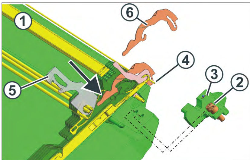
更换沉降片
