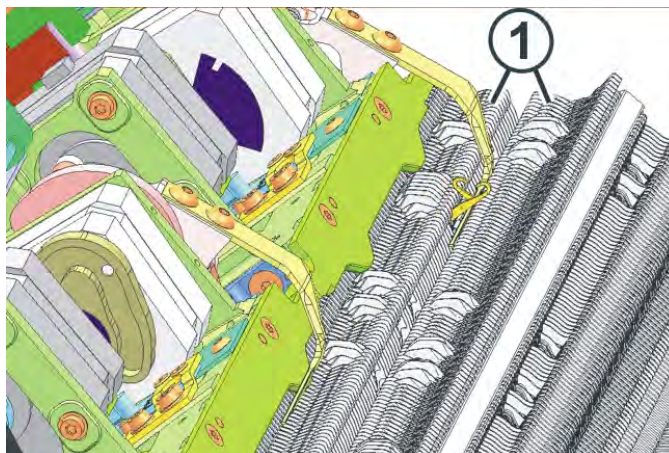
沉降片
