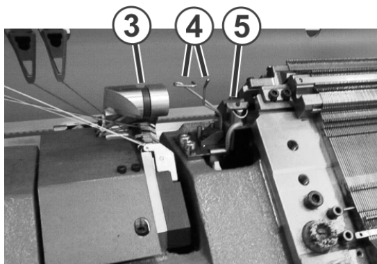
导纱系统
