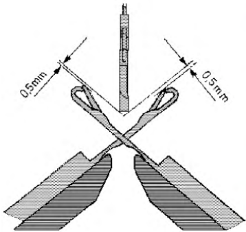
调节导纱器
