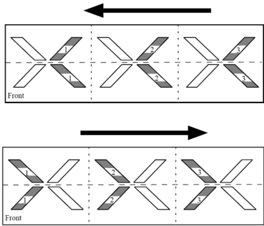
3 系统编织机成圈三角的编号
