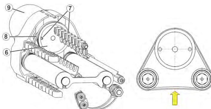
皮带
