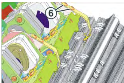
工作状态的压脚
