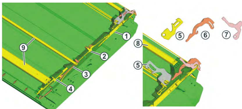
针床（示意图）
