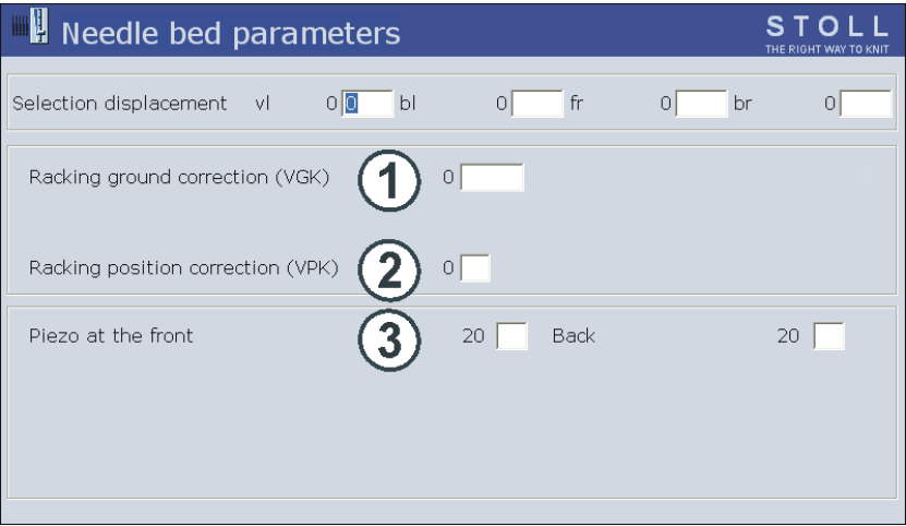
“针床参数”窗口
