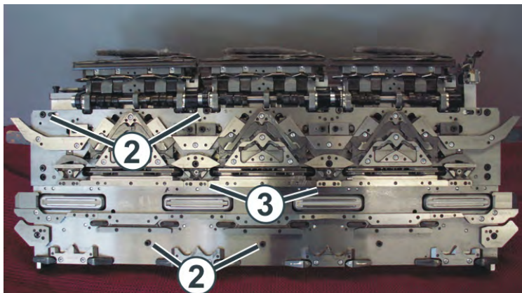
三角底板上铸件的螺丝
