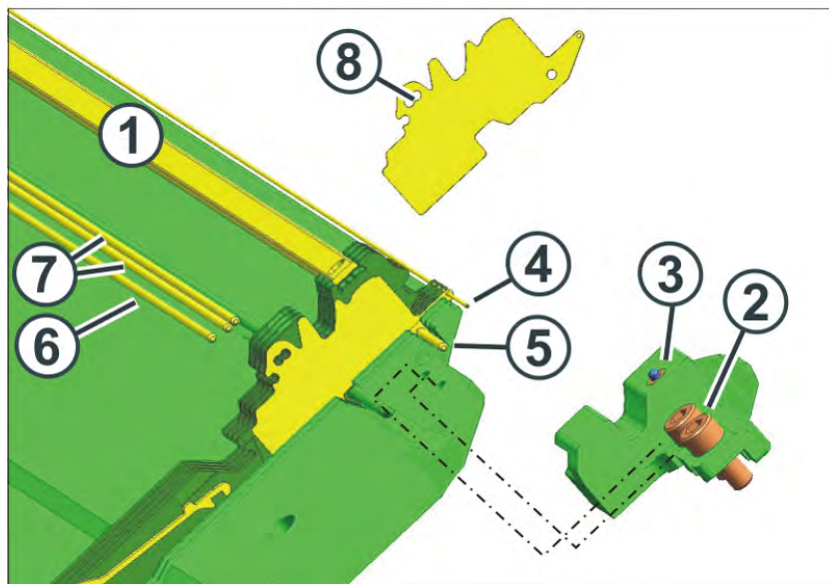
更换钢丝支架
