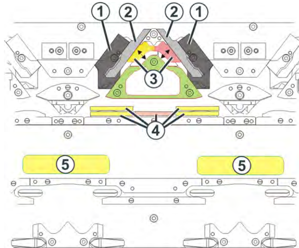
编织系统
