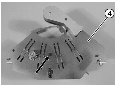
中间板
