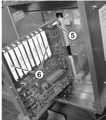
控制箱上伺服驱动和横移的镇流保险（5）
