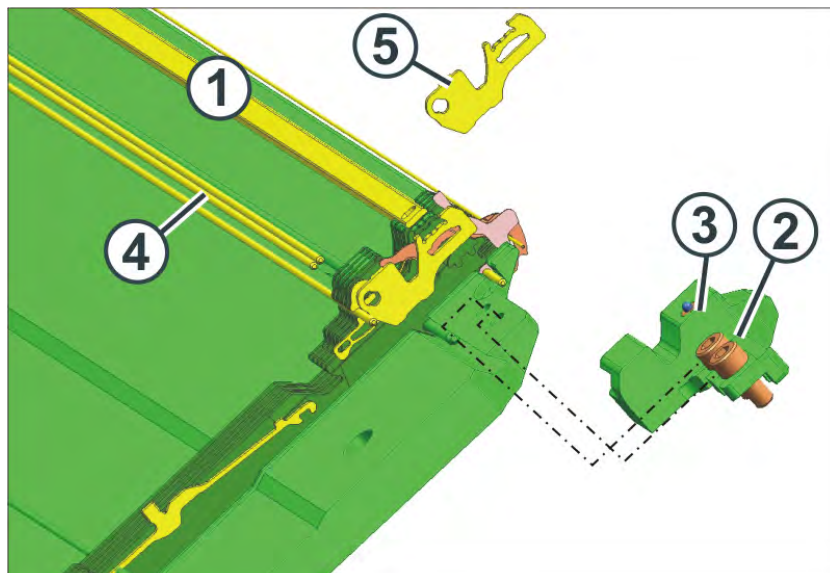
更换织针导向件
