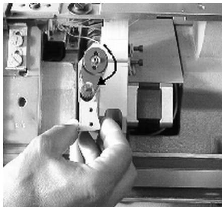
传送片的原始位置
