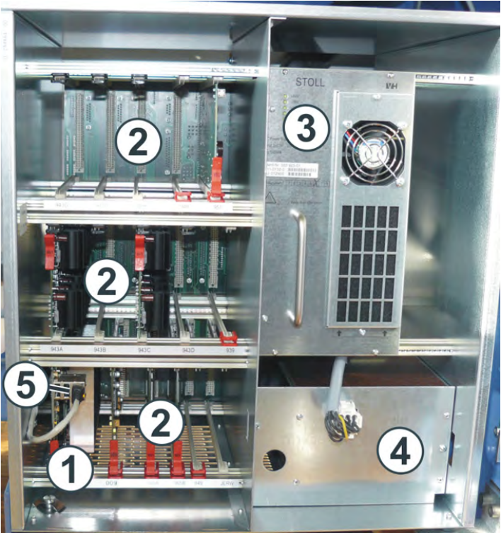
左控制箱
