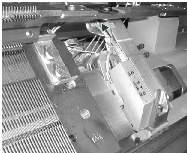
按箭头方向拉紧齿形皮带
