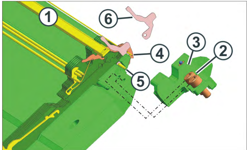
更换导纱钩
