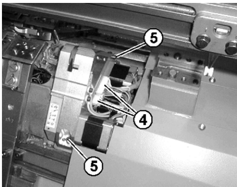
切夹纱装置的电缆线和螺丝
