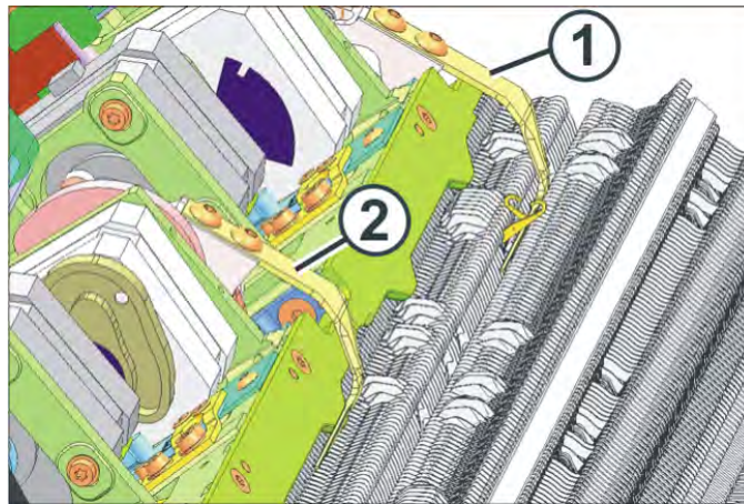
带步进马达的压脚
