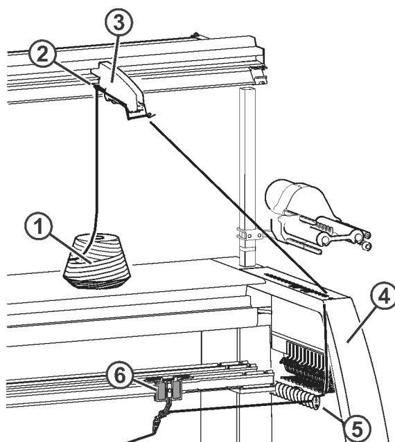
穿纱路径 1
