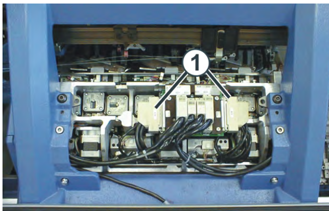
插头（密度马达、选针系统）
