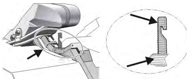
切夹纱剪刀和夹纱小齿轮
