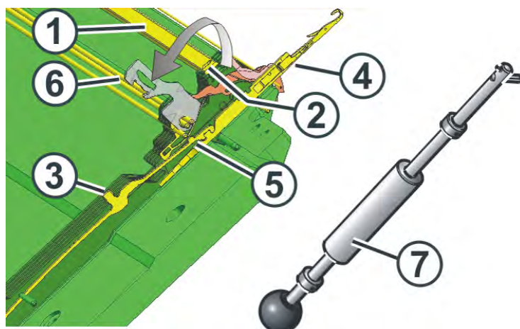
更换织针和挺针片
