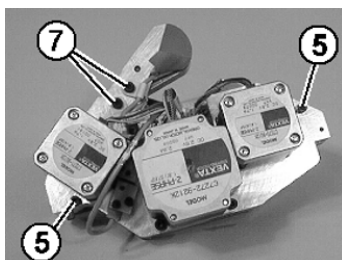
切夹纱装置
