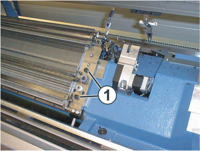
松开针床
