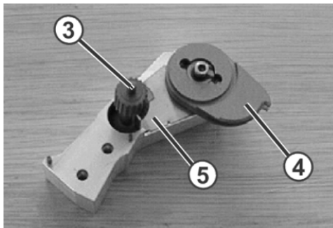
指型支架元件
