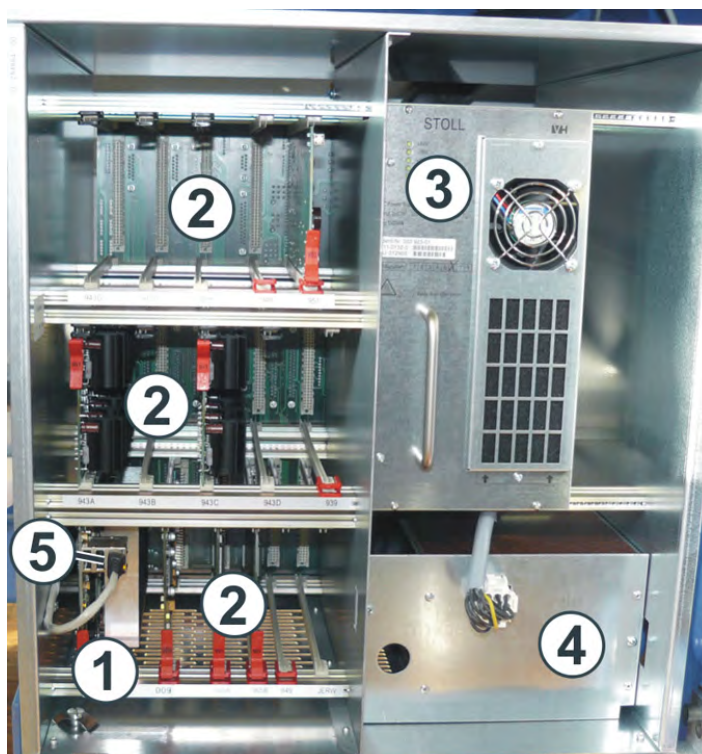
Armario de control izquierdo
