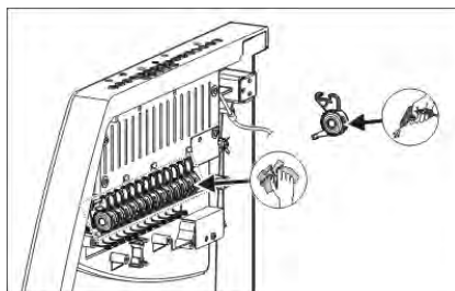
Limpieza del freno permanente
