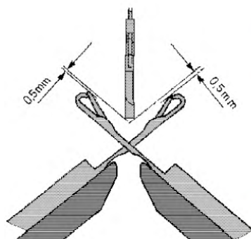
Ajuste de los guiahilos
