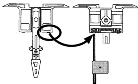
Ajuste de la guía del guiahilos
