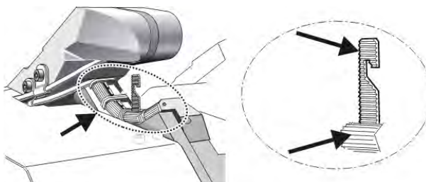
Aguja de pinzado y de corte y piñón de sujeción
