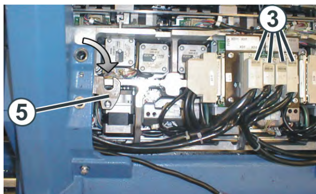
Placas basculantes
