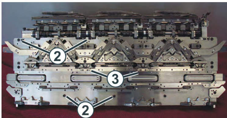
Tornillos para cuerpo fundido en la placa de cerrojos
