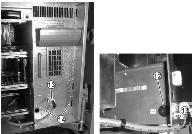
Fusible de batería (12) debajo de la fuente de alimentación
