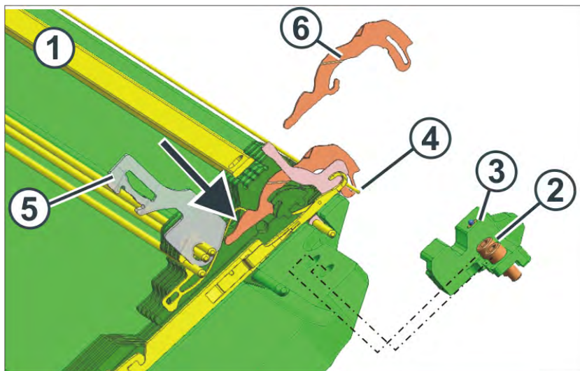
Sustitución de una platina de retención
