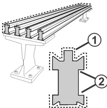
Aceitado de las barras de guiahilos
