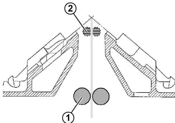
Estirador auxiliar
