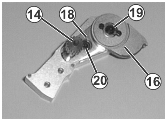
Soporte de los dedos
