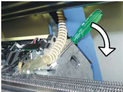
Tubo de aspiración
