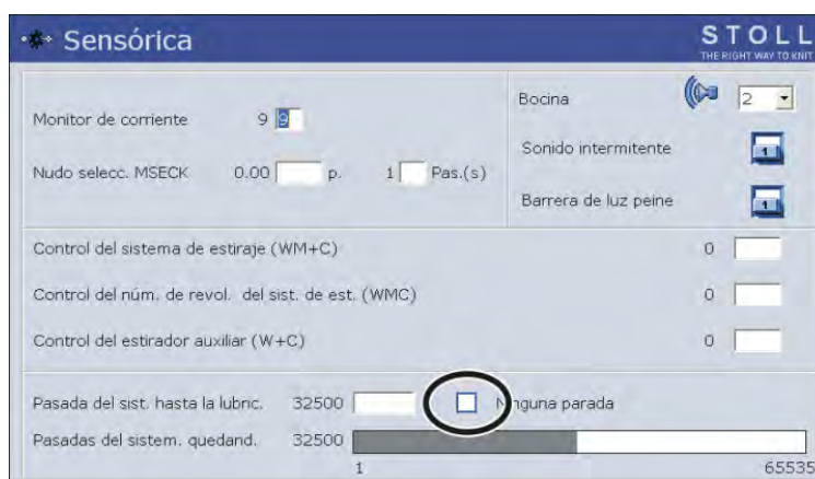
Ventana "Sensórica"
