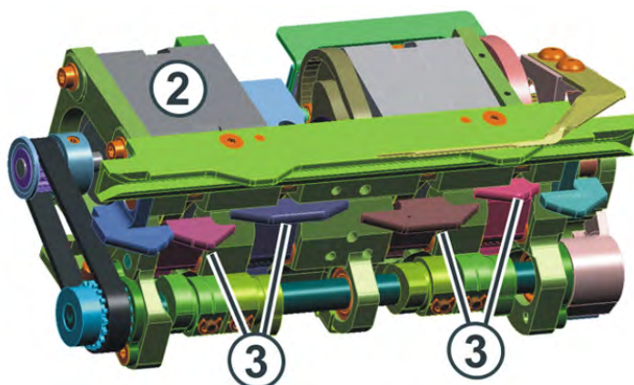
Control de las platinas de retención
