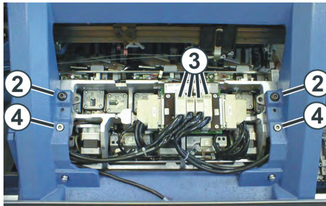
Fijación del carro en la parte del carro
