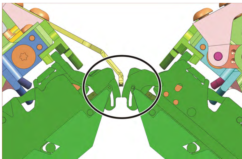
Ajuste de los prensamallas
