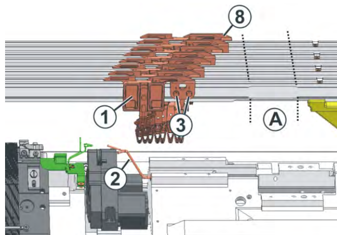
Ajuste del tope de guiahilos
