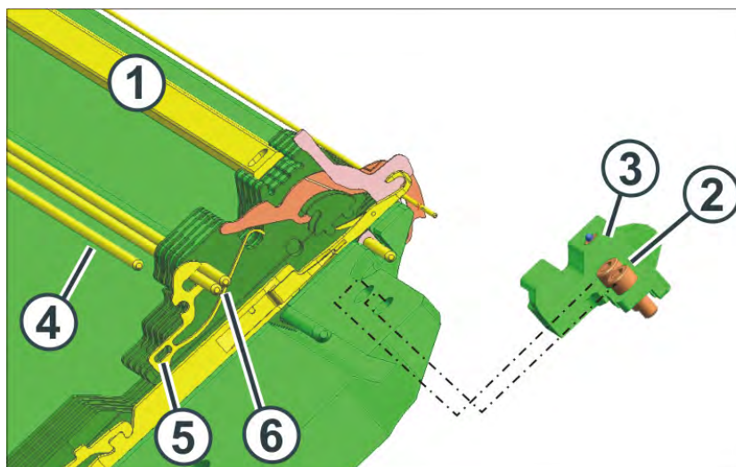
Cambio de un resorte de la platina de retención
