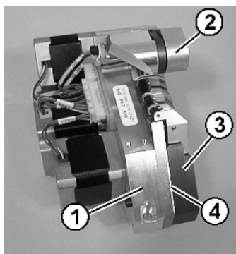
Carcasa del dispositivo de pinzado y de corte del hilo
