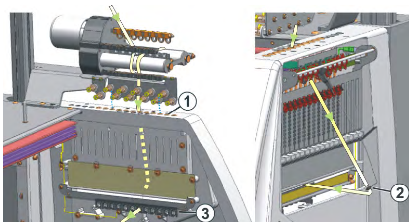
Recorrido del hilo a través de la cubierta de protección lateral
