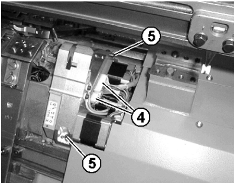
Cable y tornillos del dispositivo de pinzado y de corte del hilo
