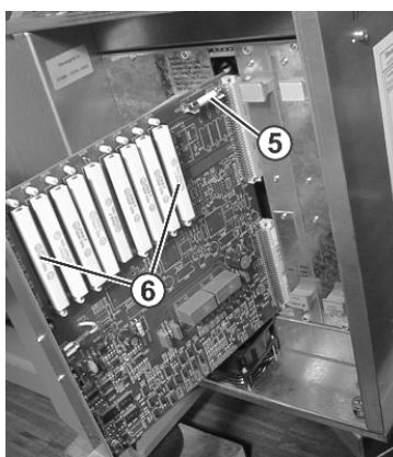
Fusible de sobrecarga (5) para el accionamiento servo y el variador en la unidad de control de la derecha
