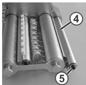
Ajustar la distancia entre la guía de parada y el rodillo de fricción
