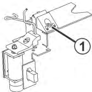
Ajuste del pinzahilos
