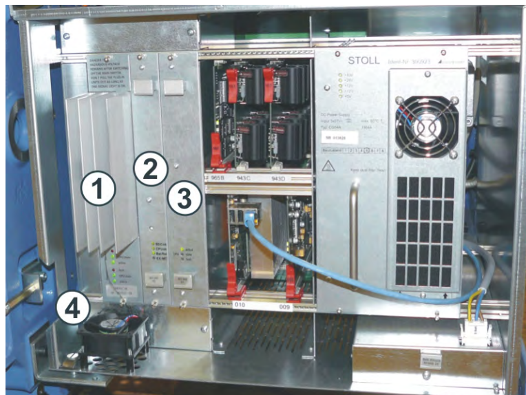
Steuerschrank rechts
