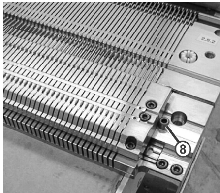
Einbau des Auswahlplatinenbetts
