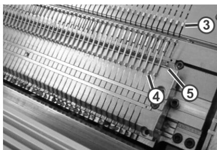
Hochheben der Auswahlplatinen
