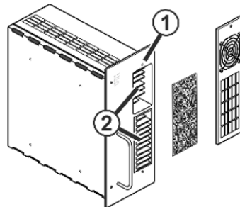
Lüfter Netzteil
