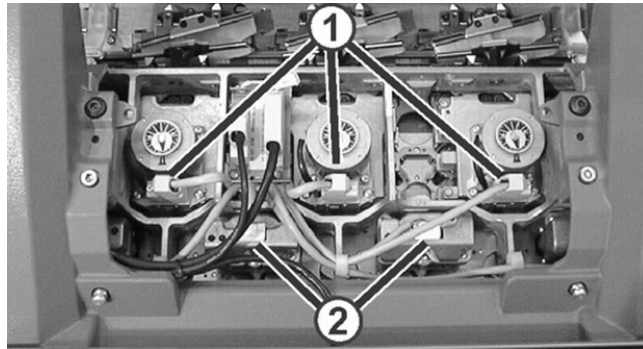
Stecker der Auswahlssysteme
