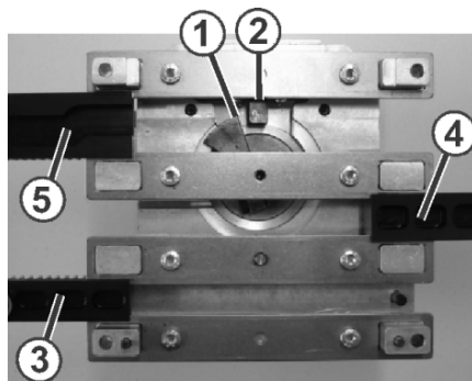
Einbauposition
