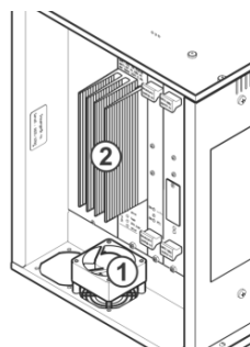
Steuergerät
