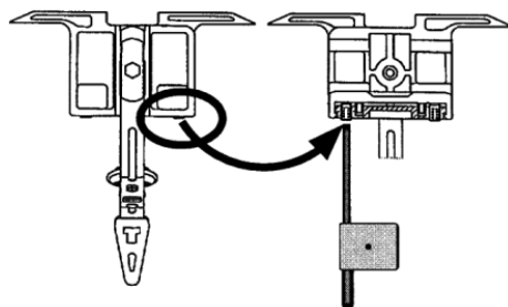
Einstellen der Führung des Fadenführers
