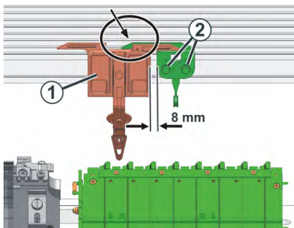
Einstellen der Fadenführerbegrenzer
