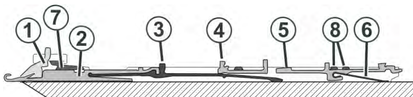
Abb. 27: Nadelbett (Schematische Darstellung)
