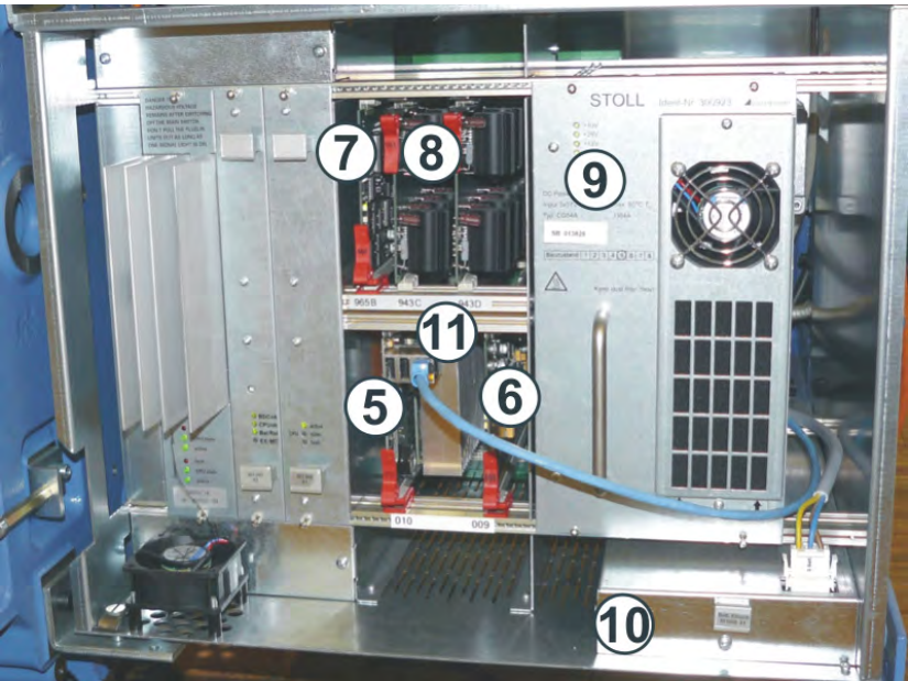
Steuerschrank rechts
