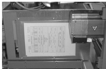
Maschinendatenblatt am rechten Steuerschrank
