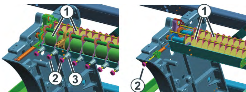
Abb. 29: Hauptabzug (rechtes Bild: CMS 502)
