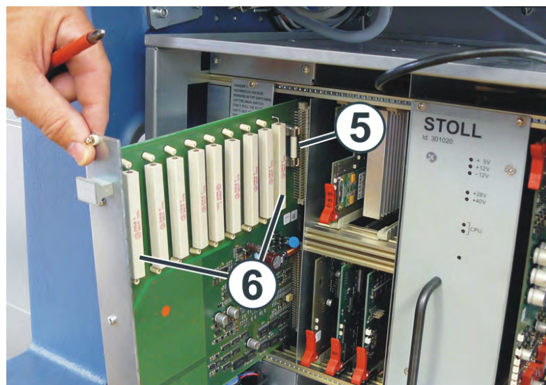
Ballastsicherung für Servo-Antrieb und Versatz auf der Input-, Output-Karte
