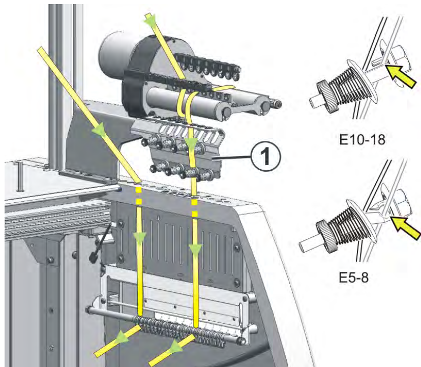
Weg des Fadens durch die Permanentbremse
