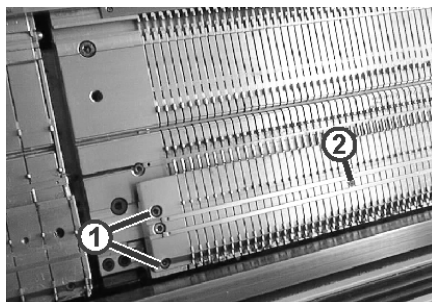
Lösen des Auswahlplatinenbetts
