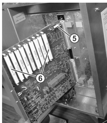
Ballastsicherung für Servo-Antrieb und Versatz am Steuergerät rechts
