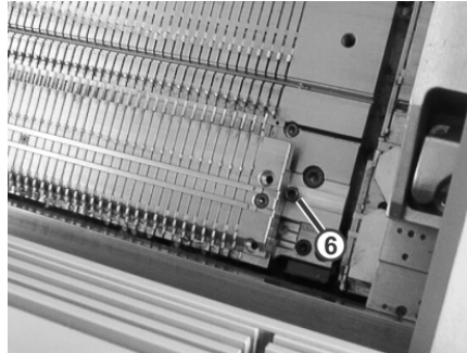
Einbau des Auswahlplatinenbetts
