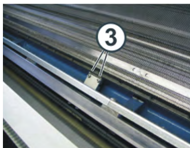
Anbindung der Impulsgeberschiene
