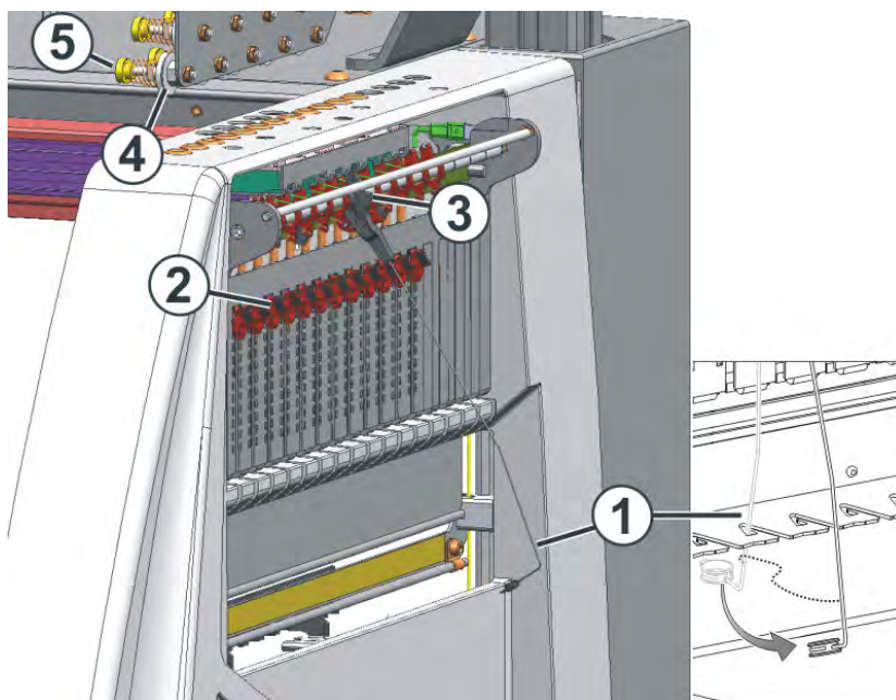
Einstellen der Fadenspannung
