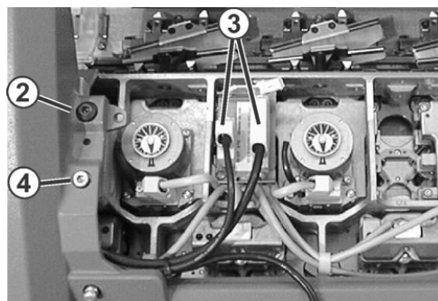
Geöffneter Schlittenwagen
