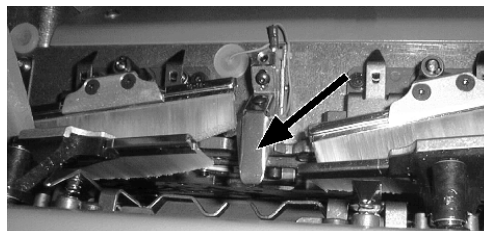
Nadelwächter
