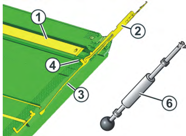
Wechseln von Nadel und Kupplungsteil
