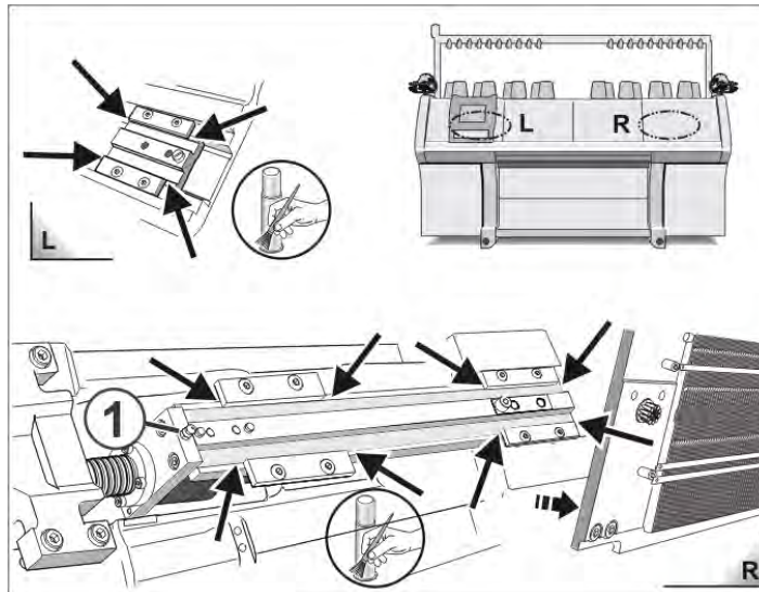
Versatzeinrichtung fetten
