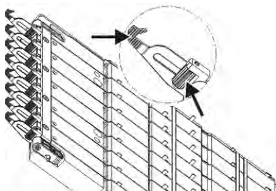
Reinigen der Fadenklemm- und Schneideinrichtung
