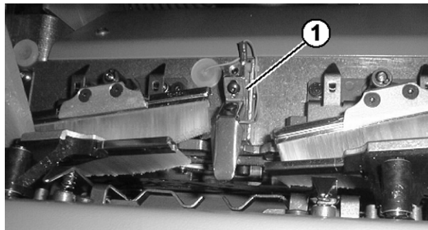
Nadelwächter
