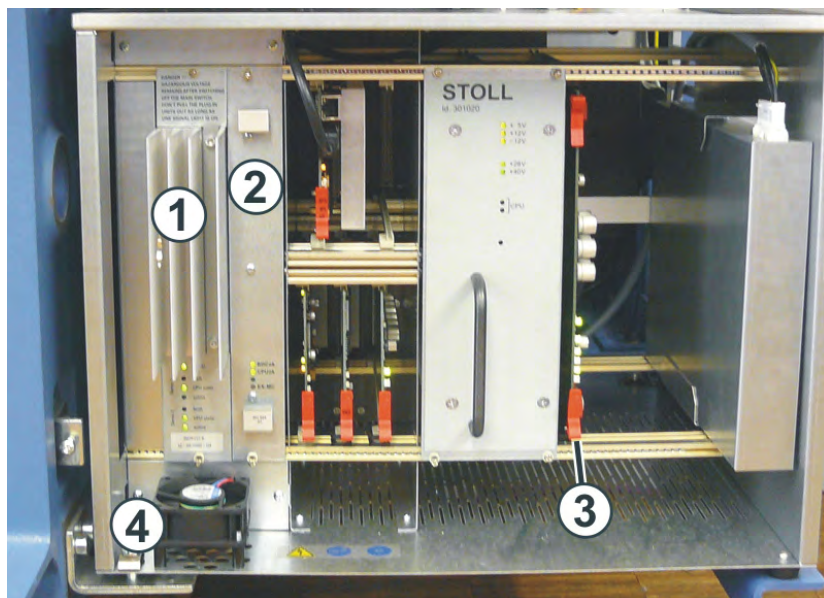
Steuerschrank rechts
