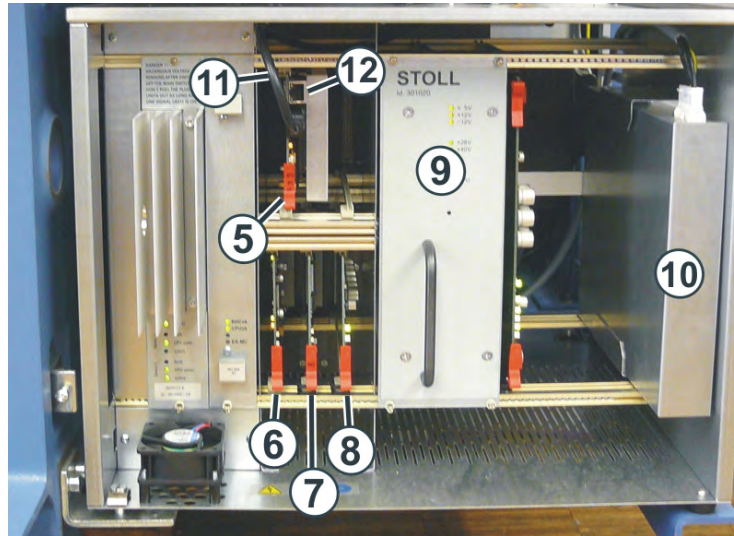
Steuerschrank rechts
