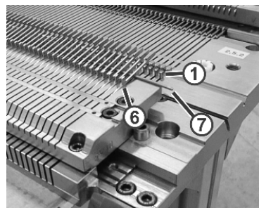
Hochheben der Auswahlplatinen
