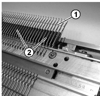
Reinigen des Nadelbetts
