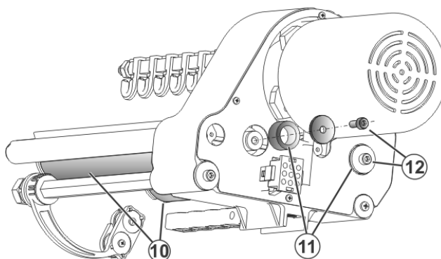
Schrauben für Friktionswalzen
