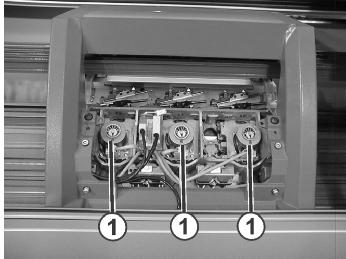
Schrittmotor zur Einstellung der Maschenfestigkeit
