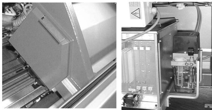
Zentralschmierung am Schlitten, rechts: Ölversorgung
