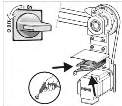
Lüfter Hauptantrieb
