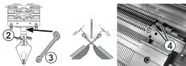
Einstellen der Intarsiafadenführer
