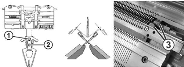
Einstellen der Intarsiafadenführer
