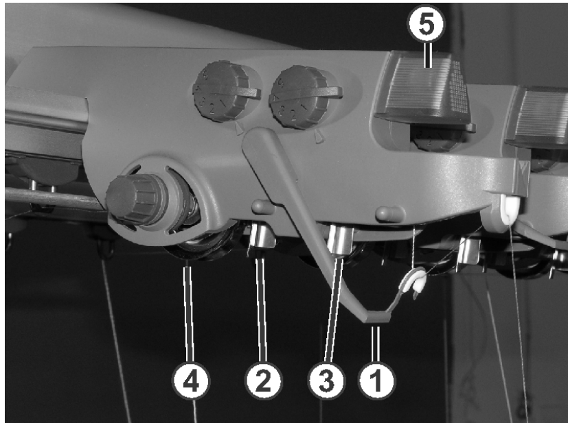
Fadenkontrolleinheit
