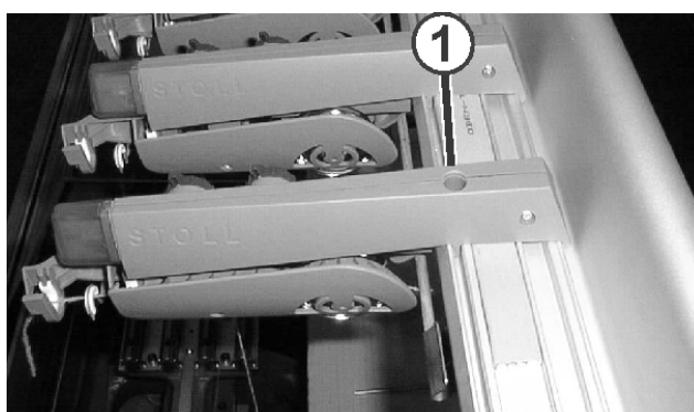
Ausbau einer Fadenkontrolleinheit
