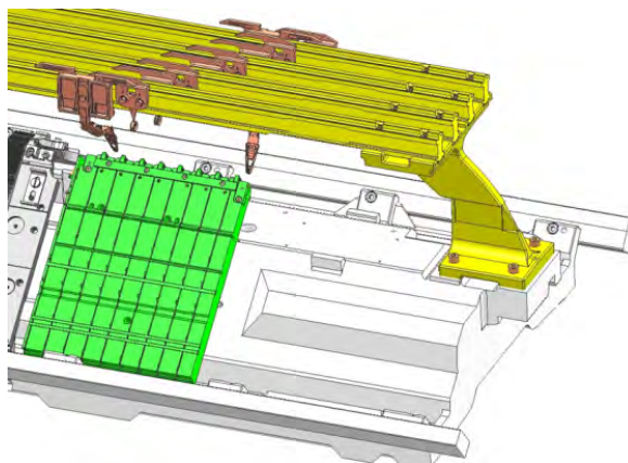
Staffelung der Fadenführerbegrenzer
