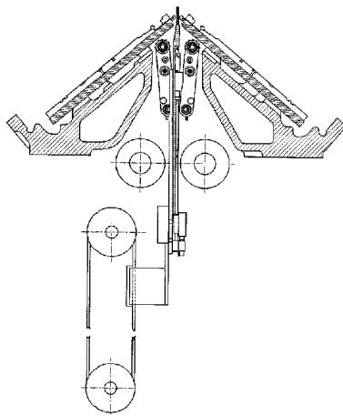
Kammabzug
