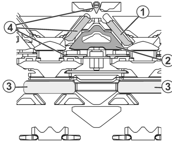
Stricksystem
