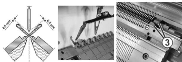
Einstellen der Fadenführer
