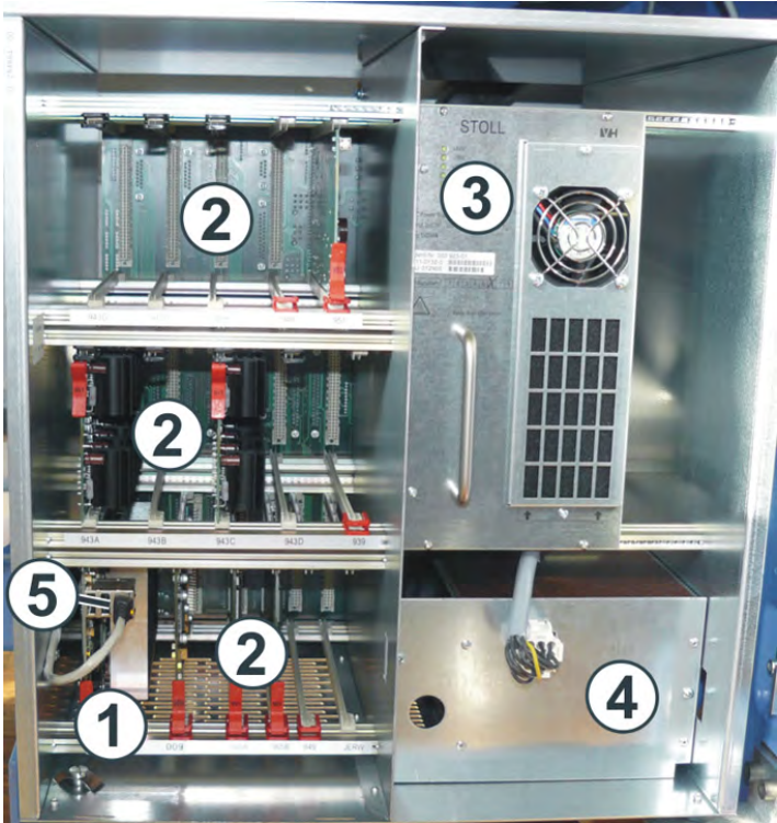
Steuerschrank links
