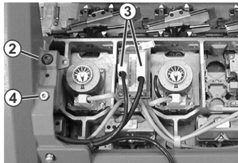
Geöffneter Schlittenwagen
