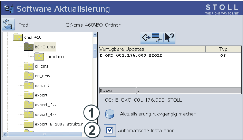
Erweitertes Fenster "Software Aktualisierung"
