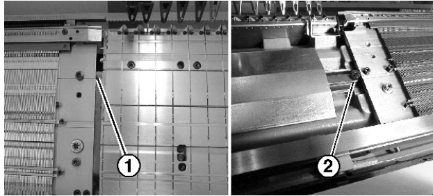
Einbau des vorderen und hinteren Nadelbetts
