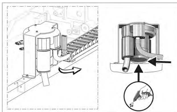
Pulizia della copertura del motore
