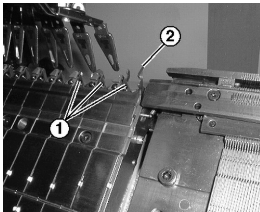
Dispositivo di pinzatura e taglio del filo
