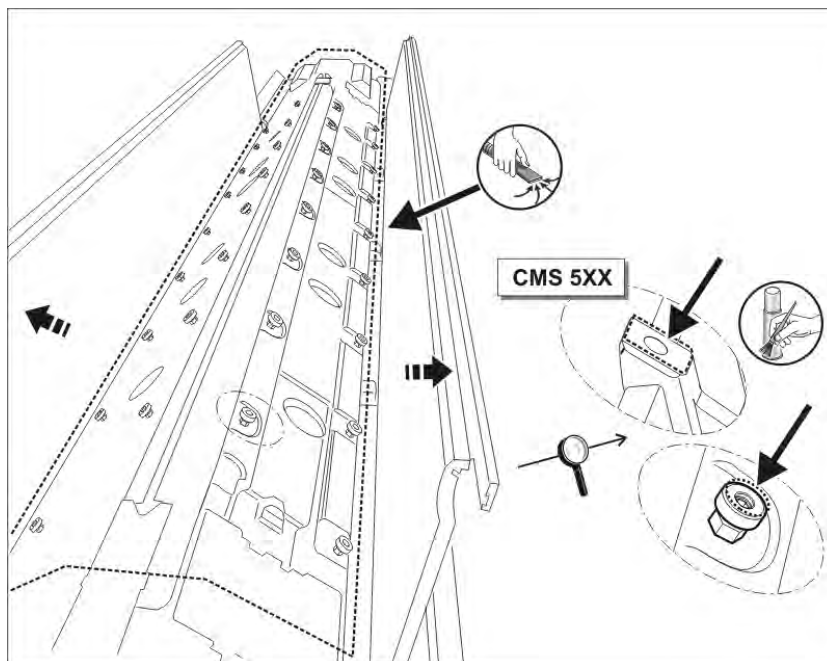
Ingrassaggio degli appoggi della frontura
