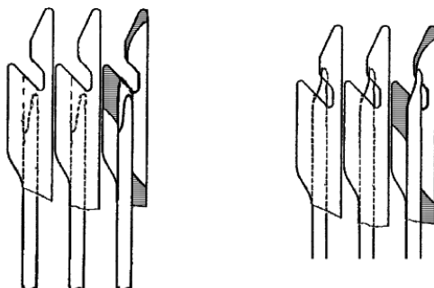
Gancio del pettine del tirapezza con slitte (aperte a sinistra, chiuse a destra)
