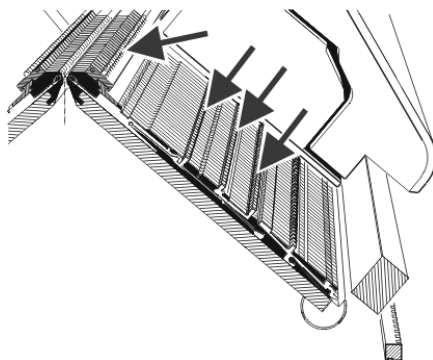
Punti di lubrificazione della lubrificazione centralizzata
