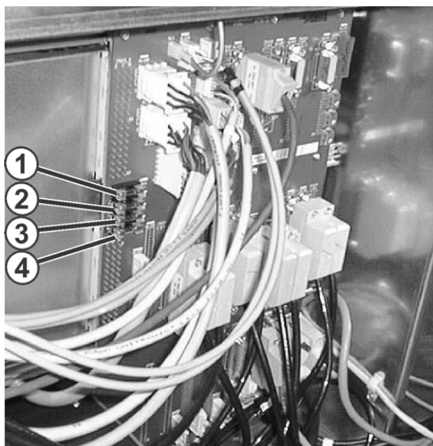
Fusibili sul lato posteriore dell'apparecchio di comando sinistro
