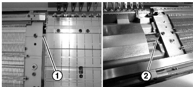
Montaggio delle fronture anteriore e posteriore
