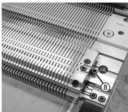
Montaggio della frontura della platina di selezione
