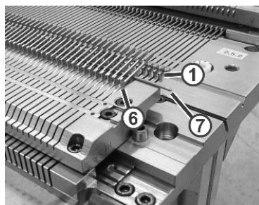
Sollevamento delle platine di selezione
