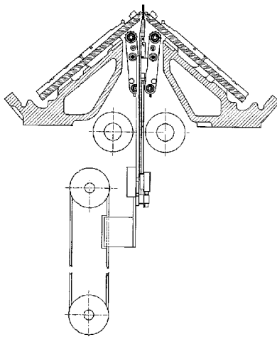
Pettine del tirapezza
