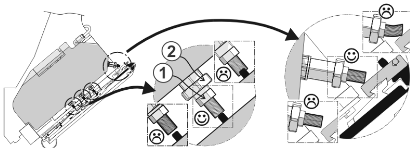
Spazzolini della lubrificazione centralizzata
