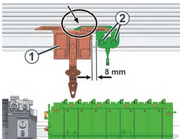
Regolazione dei limitatori dei guidafile
