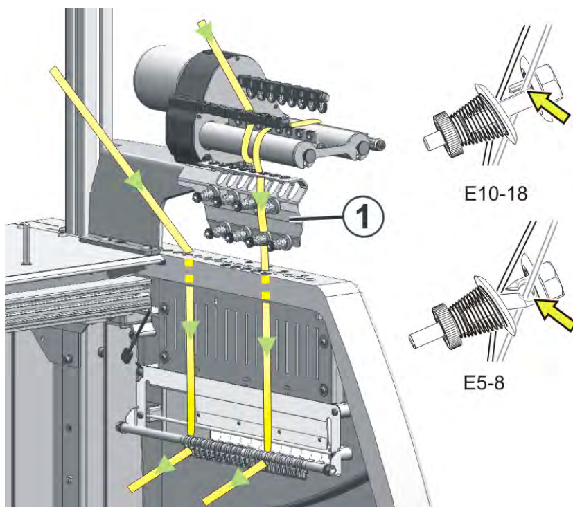
Percorso del filo attraverso il freno permanente
