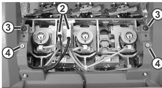
Fissaggio del carro alla slitta
