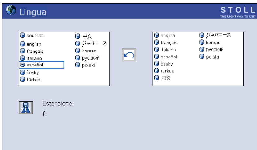
Finestra "Lingua"
