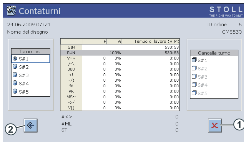
Finestra "Contaturni"
