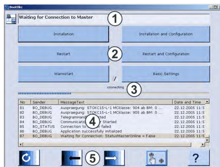
Finestra "BootOkc"
