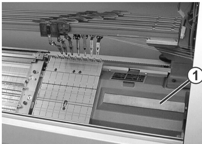
Superficie di appoggio della slitta
