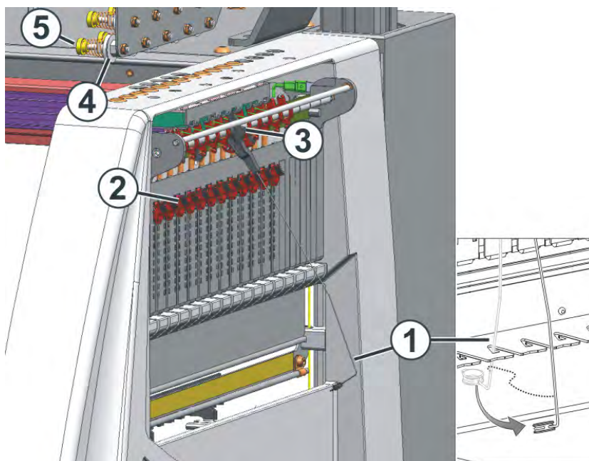
Regolazione della tensione del filo
