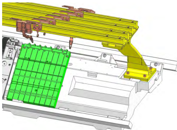
Differenziazione dei limitatori dei guidafile
