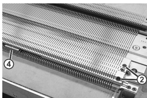
Allentamento della frontura delle platine di selezione
