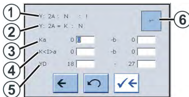
Finestra "Guidafile"
