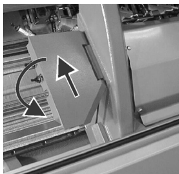
Lubrificazione centralizzata in posizione di lavoro
