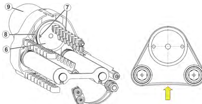
Cinghia di comando
