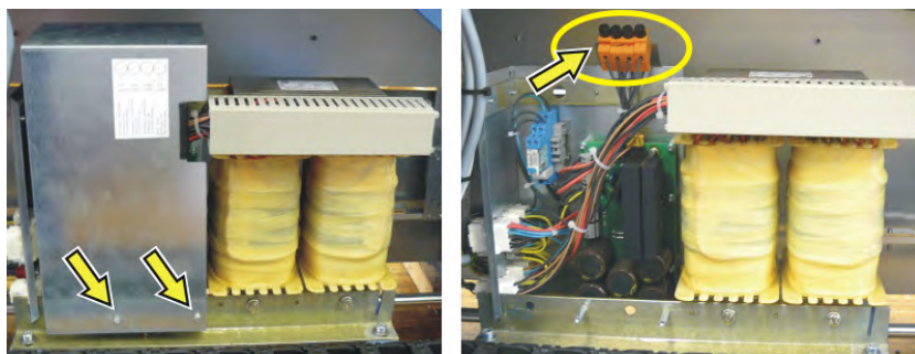
Fusibili del trasformatore sul lato posteriore della macchina
