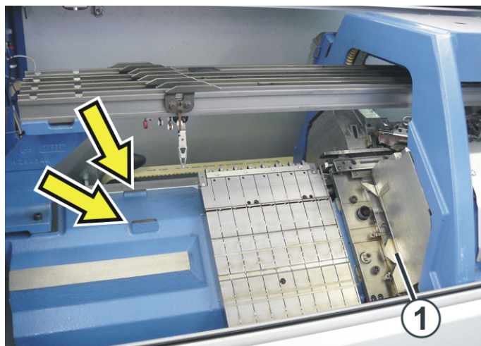
Posição "Carro na frontura" (para melhor vista geral, as coberturas de proteção foram abertas)
