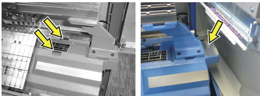
Superfície de apoio para o nível (direita: CMS 502 HP+)
