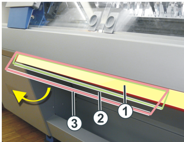
Включващ лост
