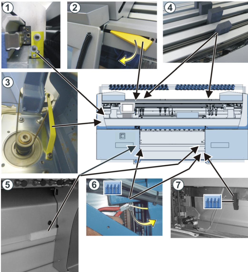
运输固定件的固定点
