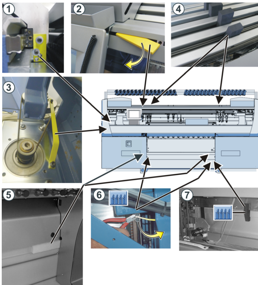
Punti di montaggio delle protezioni per il trasporto
