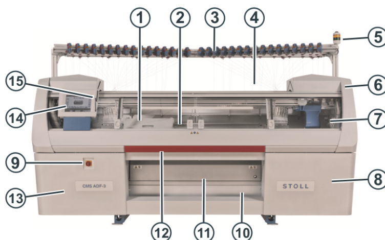
Vista anteriore della macchina per maglieria
