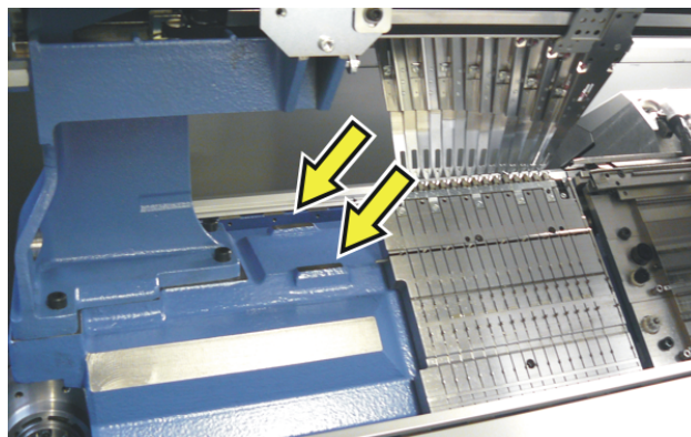
Superficie di appoggio sinistra per la livella
