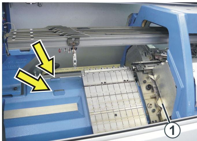
Pozycja "Głowica na łożu igłowym" (dla lepszej orientacji otwarto osłony)
