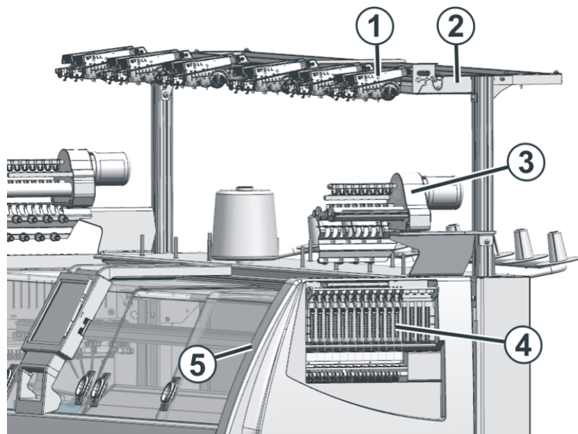
Rechte Seitenansicht
