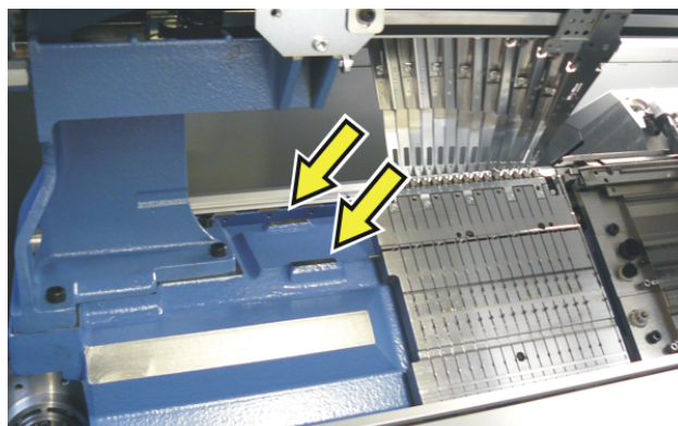
Lewa powierzchnia do ustawienia poziomnicy
