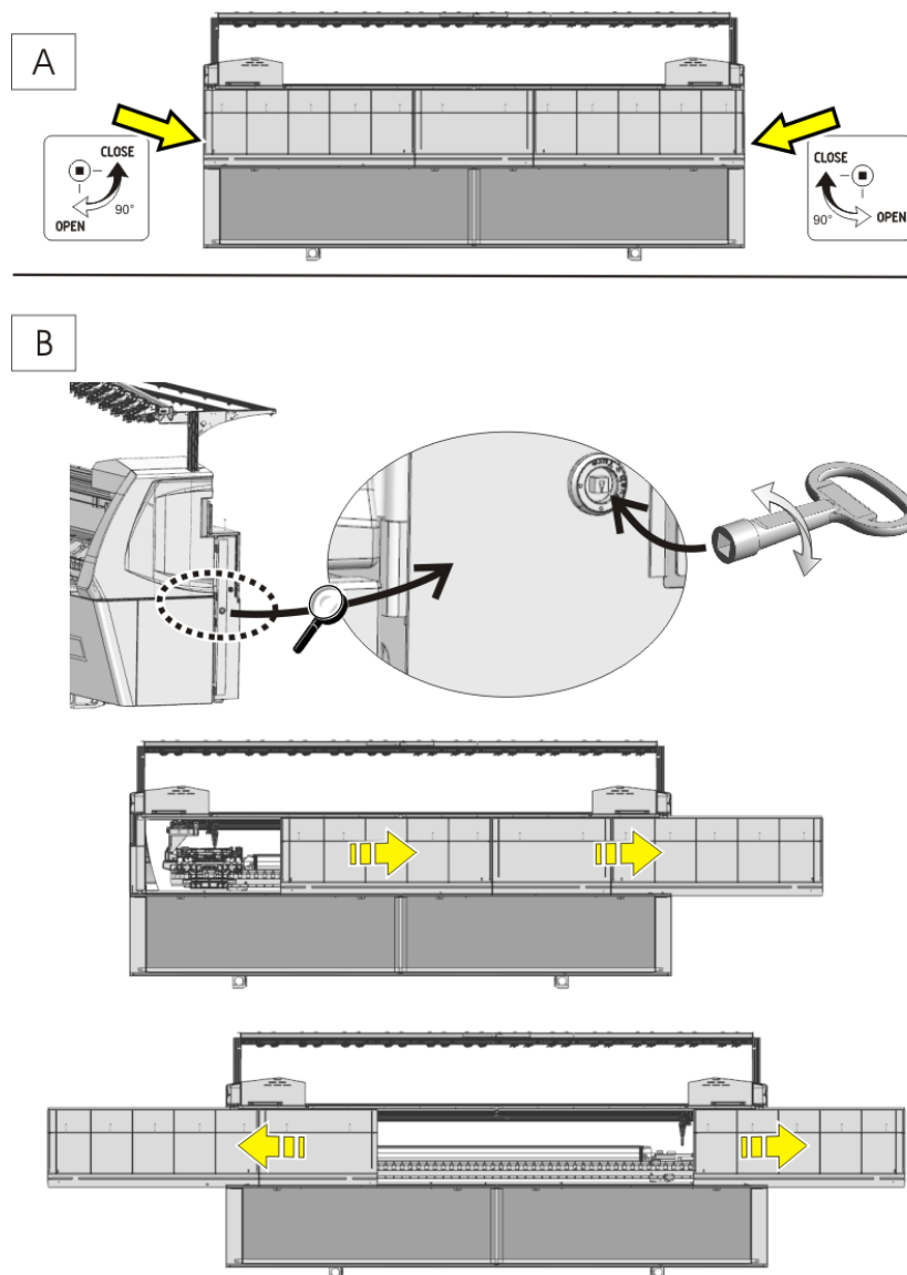
Przesuwna ścianka dla ADF 830
